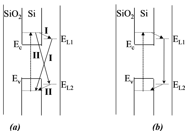
Figure 1.12 – (a) Mécanisme de recombinaison de type II d'après Sacilloti et al. [28]
