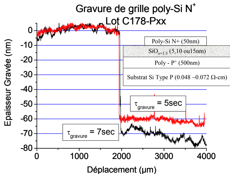
Figure 3.17 – Profondeur de gravure mesurée par profilométrie sur le lot C178-Pxx, le schéma du dispositif finalisé.
