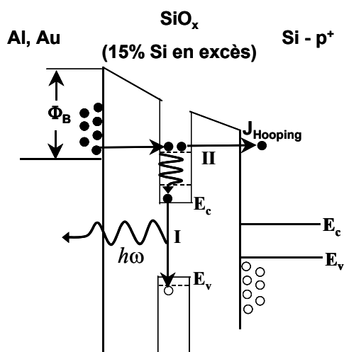
Figure 3.14 – Mécanisme d'injection et d'EL dans les dispositifs du lot O18-xx en accumulation.
