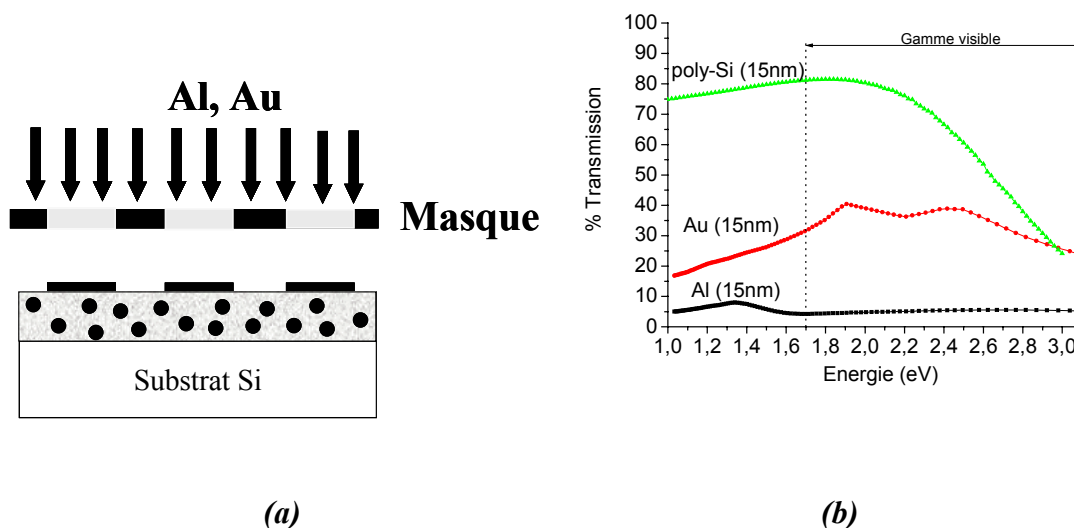
Figure 3.4 – (a) Schéma d'obtention de DELs par évaporation d'une grille métallique (b) Calcul du pourcentage de transmission des grilles d'Al, d'Au et de poly-Si.
