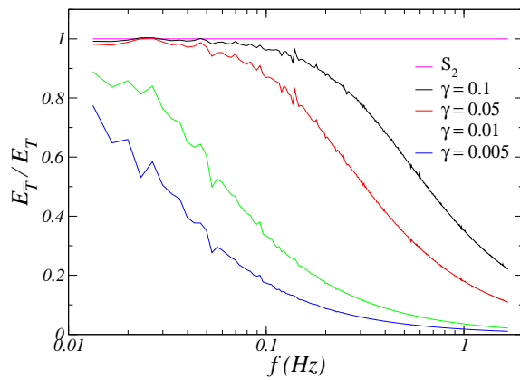
(a) Fonction de transfert appliquée à \tilde{T} issu de S_2 .
