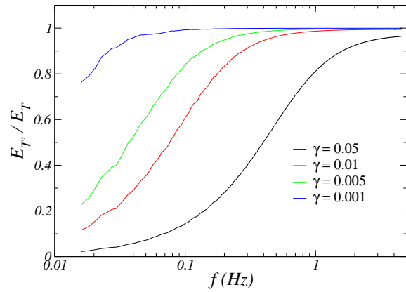
(b) Fonction de transfert appliquée à T' issu de S_1 .
