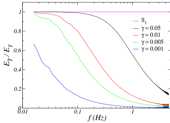
(a) Fonction de transfert appliquée à \tilde{T} issu de S_1 .
