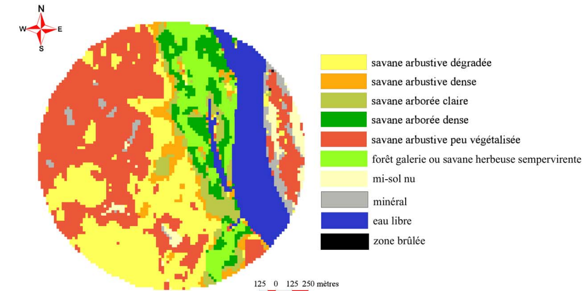
Figure 109. Formations végétales du site de Karé Kopto.
