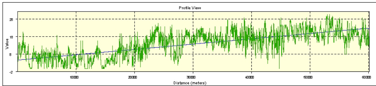
Figure 19. Variation nord-sud de l'indice de végétation dans la partie nord de la zone d'étude.
