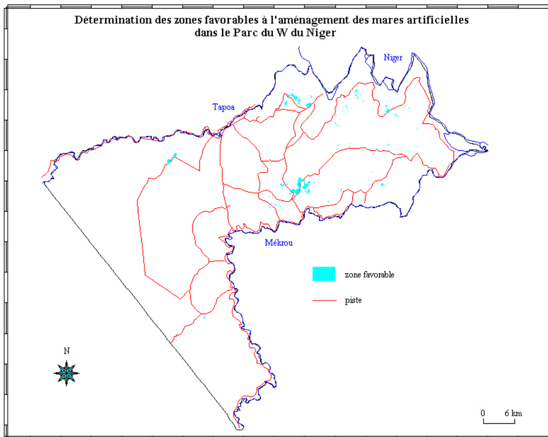
Figure 31. Détermination des zones favorables à l'aménagement des mares artificielles dans le Parc du W du Niger.
