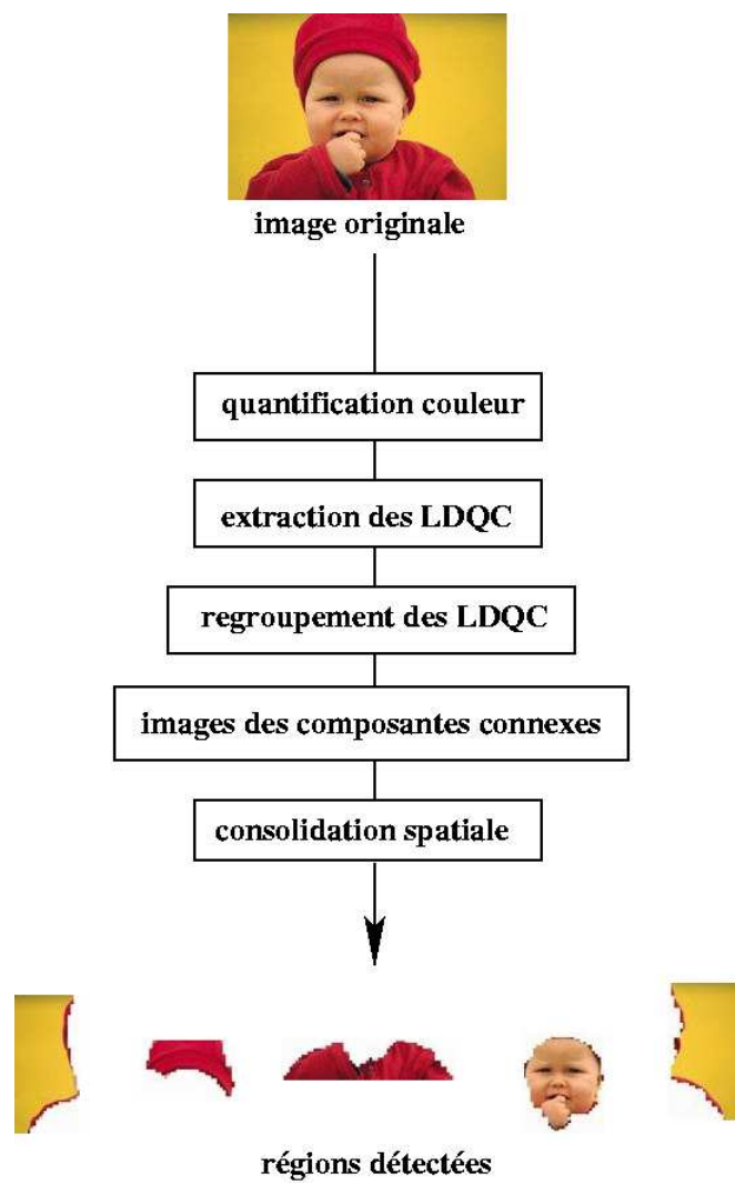
FIG. 3.1 – Résumé du déroulement de la méthode de segmentation.
