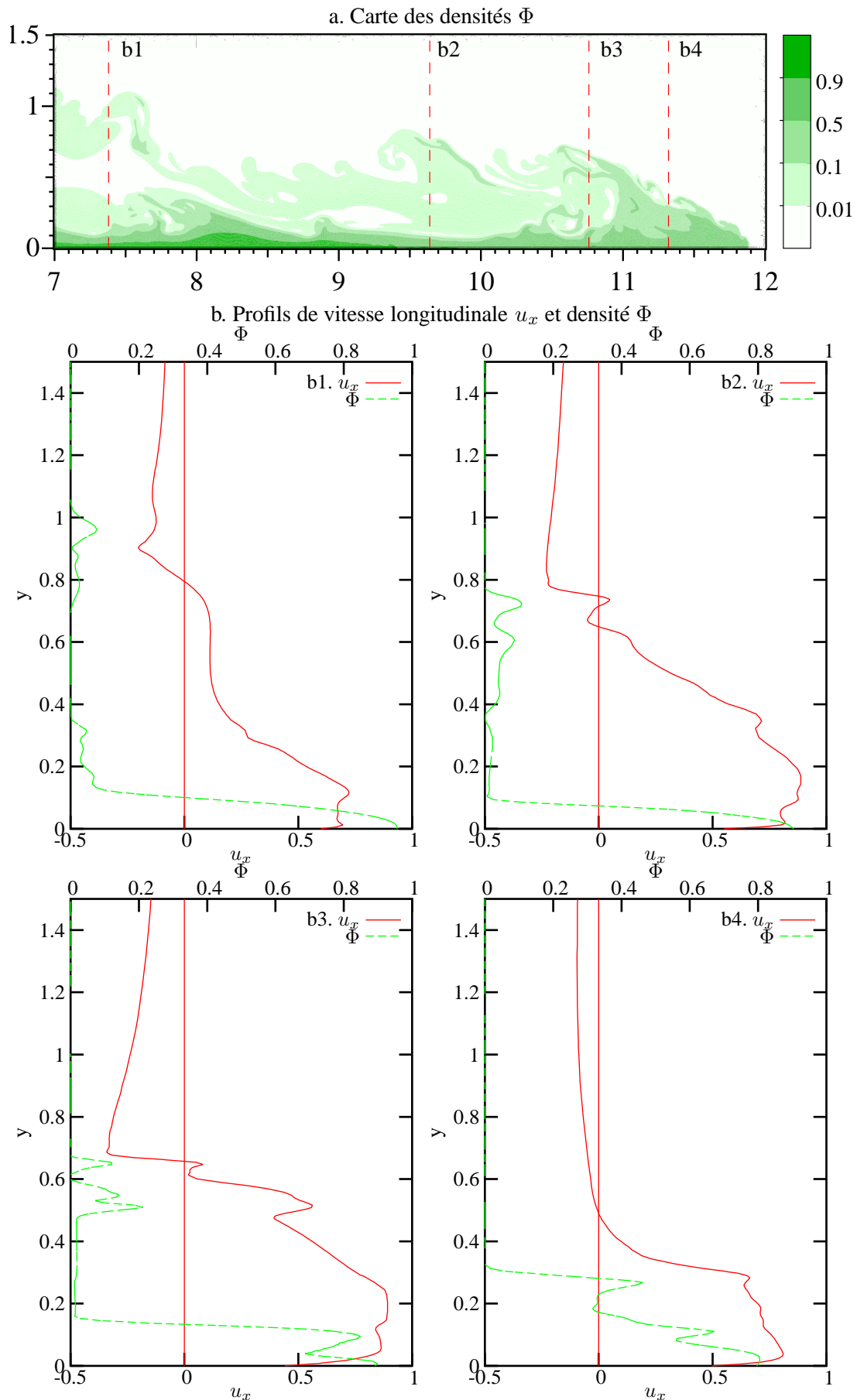
FIG. 54 – Profils de densité dans la tête d'un nuage de forte densité ( N10 ) lorsque le front atteint la position x_f = x_f^*/2 . On a U_f \simeq 0.71 , U_{MC} \simeq 0.59 . Les profils sont tracés sur les lignes de coupe x_f - 4h (b1) et x_f - 2h (b2), x_f - h (b3) et x_f - h/2 (b4).
