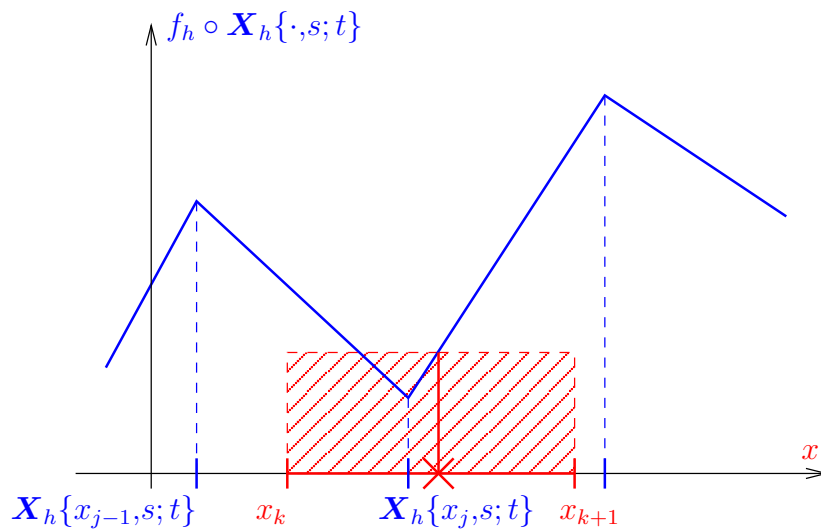
FIG. 7 – Exemple en dimension 1 de l'intégration par une méthode du point central sur l'élément [x_k; x_{k+1}] de la fonction f_h \circ X_h , avec f_h et un champ de vitesse affines par morceaux, et une méthode d'Euler pour calculer X_h . ( f_h \circ X_h est donc affine par morceaux sur un maillage \{X_h(x_1, s; t), \dots, X_h(x_N, s; t)\} ).
