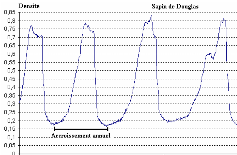
Figure 1.13 : Exemple de profil microdensitométrique obtenu sur un bois adulte de Douglas Fir (données numériques fournies par P. Rozenberg)
