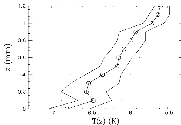
FIG. 4.9 – Profil vertical de la température moyenne (ligne continue et points \circ ), minimale et maximale (lignes continues sans point) en présence d'ondes hydrothermales, pour h=1,2 mm, \Delta T = 15 K et à la position r = 17,5 mm.
