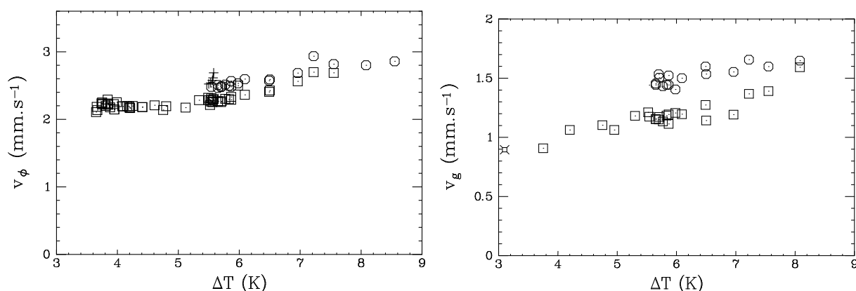
FIG. 3.19 – Evolution de la vitesse de phase v_\phi = k/\omega (à gauche) et de la vitesse de groupe (à droite, mesurée comme vitesse de propagation de perturbations) dans le rectangle en fonction de \Delta T . Les carrés ( \square ) et les ronds ( \circ ) correspondent respectivement au modes 21 et 17. Le premier point du graphe de la vitesse de groupe, pour \Delta T = 3,1 K, correspond à la valeur au seuil dans l'anneau.
