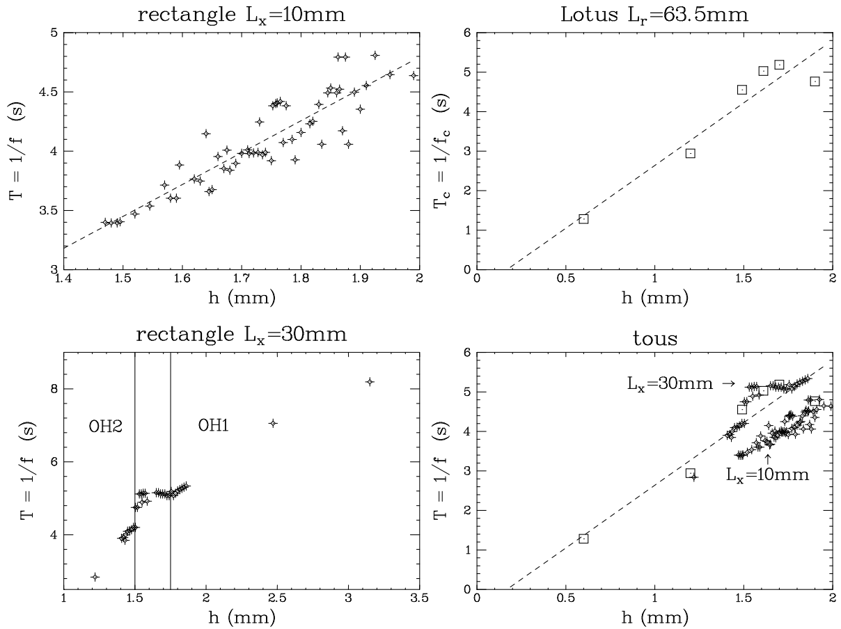
FIG. C.5 – Variation de la période T = f^{-1} avec la hauteur h . A gauche : cas du rectangle pour L_x = 10 \text{ mm} (en haut) et L_x = 30 \text{ mm} (en bas) ; les mesures sont effectuées sur différentes valeurs de \Delta T et la dépendance en \epsilon disperse les points. Pour L_x = 30 \text{ mm} , des OH2 sont observées à petite hauteur et il existe une plage (en h ) de transition entre les deux types d'ondes. A droite : cas du disque (en haut) ; seules les valeurs au seuil de l'instabilité en onde sont reportées. La compilation des résultats (en bas à droite) montre la dépendance vis-à-vis de L_{\parallel} : le confinement augmente la fréquence. Un saut de fréquence distingue les deux types d'ondes hydrothermales.
