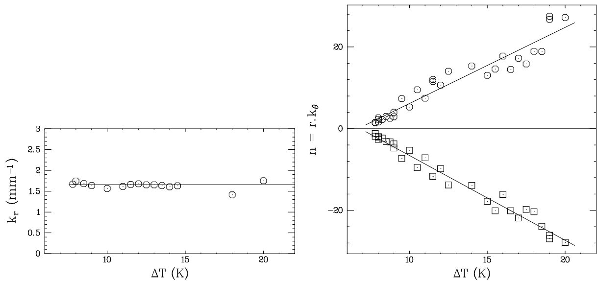
FIG. 5.28 – Evolution du vecteur d'onde des OH2 pour h = 1, 2 mm et \Delta T > 0 . A gauche : k_r ; à droite : k_\theta .
