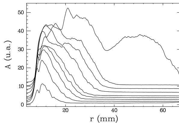
FIG. 5.29 – Empilement de profils radiaux d'amplitude locale pour h = 1, 2 mm et différents \Delta T > 0 : 8, 9, 10, 11, 12, 14, 16, 18 et 20 K. Pour des raisons de clarté, les profils ont été décalés dans la direction verticale d'un facteur proportionnel à \Delta T . Sur le dernier profil ( \Delta T = 20 K), les OH1 sont présentes et l'amplitude est finie partout dans la cellule.
