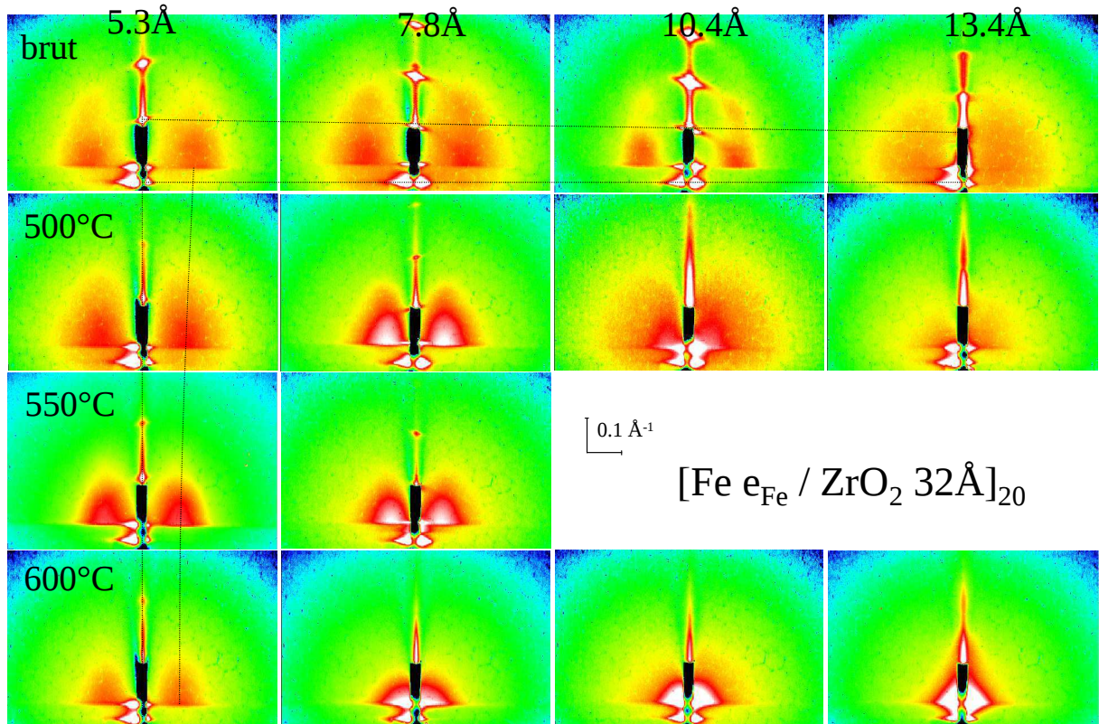
FIG. 4.16 – Figures GISAXS mesurées sur les multicouches [\text{Fe } e_{\text{Fe}} / \text{ZrO}_2 \text{ } 32\text{\AA}]_{20} en fonction de l'épaisseur de fer déposée, e_{\text{Fe}} = 5.3, 7.8, 10.4 et 13.4\text{\AA} , et de la température de recuit T_R = 500, 550 et 600^\circ\text{C} . Le trait horizontal (resp. vertical) indique la position de l'axe q_{//} (resp. q_z ). Les lignes incurvées passent par les pics de Bragg et les pics de corrélations selon q_{//} .
