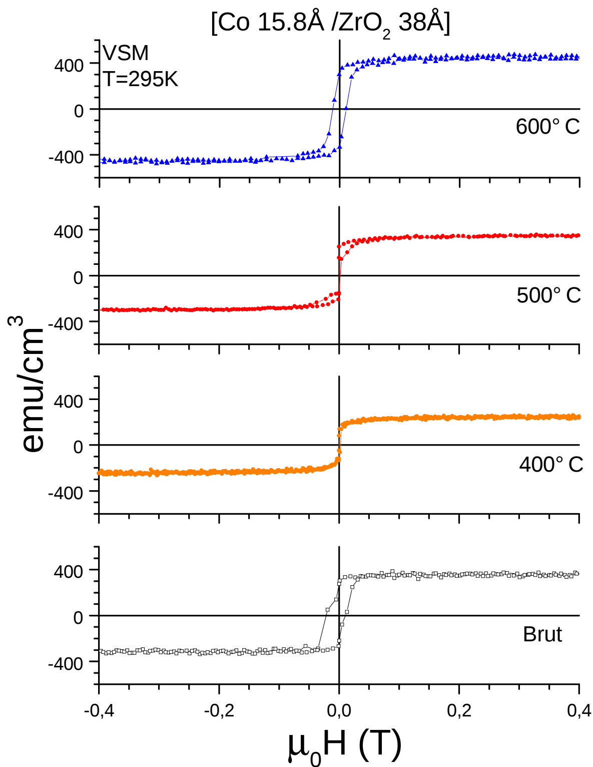
FIG. 6.12 – Cycles d'aimantation des multicouches [\text{Co } 15.8\text{\AA} / \text{ZrO}_2 \text{ } 38\text{\AA}]_{40} brute de dépôt et recuites à 500, 550 et 600° C, mesurés au VSM à 295K.
