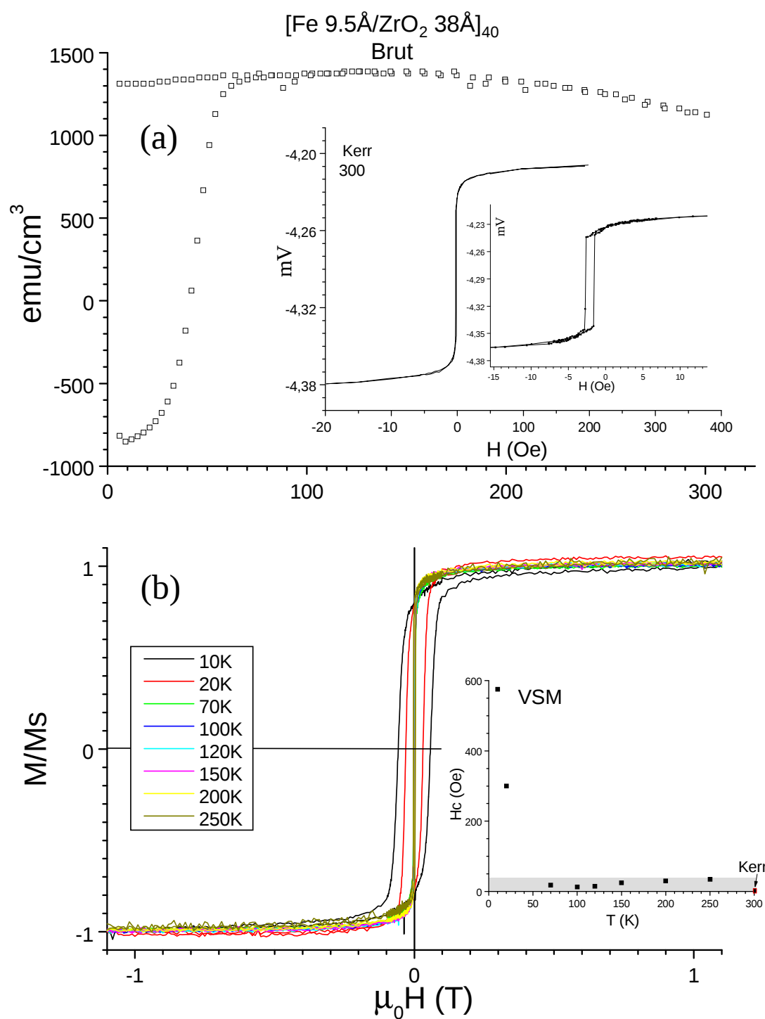
FIG. 6.2 – Comportement magnétique de la multicouche [\text{Fe } 9.5\text{\AA} / \text{ZrO}_2 \text{ } 38\text{\AA}]_{40} brute de dépôt : (a) Courbe ZFC-FC avec H=100\text{Oe} . En insertion, cycle d'aimantation mesuré par effet Kerr à 300\text{K} , avec un agrandissement du cycle à faible champ : H_C \sim 10\text{Oe} . Le décalage est dû à la rémanence des bobines de champ. (b) Cycles mesurés au VSM à plusieurs températures. En insertion, valeurs du champ coercitif mesurées en fonction de la température de mesure au VSM et par effet Kerr à 300\text{K} .
