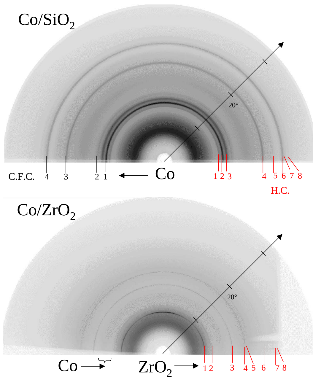
FIG. 5.3 – Diffraction X aux grands angles en incidence rasante sur [Co 15.3Å/SiO 2 43Å] (haut) et [Co 10.7Å/ZrO 2 38Å] (bas) recuits à 600°C effectuée sur ID09 par F. d’Acapito. \lambda=0.46\text{\AA} . Les chiffres repères pour l’élément métallique et la matrice les raies suivantes dans l’ordre : Co (H.C.) : (100), (002), (101), (110), (103), (200), (112) et (201) ; Co (C.F.C.) : (111), (200), (220) et (311). ZrO 2 cubique : (111), (200), (220), (311), (222), (400), (331), (420).
