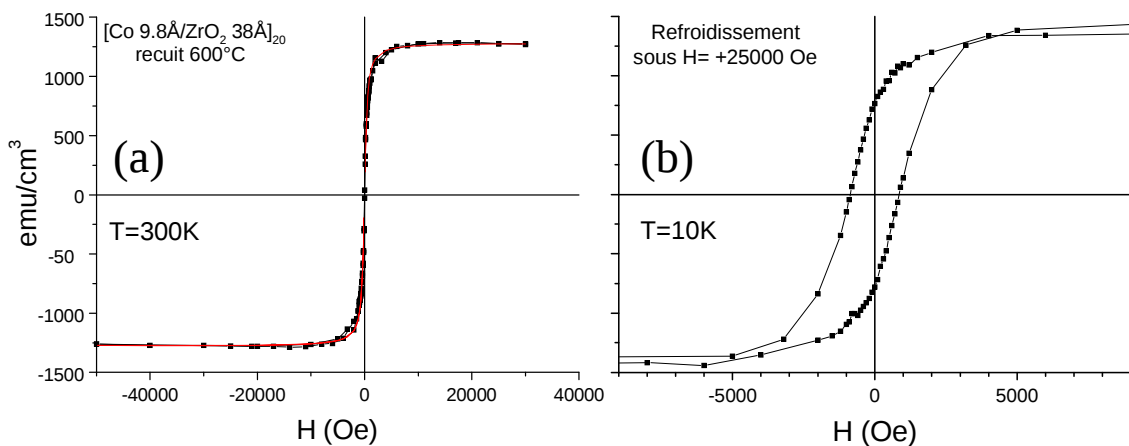
FIG. 6.10 – Magnétisme de la multicouche [\text{Co } 9.8 \text{ \AA} / \text{ZrO}_2 \text{ } 38 \text{ \AA}]_{20} recuite à 600^\circ\text{C} . (a) Cycle d'aimantation mesuré à 300K. (b) Cycle d'aimantation mesuré à 10K après un refroidissement à partir de 300K sous un champ H = + 25000 Oe.
