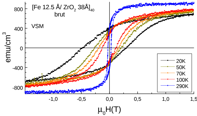
FIG. 6.5 – Cycles d'aimantation mesurés au VSM sur la multicouche [\text{Fe } 12.5\text{\AA} / \text{ZrO}_2 \text{ } 38\text{\AA}]_{40} brute de dépôt à plusieurs températures.
