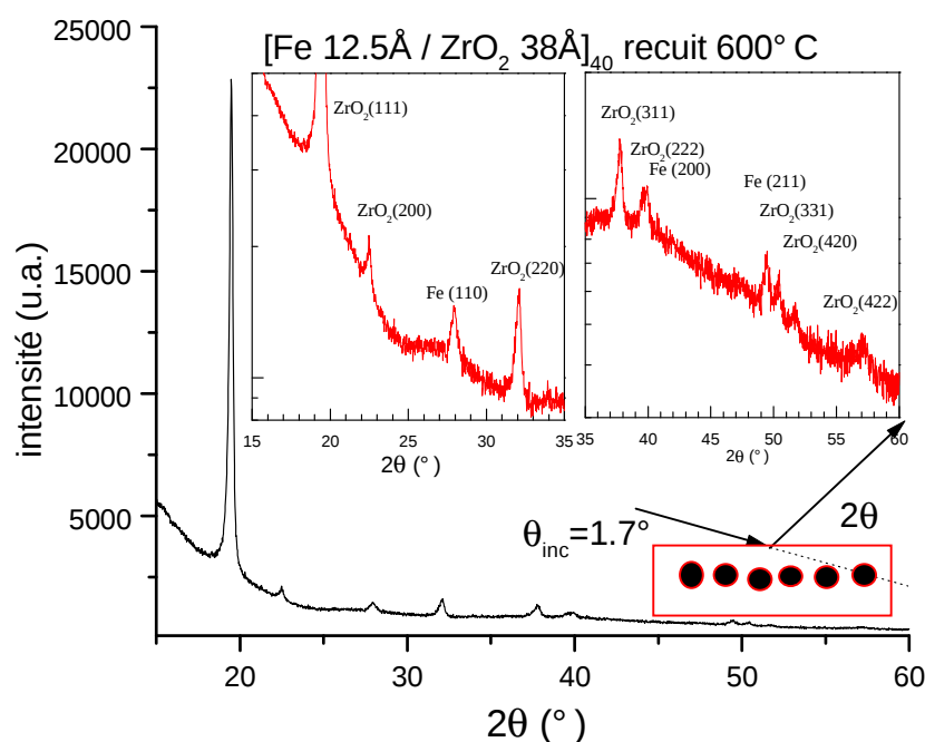
FIG. 5.1 – Diffraction X aux grands angles en incidence rasante sur une multicouche [Fe 12.5Å / ZrO 2 38Å] 40 recuite à 600°C. Le spectre a été réalisé sur BM32 à l'aide d'un détecteur ponctuel (NaI) sous une incidence de 1.7° et pour \lambda = 0.98 \text{ \AA} .
