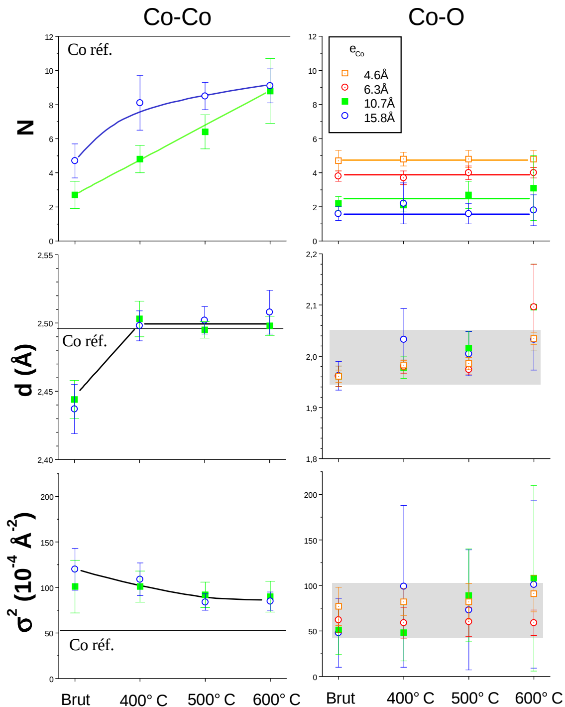
FIG. 5.14 – Valeurs des paramètres structuraux ( N , nombre de voisins, d , première distance, et \sigma^2 , facteur de Debye-Waller) issus des ajustements des spectres des multicouches [\text{Co } e_{Co}/\text{ZrO}_2 \text{ 38 Å}]_{20} brutes de dépôt, recuites à 400 et 600°C en fonction de l'épaisseur de cobalt, e_{Co} , pour la couche de voisins atomiques cobalt (colonne de gauche) et oxygène (colonne de droite). Les valeurs obtenues des facteurs E_0 ne sont pas représentées : elles varient relativement peu d'un échantillon à l'autre. Le facteur de qualité r est plus important pour les multicouches de faibles épaisseurs ( e_{Co}=4.6 et 6.3 \text{ Å} ) et celles à l'état brut de dépôt ou recuites à 400°C.
