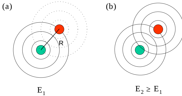
FIG. 3.7 – Exemple de rétrodiffusion (sans déphasage) de l'onde associée au photoélectron par un voisin à une distance R de l'atome absorbeur. (a) Maximum de probabilité d'absorption pour E_1 , quand le maximum d'amplitude de l'onde rétrodiffusée se situe au centre de l'atome absorbeur. (b) Diminution de la probabilité d'absorption pour une énergie des photons incidents légèrement supérieure à E_1 . On obtient des maxima de probabilité quand 2(\frac{2\pi}{\lambda})R est un multiple de 2\pi . L'oscillation de la section efficace d'absorption est donc \pi/R périodique en fonction de k .
