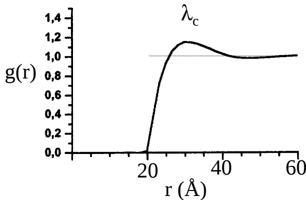
FIG. 3.15 – Fonction de corrélation radiale g(r) typique des centres de particules de rayon 20Å (d'après [Vass 00]). g(r) est nulle jusqu'à 20Å en raison de l'impossibilité d'interpénétration des particules (modèle des sphères dures). Elle présente un maximum en \lambda_c et tend de manière oscillante vers 1 pour les grandes valeurs de r .
