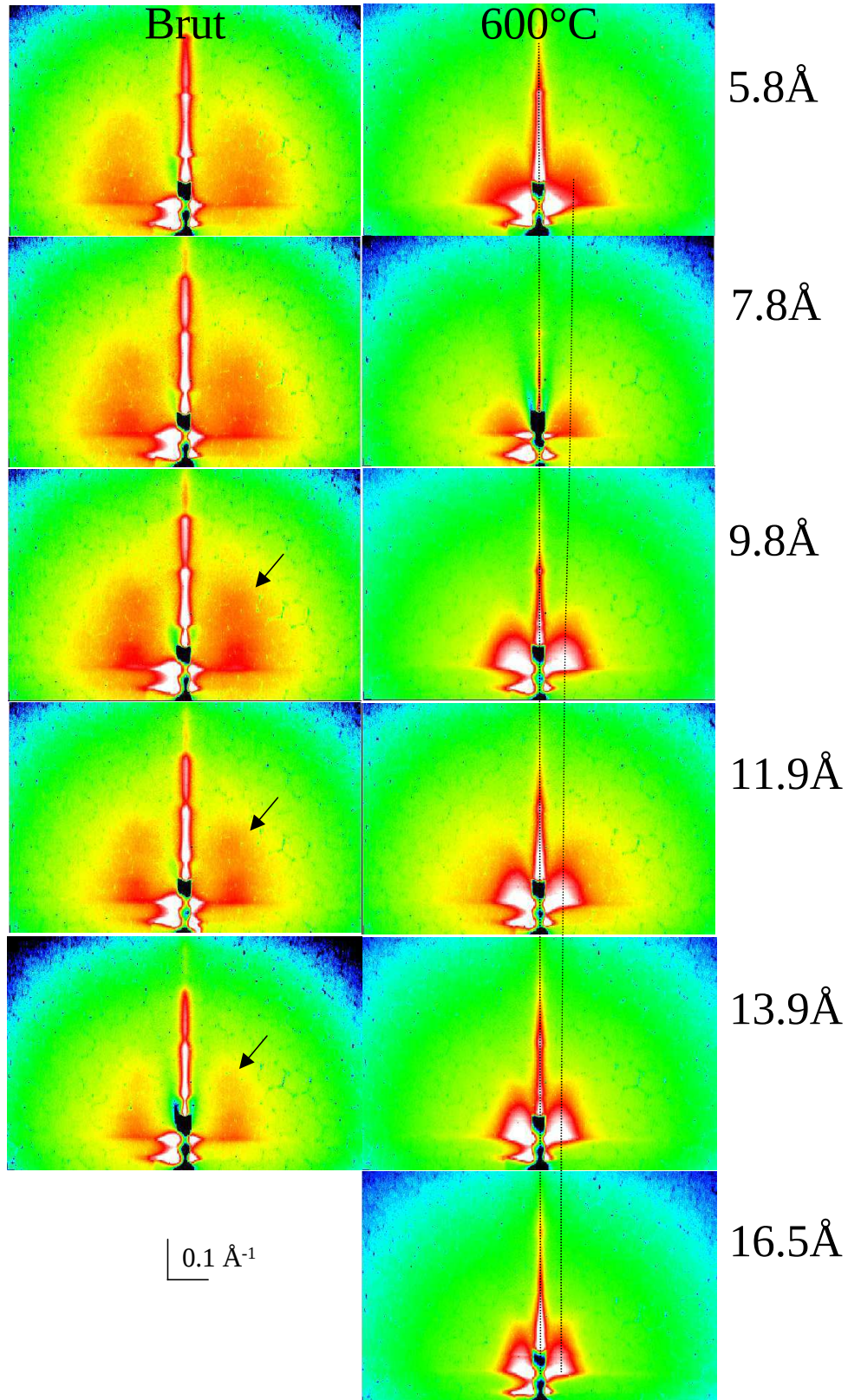
FIG. 4.17 – Figures GISAXS mesurées sur les multicouches [\text{Co } e_{\text{Co}}/\text{ZrO}_2 \text{ } 38\text{\AA}]\text{ }_{20} à l'état brut de dépôt ou recuites à 600^\circ\text{C} en fonction de l'épaisseur de cobalt déposée, e_{\text{Co}}=5.8, 7.8, 9.8, 11.9, 13.9 et 16.5\text{\AA} . Le trait vertical indique la position de l'axe q_z . La ligne incurvée passe par les pics de corrélations selon q_{//} . Les flèches signalent la présence d'un maximum local de l'intensité diffusée en dehors des axes q_z et q_{//} .
