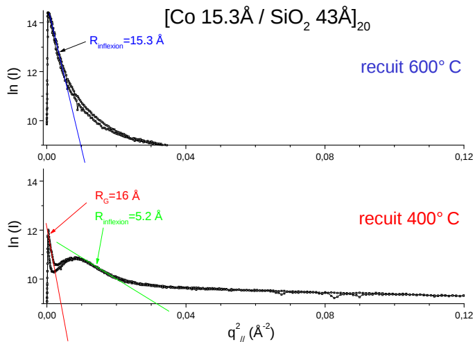
FIG. 4.31 – Coupes d'intensité diffusée dans la direction q_{//} à la hauteur de l'horizon Yoneda pour les multicouches [Co\ 15.3\text{\AA} / SiO_2\ 43\text{\AA}]_{20} recuites à 400 et 600°C. L'intensité est tracée selon la méthode de Guinier, \ln(I(q)) en fonction de q^2 . La pente à l'origine de l'intensité dans ce tracé donne le rayon de giration des particules, R_G : p(0)=R_G^2/3 . Par analogie en l'absence de pente à l'origine, on peut extraire un rayon de giration au point d'inflexion de la courbe d'intensité : p(\text{inflexion})=R_{inflexion}^2/3 . Le rayon des particules sphériques est supérieur de 30% au rayon de giration mesuré : R=\sqrt{5/3}R_G .
