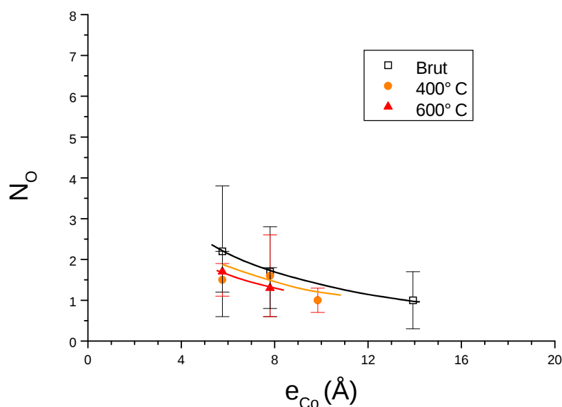
FIG. 5.16 – Valeurs du nombre de voisins atomiques O, N_O , en fonction de l'épaisseur de cobalt e_{Co} pour des multicouches [Co\ e_{Co}/ZrO_2\ 38\text{\AA}]_{20} brutes de dépôt, recuites à 400 et 600°C. Malgré la pondération en k du signal EXAFS avantageuse pour la contribution Co-O, l'environnement local des atomes de cobalt contient peu d'atomes d'oxygène.
