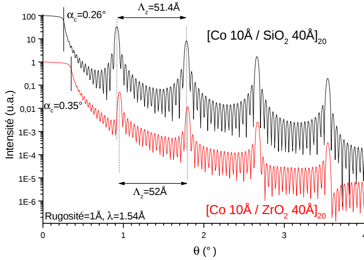
FIG. 4.3 – Simulation de l'intensité réfléchie par des multicouches de [\text{Co } 10\text{\AA} / \text{SiO}_2 \text{ } 40\text{\AA}]_{20} et [\text{Co } 10\text{\AA} / \text{ZrO}_2 \text{ } 40\text{\AA}]_{20} à la longueur d'onde \lambda=1.54\text{\AA} . La rugosité a été fixée à 1\text{\AA} . Les valeurs de la table (4.1) ont été utilisées dans le calcul par le serveur [CRXO]. L'estimation de la période de la bicouche conduit à une valeur supérieure de quelques \text{\AA} à celle attendue. Les valeurs des angles critiques déduits des courbes sont en très bon accord avec ceux obtenus à partir de la formule (3.32). En raison du contraste électronique, l'intensité réfléchie de \text{Co/SiO}_2 est supérieure à celle de \text{Co/ZrO}_2 d'un facteur compris entre 5 et 7 selon les épaisseurs étudiées dans cette thèse.
