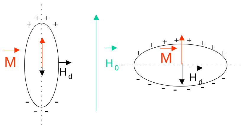
FIG. 2.7 – Formation de pôles magnétiques et intensité du champ démagnétisant en fonction de la direction d'application du champ \vec{H}_0 selon les axes principaux d'une ellipsoïde de révolution.
