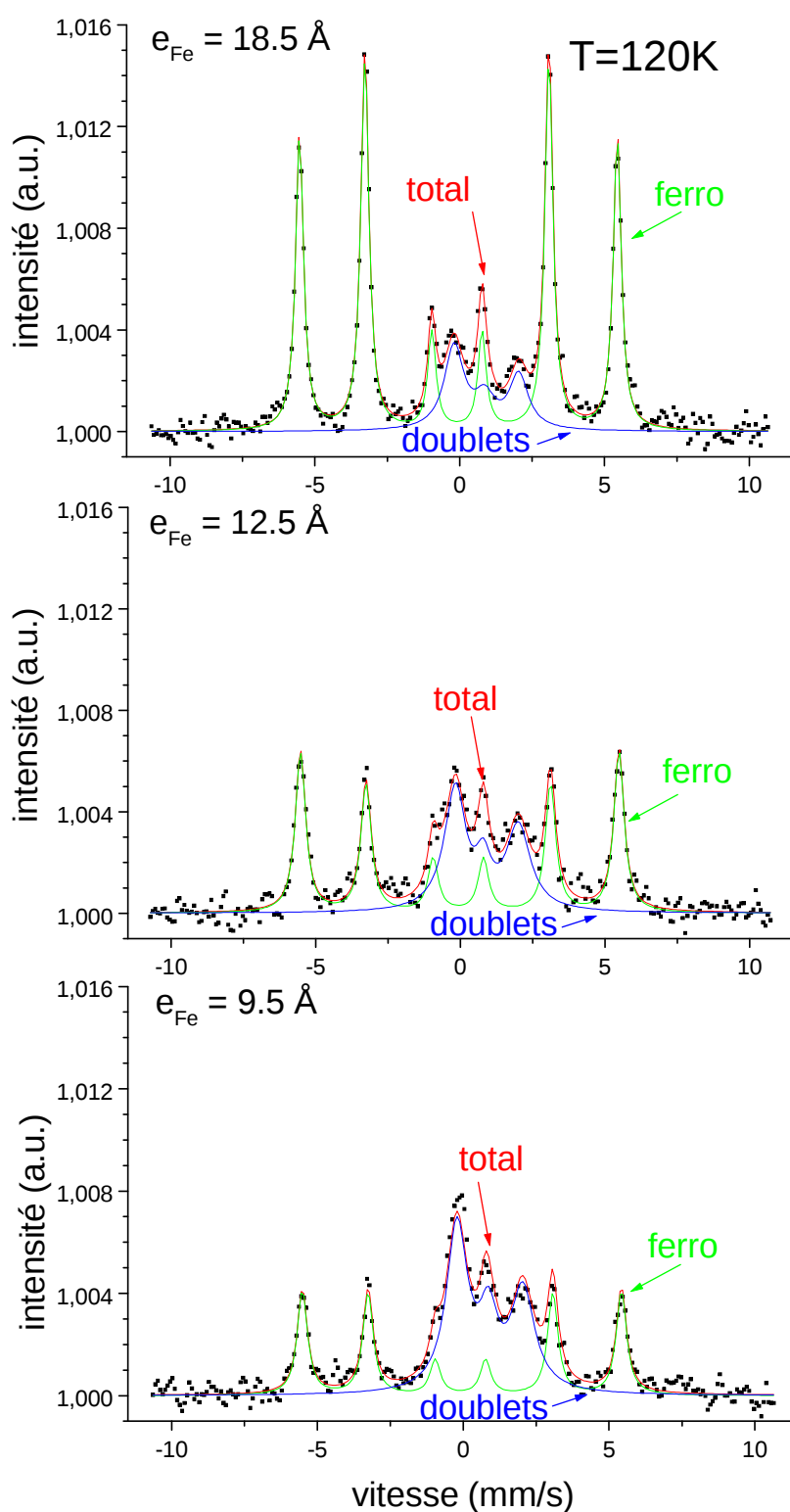
FIG. 5.29 – Spectres Mössbauer mesurés à 120K de multicouches [Fe\ e_{Fe}/ZrO_2\ 38\text{\AA}]_{40} recuites à 600^\circ\text{C} pour trois épaisseurs e_{Fe}=9.5, 12.5 et 18.5\text{ \AA} . L'intensité du signal des doublets attribués aux ions Fe^{2+} et Fe^{3+} décroît à mesure que e_{Fe} augmente.
