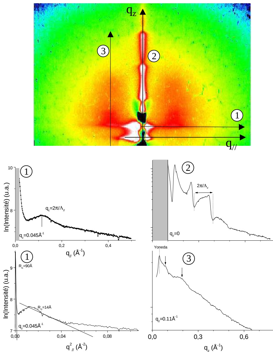
FIG. 4.19 – Figure GISAXS de la multicouche [\text{Co } 9.8\text{\AA}/\text{ZrO}_2 \text{ } 38\text{\AA}]_{20} brute de dépôt. Les variations de l'intensité diffusée selon les directions de coupe indiquées sont données dans les graphiques du bas. (1) coupe // au niveau de l'horizon, (2) coupe dans le plan d'incidence à q_{//}=0 , (3) coupe selon q_z au niveau du maximum d'intensité en q_{//} . Les régions masquées par les puits sont signalées en gris.
