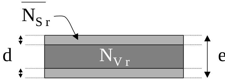
FIG. 6.31 – Calcul du nombre moyen de voisins réduit pour une couche continue (dimension infinie dans le plan). On attribue aux deux couches superficielles d'épaisseurs d , un nombre moyen de voisins réduit de surface N_{Sr} .
