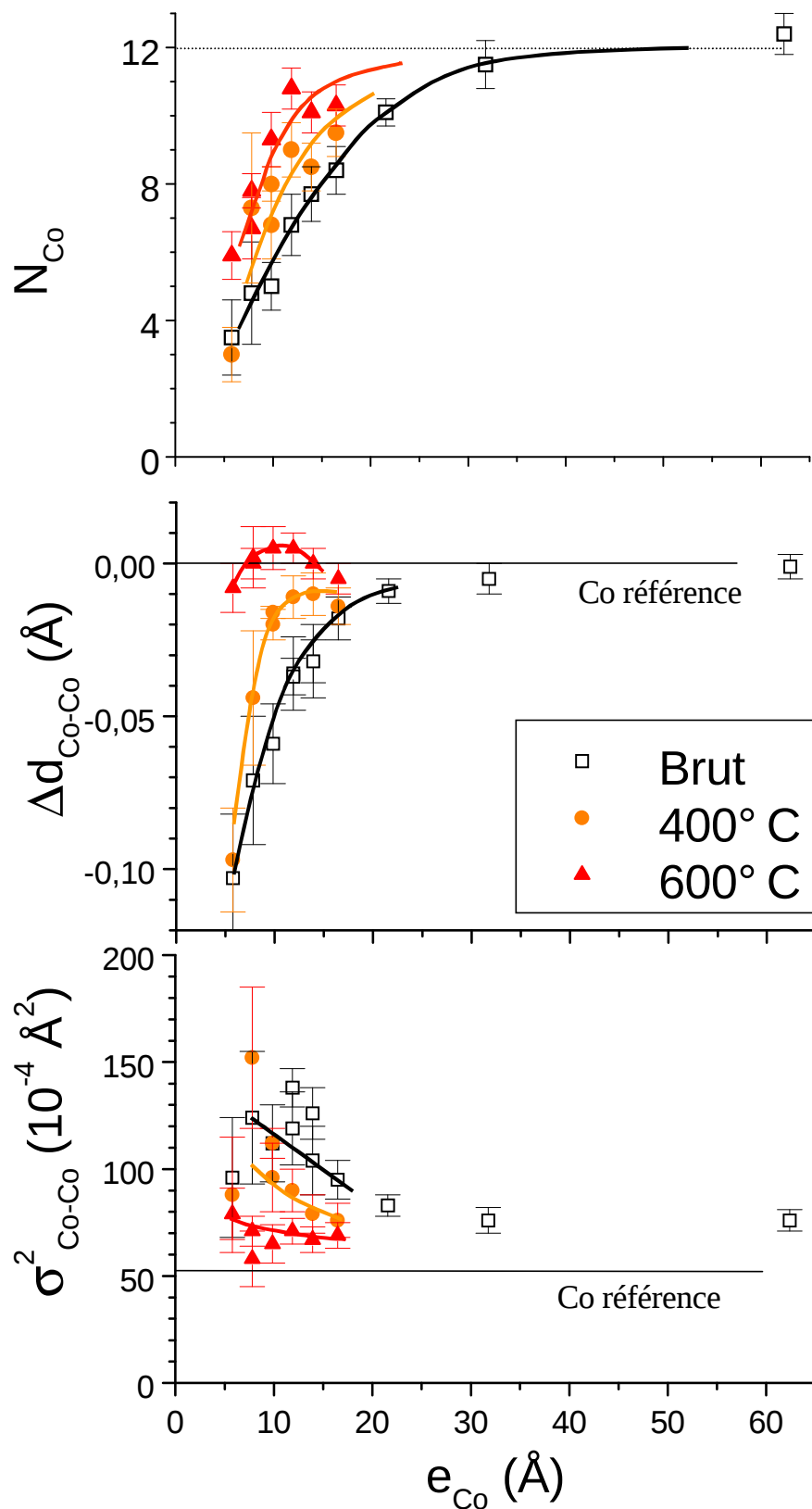
FIG. 5.17 – Valeurs du nombre de voisins atomiques Co, N_{Co} , de l'écart de la première distance atomique entre voisins cobalt à la distance mesurée dans le cobalt massif ( 2.497\text{Å} ), \Delta d_{Co-Co} , et du désordre de la première couche de voisins cobalt \sigma^2_{Co-Co} , en fonction de l'épaisseur de cobalt e_{Co} pour des multicouches [\text{Co } e_{Co}/\text{ZrO}_2 \text{ } 38\text{Å}]_{20} brutes de dépôt, recuites à 400 et 600°C. Les spectres ont été mesurés à 300K en CEY en mode de détection de fluorescence. Pour les ajustements, les signaux EXAFS ont été multipliés par k . L'erreur statistique est indiquée par une barre d'erreur. Les lignes tracées sont des guides pour les yeux.
