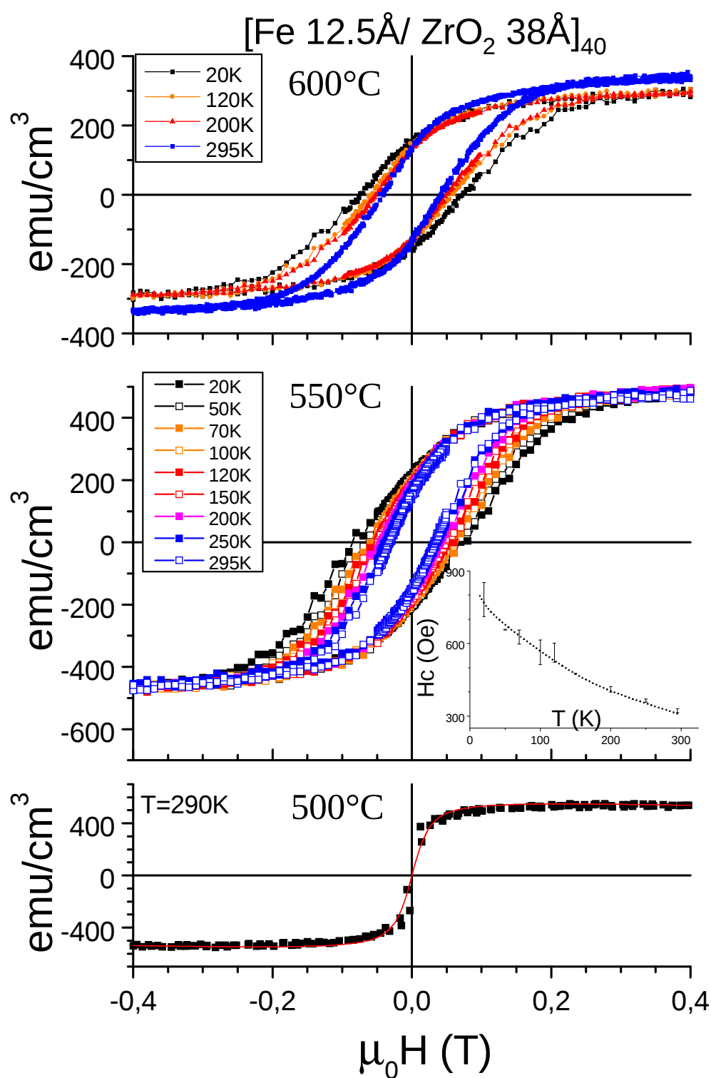
FIG. 6.6 – Cycles d'aimantation mesurés à plusieurs températures au VSM sur les multicouches [\text{Fe } 12.5\text{\AA} / \text{ZrO}_2 \text{ } 38\text{\AA}]_{40} recuites à 500, 550 et 600°C. En insertion, variation du champ coercitif de la multicouche recuite à 550°C avec la température.
