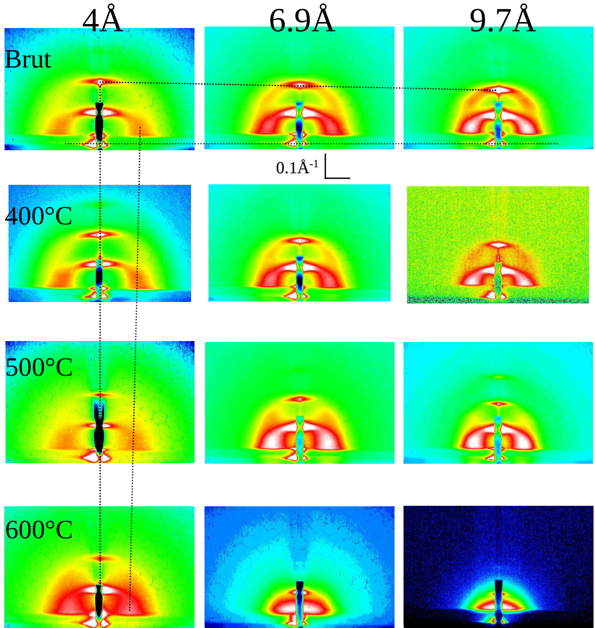
FIG. 4.22 – Clichés de diffusion GISAXS des multicouches [\text{Co } e_{\text{Co}} / \text{SiO}_2 \text{ } 43.2 \text{ \AA} ]_{20} pour trois épaisseurs de cobalt déposé e_{\text{Co}} = 4, 6.9 et 9.7 \text{ \AA} en fonction du recuit thermique (brut de dépôt, recuit à 400, 500 et 600^\circ\text{C} ). L'échelle angulaire est commune à tous les clichés qui ont été alignés verticalement selon q_{\parallel}=0 , et horizontalement selon la hauteur du faisceau direct. L'échantillon e_{\text{Co}}=9.7 \text{ \AA} recuit à 400^\circ\text{C} a été mesuré avec un temps de comptage inférieur à celui des autres échantillons. L'échelle des intensités est logarithmique.
