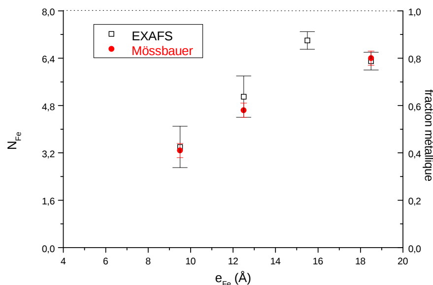
FIG. 6.26 – Comparaison des valeurs de la fraction métallique dans les multicouches [Fe\ e_{Fe}/ZrO_2] , mesurée à partir de l'intensité des composantes ferro- et superparamagnétique des spectres Mössbauer et du nombre de premiers voisins atomiques fer issus des ajustements des spectres EXAFS.
