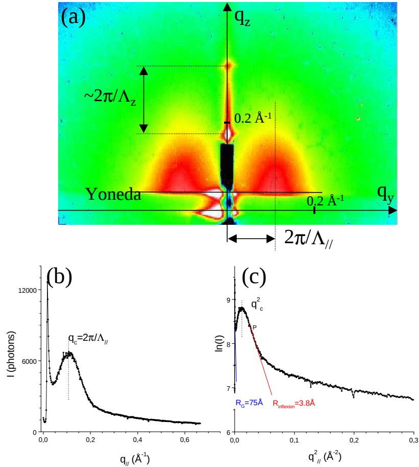
FIG. 4.18 – Image GISAXS obtenue sur la multicouche [\text{Fe } 5.3 \text{ Å}/\text{ZrO}_2 \text{ } 32 \text{ Å}]_{20} recuite à 550^\circ\text{C} . Les variations de l'intensité diffusée dans la direction q_{//} au niveau de l'horizon du Yoneda est tracée en échelle linéaire en fonction q_{//} et en échelle logarithmique en fonction de q_{//}^2 (tracé de Guinier).
