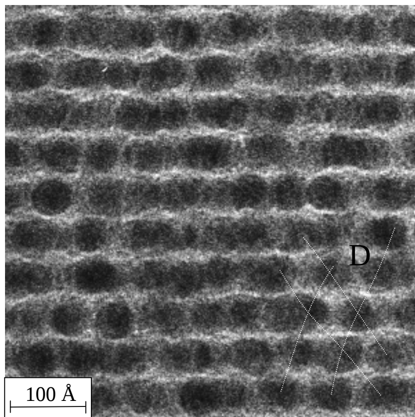
FIG. 4.11 – Clichés de microscopie électronique en transmission à haute résolution de MD [\text{Co } 15.3\text{\AA} / \text{SiO}_2 \text{ } 43\text{\AA}]_{20} pour des recuits effectués à 400 et 600°C. Le cobalt est en contraste sombre et la matrice de \text{SiO}_2 en contraste clair. Les régions A, B, C et D sont discutées dans le texte.
