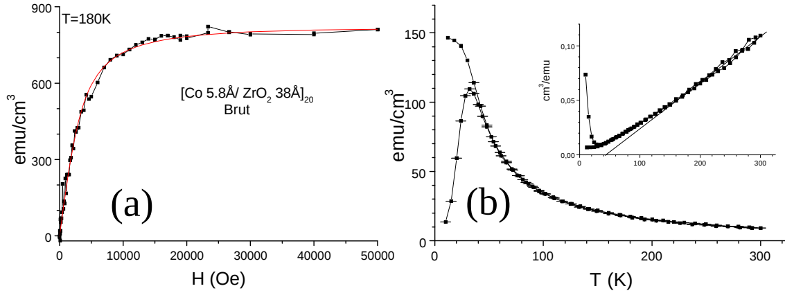
FIG. 6.8 – Magnétisme de la multicouche [\text{Co } 5.8 \text{ \AA} / \text{ZrO}_2 \text{ } 38 \text{ \AA}]_{20} brute de dépôt. (a) Cycle d'aimantation mesuré à 180K. (b) Courbe ZFC-FC avec H=100\text{Oe} . En insertion, inverse de l'aimantation mesurée dans le cycle ZFC-FC.
