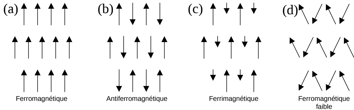
FIG. 2.5 – Orientations possibles des moments magnétiques dans les métaux Fe et Co, et leurs oxydes. (a) Ferromagnétisme dans \alpha\text{-Fe} et \alpha\text{-Co} . (b) Antiferromagnétisme (orientations antiparallèles) dans les oxydes CoO, FeO, et \alpha\text{-Fe}_2\text{O}_3 , T < T_{\text{Morin}} = 265\text{K} . (c) Ferrimagnétisme (deux sous réseaux d'orientations indépendants) dans \text{Fe}_3\text{O}_4 et \gamma\text{-Fe}_2\text{O}_3 . (d) ferromagnétisme faible (désorientation des moments antiparallèles due à des frustrations d'orientations et des défauts de position) \alpha\text{-Fe}_2\text{O}_3 , T > 265\text{K} .
