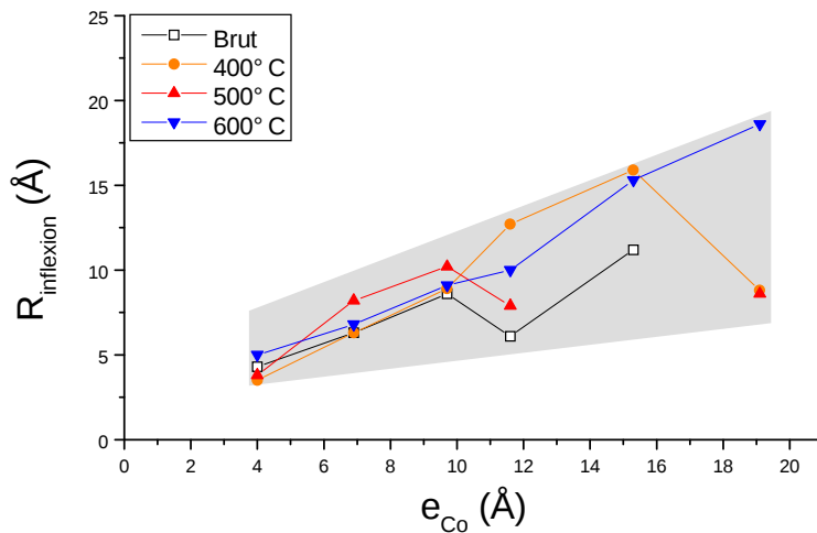
FIG. 4.32 – Valeurs du rayon de giration R_{inflexion} , mesuré au moyen de la pente au point d'inflexion de l'intensité dans le tracé de Guinier, dans les multicouches [Co\ e_{Co} / SiO_2\ 43\text{\AA}]_{20} en fonction de l'épaisseur de cobalt déposée, e_{Co} , et du traitement thermique (brut de dépôt, recuit à 400, 500 et 600°C).
