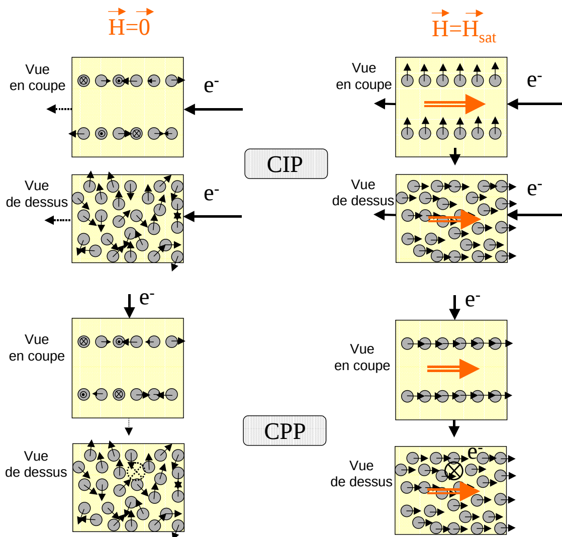
FIG. 2.20 – Géométrie Current-In-Plane (CIP) et Current-Perpendicular-to-Plane (CPP). La MD est vue du dessus (perpendiculairement aux plans des couches) ou de côté en coupe. Gauche : configuration magnétique à champ nul ou faible (résistance maximale et \vec{M} = \vec{0} ). On a supposé un couplage antiferromagnétique d'une particule d'une couche à celle d'une autre. Droite : configuration magnétique à saturation (résistance minimale et \vec{M} = \vec{M}_{\text{SAT}} ). Le vecteur \vec{H} est matérialisé par une flèche épaisse.
