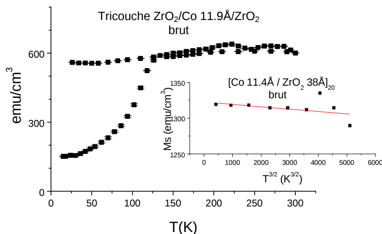
FIG. 6.11 – Courbe ZFC-FC d'une trilocouche ZrO_2/Co\ 11.9\text{\AA}/ZrO_2 brute de dépôt avec H=100\text{Oe} . Les fluctuations des mesures d'aimantation sont liées à la faiblesse du signal. En insertion : variation de l'aimantation à saturation déduite de l'aimantation à 20 et 30 kOe de la multicouche [Co\ 11.4\text{\AA}/ZrO_2\ 38\text{\AA}]_{20} brute de dépôt en fonction de T^{3/2} (point). Ajustement par la loi de Bloch (ligne continue).
