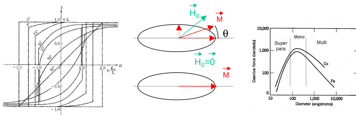
FIG. 2.8 – Gauche : Cycle d'aimantation d'une particule anisotrope en fonction de l'angle entre l'axe de facile aimantation et le champ appliqué (d'après [Chik 97]). Milieu : Directions de \vec{M} en fonction de celle du champ magnétique appliqué \vec{H}_0 . A champ nul, \vec{M} est dirigé selon l'axe de plus grande dimension. Droite : Détermination expérimentale du champ coercitif en fonction du diamètre des particules de Fe et de Co à 77K [Morr 65]. Le maximum de coercitivité ( D_M \sim 100\text{\AA} ) est atteint pour des particules monodomaines ferromagnétiques. Pour D < D_M , les particules sont monodomaines superparamagnétiques. Pour D > D_M , les particules sont multidomaines.
