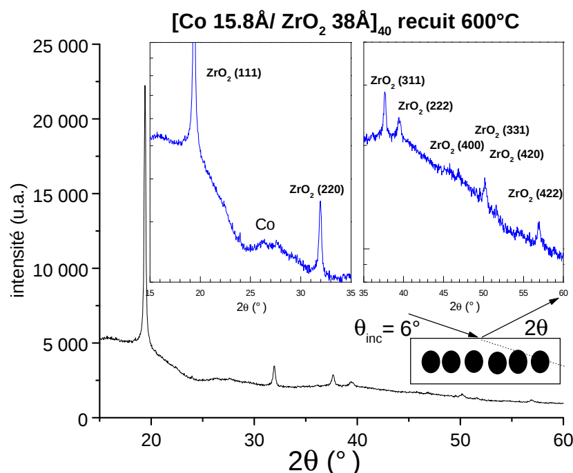
FIG. 5.2 – Diffraction X à aux grands angles en incidence rasante sur une multicouche [\text{Co } 15.8\text{\AA} / \text{ZrO}_2 \text{ } 38\text{\AA}]_{40} recuite à 600^\circ\text{C} . Le spectre a été réalisé sur BM32 sous une incidence de 6^\circ et pour \lambda=0.98\text{\AA} .
