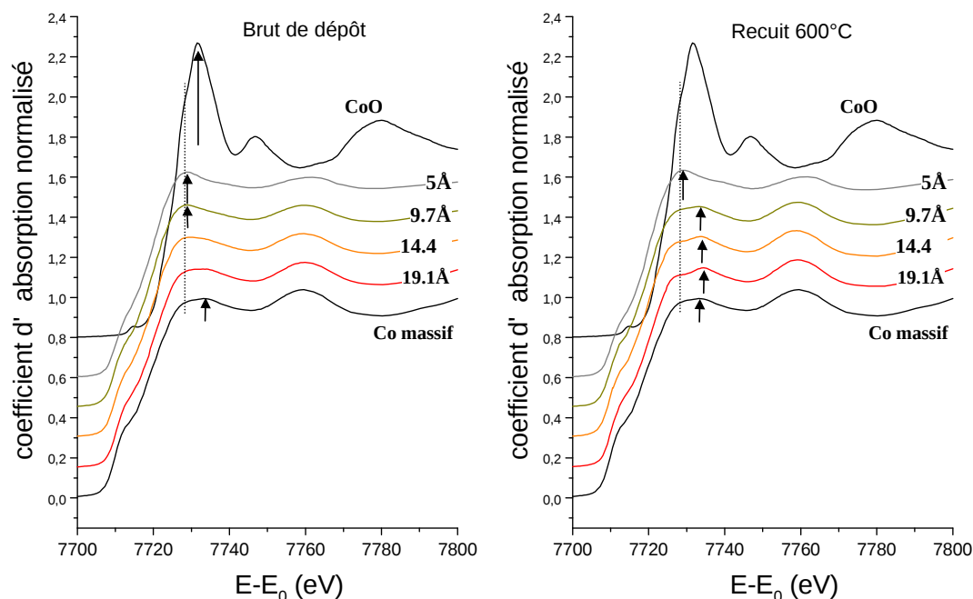
FIG. 5.24 – Région du seuil d'absorption K du cobalt et partie XANES correspondante aux multicouches [\text{Co}_{e_{\text{Co}}}/\text{SiO}_2 \text{ 41 \AA}]_{40} (seconde série) brutes de dépôt (à gauche) et recuites à 600°C (à droite).
