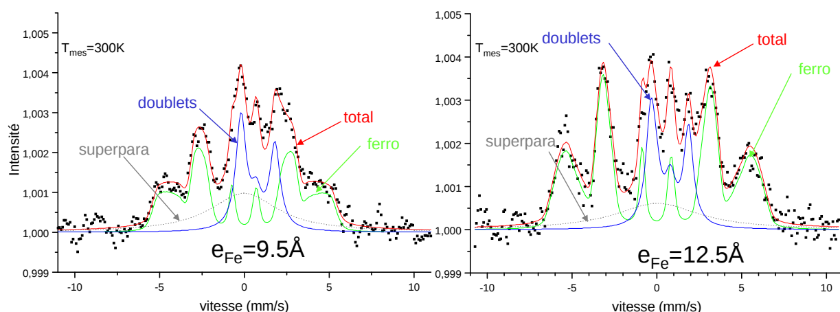
FIG. 5.25 – Spectres Mössbauer de multicouches Fe/ZrO 2 mesurés à 300K pour deux épaisseurs de fer déposées, e_{\text{Fe}}=9.5 et 12.5Å. La composante magnétique est composée du sextuplet ferromagnétique et du pic large superparamagnétique situé vers v=0 mm/s. Les deux doublets correspondent à la composante des ions fer. Le signal total est le résultat d'un ajustement des points expérimentaux composant le spectre.
