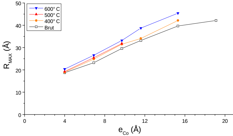
FIG. 6.22 – Valeurs du rayon de la plus grande particule, en fonction de e_{Co} et du recuit thermique, dans les multicouches [Co\ e_{Co}/SiO_2\ 43\text{Å}]_{20} .
