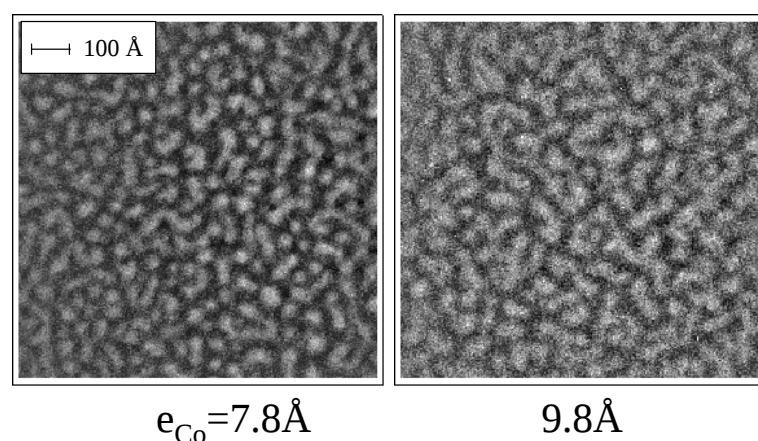
FIG. 4.10 – Cartographie chimique du cobalt sur des vues planes de tricouches \text{ZrO}_2/\text{Co}/\text{ZrO}_2 brutes de dépôt de la seconde série ( v_{\text{Co}}=0.5\text{\AA}/\text{s} ) en fonction de l'épaisseur de cobalt déposée e_{\text{Co}} pour une épaisseur de \text{ZrO}_2 de 41\text{\AA} . Le cobalt est en contraste clair et la matrice de \text{ZrO}_2 en contraste foncé. Les distances bord à bord sont estimées entre 25 et 30\text{\AA} .
