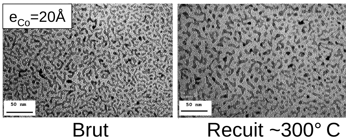
FIG. 4.15 – Vues planes en haute résolution de tricouches \text{SiO}_2/\text{Co}/\text{SiO}_2 brute de dépôt et recuite sous le faisceau électronique (température de recuit estimée à 300^\circ\text{C} ). L'épaisseur de cobalt déposée est de 20\text{\AA} et celle de \text{SiO}_2 de 200\text{\AA} . Le cobalt et la matrice de \text{SiO}_2 sont respectivement en contraste sombre et clair.
