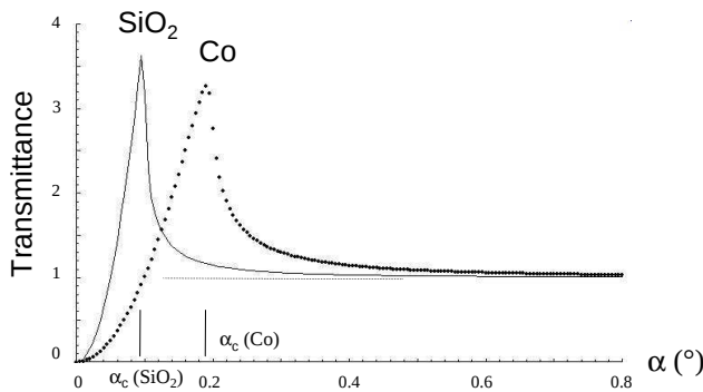
FIG. 3.14 – Variation de la transmittance en fonction de l'angle d'incidence \alpha dans le cas de Co et \text{SiO}_2 . A l'angle critique, on observe une exaltation de l'amplitude réfractée. Réciproquement, l'intensité émergente à l'angle \alpha suit la même loi. Il n'y a pas pratiquement d'intensité diffusée en dessous de l'angle donné par le pic de Yoneda.
