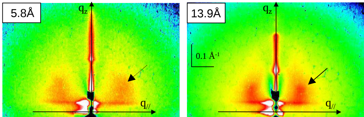
FIG. 4.20 – Figures GISAXS des multicouches [Co/ZrO 2 22Å] brutes de dépôt pour deux épaisseurs de cobalt déposées. Les flèches indiquent la position d'une tache de diffusion hors des axes q_z et q_{//} .
