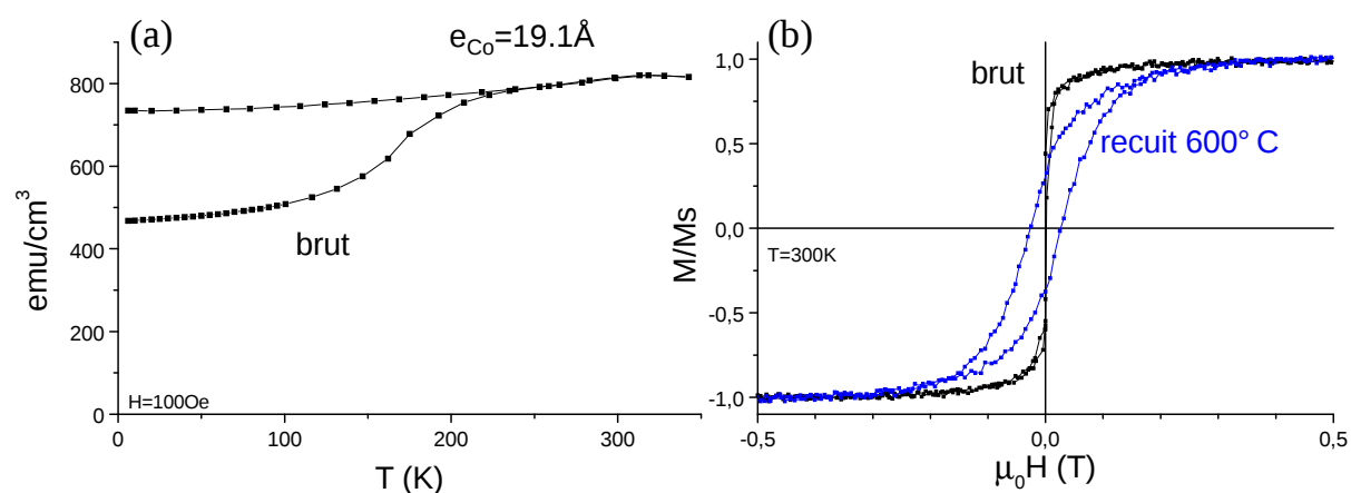
FIG. 6.18 – Mesures magnétiques effectuées sur les multicouches [\text{Co } 19.1 \text{ \AA} / \text{SiO}_2 \text{ } 43 \text{ \AA}]_{20} brute de dépôt et recuite à 600°C : (a) courbe ZFC-FC avec H = 100 \text{ Oe} ; (b) cycles d'aimantation mesurés au VSM à 300K.
