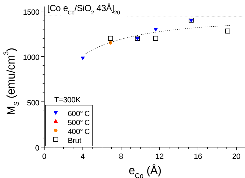
FIG. 6.19 – Valeur de l'aimantation à saturation mesurée au SQUID ou au VSM à 300K des multicouches [Co e_{Co}/SiO_2 43\text{\AA}]_{20} en fonction de l'épaisseur de cobalt déposée e_{Co} et du recuit thermique. La dispersion des valeurs par rapport au modèle de couche morte (ligne pointillée) est due à l'erreur d'estimation de la surface de l'échantillon pour connaître le volume de cobalt présent dans l'échantillon. La valeur de M_s dans du cobalt massif est indiquée par une droite horizontale.
