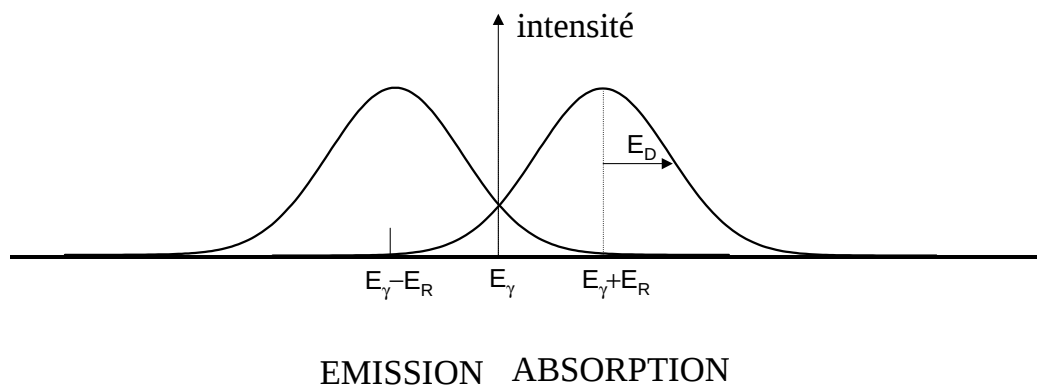
FIG. 3.18 – Superposition des probabilités d'émission et d'absorption en fonction de l'énergie. La partie commune des spectres de probabilité correspond à la probabilité d'émission et d'absorption d'un photon \gamma par un atome émetteur et un atome absorbeur agités thermiquement (largeur E_D ) et non ancrés dans un cristal (énergie de recul \pm E_R ).
