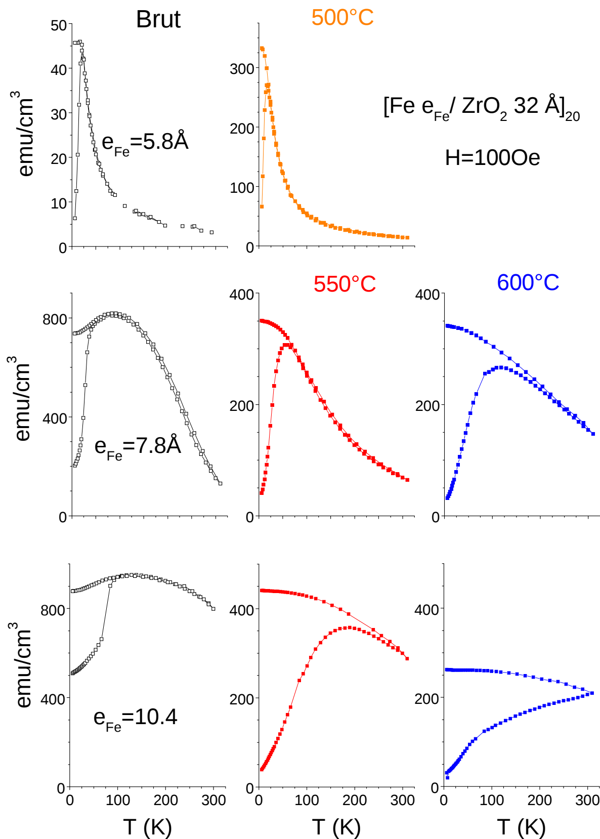
FIG. 6.1 – Courbes ZFC-FC des multicouches [\text{Fe } e_{\text{Fe}} / \text{ZrO}_2 \text{ } 32 \text{ Å}]_{20} brutes de dépôt et recuites à 500, 550 et 600°C. Le champ appliqué est de 100 Oe. La multicouche d'épaisseur e_{\text{Fe}} = 5.8 \text{ Å} est recuite à 500°C, celles d'épaisseur e_{\text{Fe}} = 7.8 et 10.4 Å le sont à 550 et 600°C.
