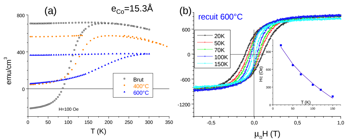
FIG. 6.17 – Mesures magnétiques effectuées sur la multicouche [\text{Co } 15.3 \text{ \AA} / \text{SiO}_2 \text{ } 43 \text{ \AA}]_{20} brute de dépôt ou recuite à 400 et 600°C : (a) Courbes ZFC-FC en fonction du traitement thermique avec H = 100 \text{ Oe} ; (b) Cycles d'aimantation de la multicouche recuite à 600°C mesurés à plusieurs températures. En insertion : variation du champ coercitif avec la température.
