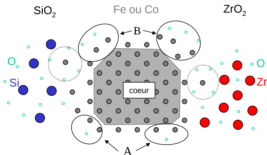
FIG. 6.25 – Schéma de l'ordre local autour des atomes de métal selon leur position éventuelle dans les multicouches discontinues : au cœur de l'agrégat ordonné (zone sombre), en bordure d'agrégats (zones A et B selon la cohérence avec la structure atomique au cœur) ou isolés des atomes de métal et entourés d'atomes d'oxygène, à proximité de l'agrégat (zones pointillées) ou à l'intérieur de la matrice (non représenté). La position des atomes en (A) est cohérente avec celles des atomes au cœur, à l'inverse des atomes en (B). La matrice de \text{SiO}_2 est supposée amorphe et celle de \text{ZrO}_2 cristallisée. Les moments des atomes de métal dans le cœur ont un comportement ferromagnétique ou superparamagnétique selon la taille de l'agrégat, la température et le temps caractéristique de mesure. Les atomes de cœur sont métalliques M^0 . Ceux entourés complètement d'atomes d'oxygène sont des ions de charge entière : \text{Fe}^{2+} , \text{Fe}^{3+} , \text{Co}^{2+} et \text{Co}^{3+} . Leur moment magnétique possède un comportement paramagnétique. Les atomes des régions (A) et (B) ont un degré d'oxydation variable M^{\delta+} selon le nombre de liaisons M-O mises en jeu, et leurs moments couplés entre eux et avec ceux des atomes de cœur ont un comportement intermédiaire entre celui du paramagnétisme et du ferromagnétisme.
