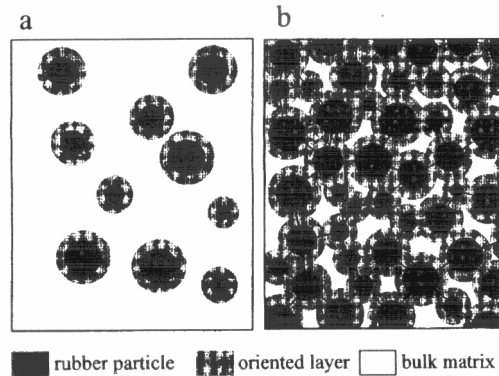
Figure 33 : Représentation schématique de l'interphase entre nodule et polymère semi-cristallin : a) ID_c > 2 \cdot dimension de l'interphase : comportement fragile ; b) ID_c < 2 \cdot dimension de l'interphase : phénomène de percolation entre les différentes interphases entraînant le développement d'une plasticité étendue [99].
