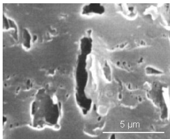
Figure 9 : Clichés de microscopie électronique à balayage : PP renforcé au choc sollicité en traction uniaxiale à (60°C, 10^{-5} s^{-1} ) (l'image de droite correspond à un agrandissement de la zone cerclée de blanc sur la photo de gauche).
