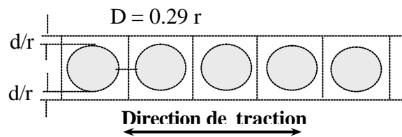
Figure 9 : Représentation schématique d'un matériau renforcé sollicité sous la forme d'une couche mince : V_f = 20\% .
