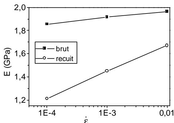
Figure 4: Evolution du module d'Young du PP modifié en fonction de la vitesse de déformation : matériau à l'état brut et recuit ( T = 20^{\circ}\text{C} ).
