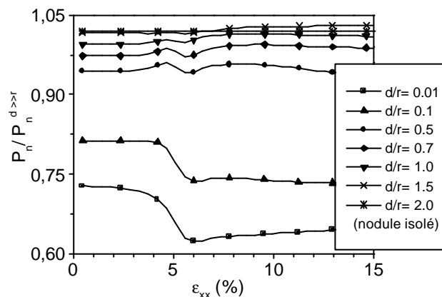
Figure 26 : Dépression dans le nodule normalisée par la dépression lors que le milieu peut être considéré comme infini ( d \gg r ) en fonction de la distance à la surface libre : V_f = 1\% .
