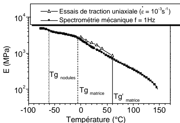
Figure 3 : Evolution du module d'Young en fonction de la température pour des essais de traction uniaxiale quasi-statiques ( \dot{\epsilon} = 10^{-3} \text{s}^{-1} ) et dynamiques .
