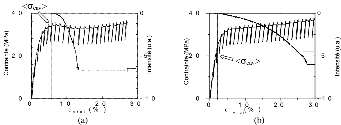
Figure 5 : Mesure de l'intensité transmise par deux PMMA renforcés initialement transparents au cours d'un essai de traction uniaxiale (20°C, 10 -3 s -1 ) : a) matériau de type 'A' ; b) matériau de type 'B'.
