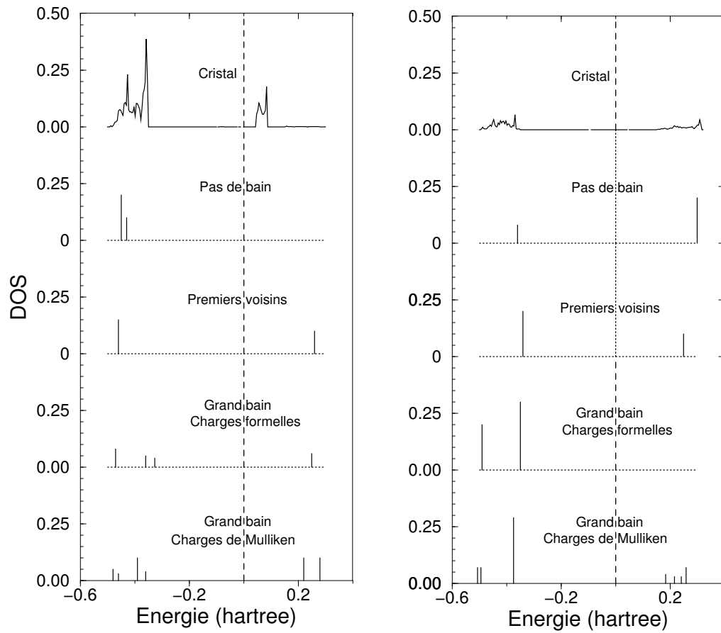
FIG. 6.17 – Densité d'état projetée sur les orbitales 2p_x (à gauche) et 2p_z (à droite) de l'oxygène central des barreaux. Le calcul HF sur le cristal est donné en haut. Suivent en descendant les résultats HF sur le fragment nu, sur le fragment immergé dans un bain comprenant les premiers voisins des atomes du fragment, dans un grand bain de 13\text{\AA} de rayon centré sur le fragment, formé par les charges formelles, puis le même bain formé avec les charges de Mulliken.
