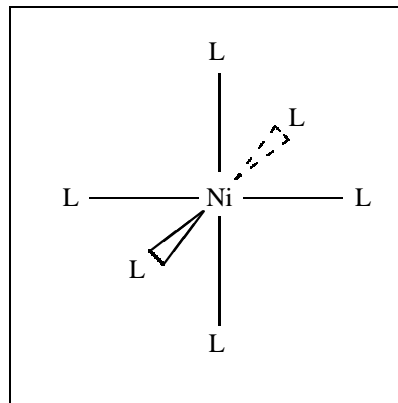
FIG. 1.3 – Un atome de nickel dans un environnement octaédrique de ligands L.
