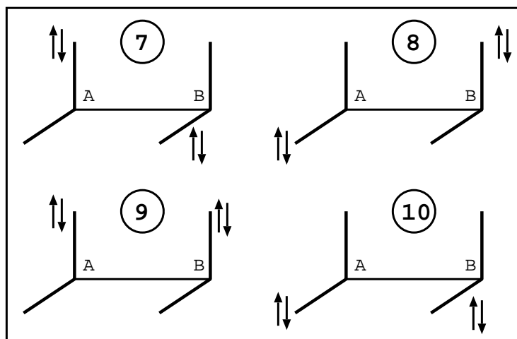
FIG. 3.5 – Les déterminants pseudo-ioniques à deux couches fermées.
