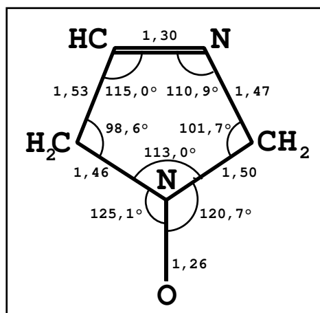
FIG. 5.12 – Structure de l'imidazoline choisie comme second modèle au radical nitroxyde. Les distances sont données en angstroms.
