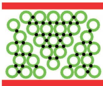
FIG. 3.38 – Inversion du faciès de rupture numérique pour \mu_{\text{inf}} = \mu_{\text{sup}} = 0,05
