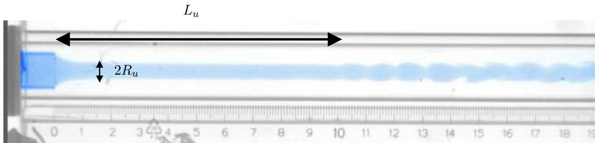
FIG. 3.3. Configuration des fluides w et o pour des débits d'injection respectifs : 0.27 \text{ cm}^3 \cdot \text{s}^{-1} et 0.68 \text{ cm}^3 \cdot \text{s}^{-1} . La longueur uniforme est notée L_u , et le rayon uniforme est noté R_u . R_u est imposé par le rapport des débits.
