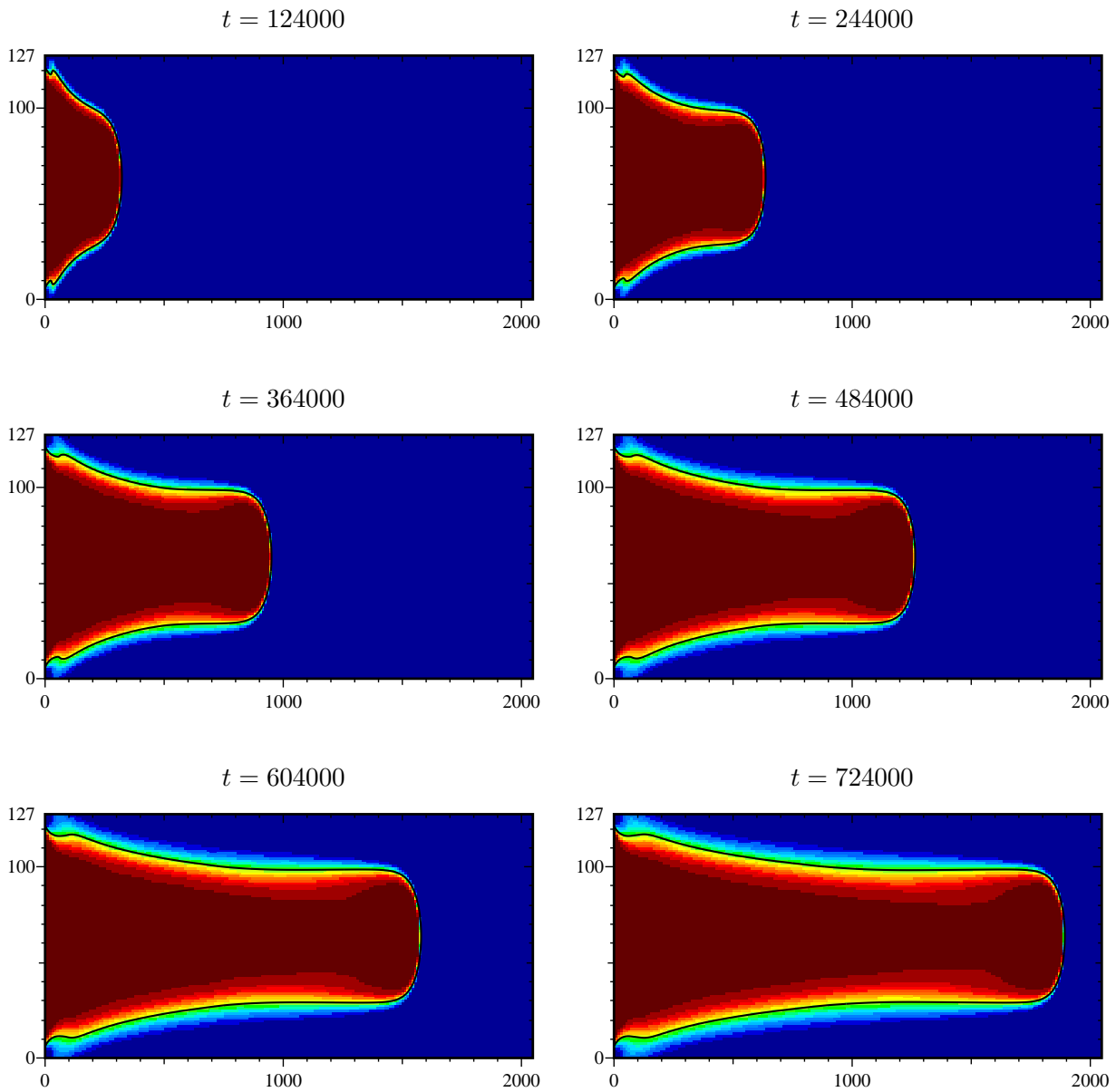
FIG. 1.2. Évolution du champ de concentrations en fonction du temps. La condition d'entrée est C_g = 0.85 . Les paramètres sont : M = 10 , u_0 = 16 \cdot 10^{-4} , D_0 = 5 \cdot 10^{-5} , Pe = 4096 et Re = 1 .
