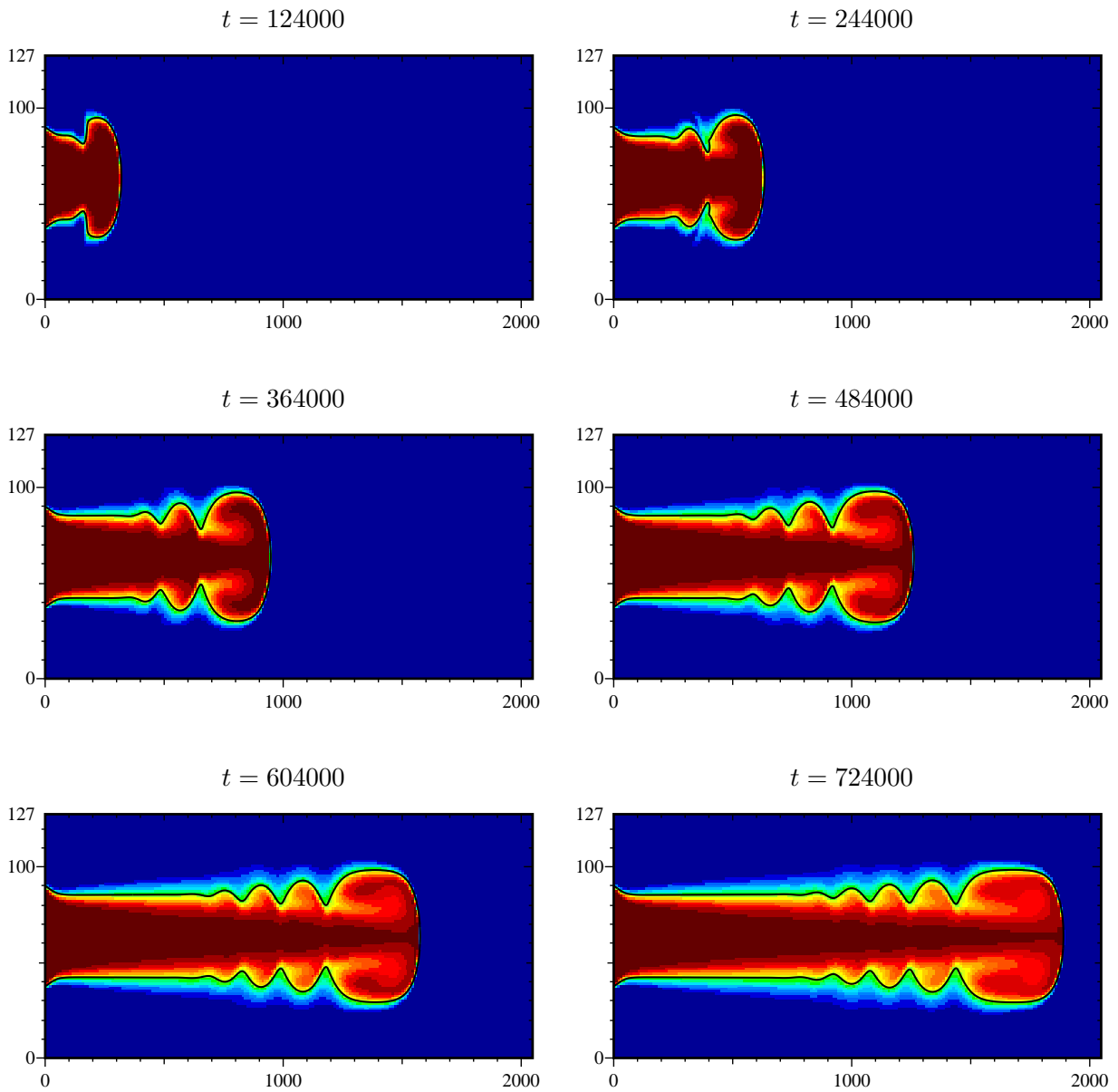
FIG. 1.3. Évolution du champ de concentrations en fonction du temps. La condition d'entrée est C_g = 0.4 . Les paramètres sont : M = 10 , u_0 = 16 \cdot 10^{-4} , D_0 = 5 \cdot 10^{-5} , Pe = 4096 et Re = 1 .
