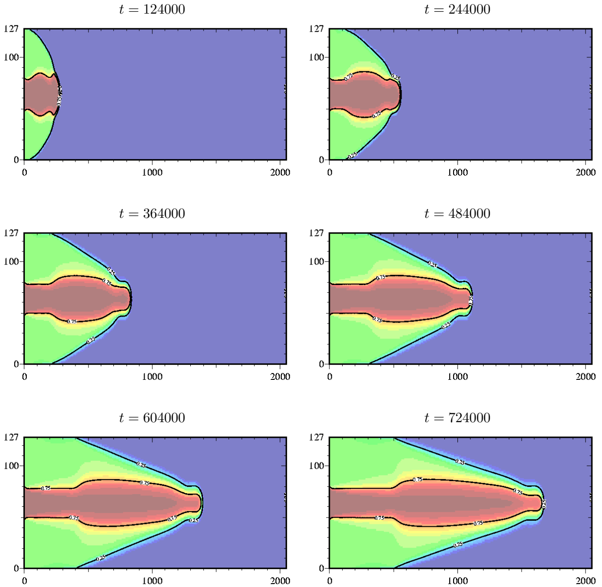
FIG. 4.1. Évolution du champ de concentrations en fonction du temps pour un système hyperbolique. La condition d'entrée est du type A \neq G . Les paramètres sont : M = 1 , \Lambda = 0.1 , u_0 = 16 \cdot 10^{-4} , D_0 = 5 \cdot 10^{-5} , Pe = 4096 .
