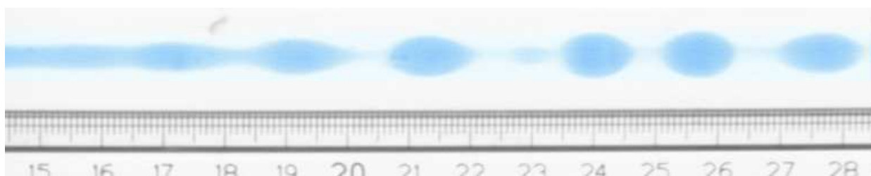
FIG. 3.5. Formation de "chapelets". Les débits respectifs du fluide w et o sont : 0.03 \text{ cm}^3 \cdot \text{s}^{-1} et 0.20 \text{ cm}^3 \cdot \text{s}^{-1} . Cette instabilité se forme à L_u = 15 \text{ cm} en aval de l'injection.
