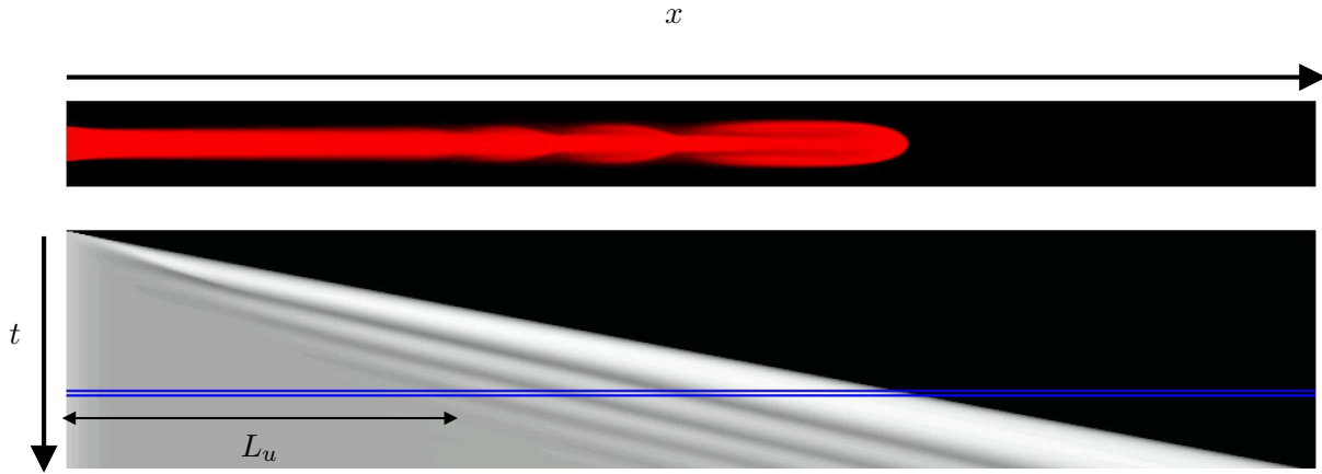
FIG. 1.4. Champ de concentrations et diagramme spatio-temporel de la concentration moyenne, pour la simulation de la figure 1.3. En haut, le champ de concentrations est représenté en rouge, il correspond au temps t = 484000 . En bas, diagramme spatio-temporel de la concentration moyenne. Les fortes saturations sont représentées en clair. La ligne en bleu correspond au temps de la configuration ci-dessus ( t = 484000 ). La longueur uniforme est notée L_u .
