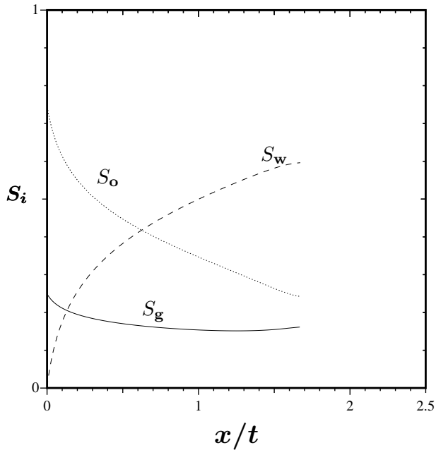
FIG. 2.9. Solution analytique du problème de Riemann dans le cas d'un système mixte : M = 1 et \Lambda = 10 . Le point de départ A correspond à S_g = 0.25 et S_o = 0.75 . La solution relie le point A au point B par une onde de raréfaction lente. Le point B est situé sur la frontière de la zone elliptique. Sur la figure du haut est représenté le chemin dans le plan (S_g, S_w) . En bas à gauche sont représentées les saturations de chacune des phases en fonction de la variable x/t . En bas à droite sont représentées les positions des interfaces g - o (ligne continue) et o - w (ligne pointillée) en fonction de x/t .
