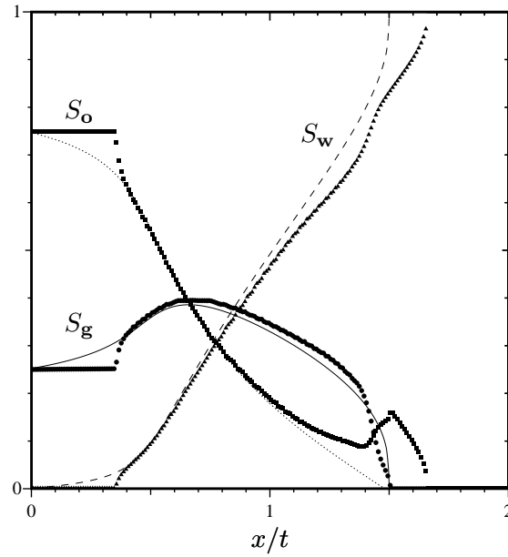
FIG. 3.4. Courbes des profils S_g , S_o et S_w correspondant à l'instant t = 501000 de la figure 3.2 en fonction de la variable x/t (normalisée par la vitesse débitante). Les courbes en traits fins représentent les profils de saturations obtenus par la courbe de raréfaction.
