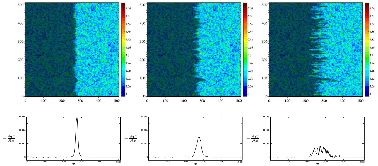
FIG. 5.4. Exemple de déplacement pour différents rapports de viscosités. A gauche : cas stable \beta = 0.4 . Au centre : cas du traceur \beta = 0 . A droite : cas instable \beta = -0.4 . Les autres paramètres sont : u_0 = 4.10^{-4} , D_0 = 10^{-4} , \sigma_f = 0.4 et \lambda = 2.2 . La carte de couleur représente le champ de perméabilités. Celui-ci est identique pour chacune des réalisations. Les niveaux de gris correspondent au champ de concentrations (noir pour C = 1 ). En bas sont tracés les gradients de concentration moyens correspondants : -\frac{\partial \bar{C}}{\partial x}(x) .
