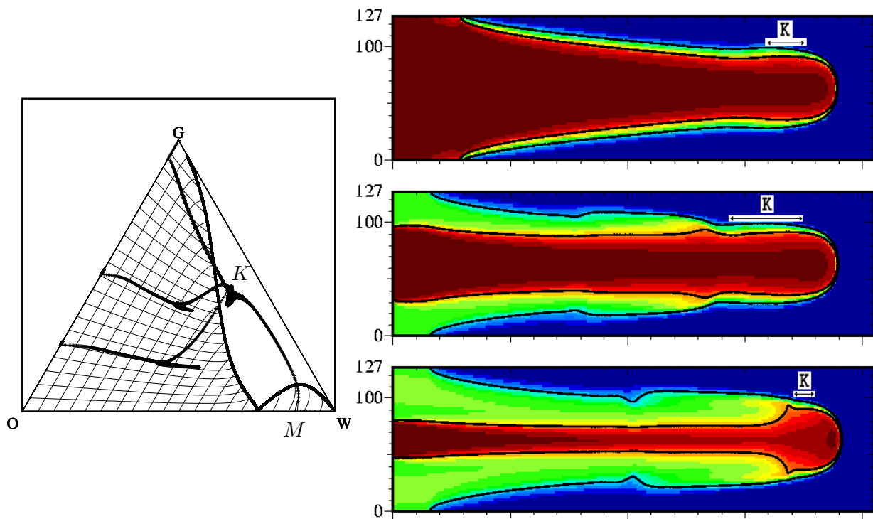
FIG. 4.9. Diagramme ternaire et configurations des fluides au même temps de simulations pour des conditions d'injection différentes. Les paramètres pour chacune des simulations sont : u_0 = 16 \cdot 10^{-4} , D_0 = 5 \cdot 10^{-5} , Pe = 4096 .
