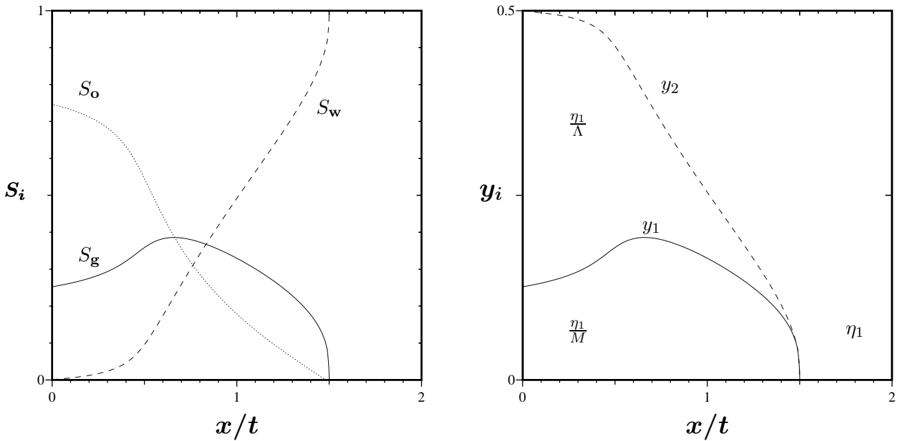
FIG. 2.8. Solution analytique du problème de Riemann dans le cas d'un système hyperbolique : M = 1 et \Lambda = 0.1 . Le point de départ A correspond à S_g = 0.25 et S_o = 0.75 . La solution relie le point A au point B par une onde de raréfaction lente. Le point B est ensuite connecté au point W par une autre raréfaction. Sur la figure du haut est représenté le chemin dans le plan (S_g, S_w) . En bas à gauche sont représentées les saturations de chacune des phases en fonction de la variable x/t . En bas à droite sont représentées les positions des interfaces g - o (ligne continue) et o - w (ligne pointillée) en fonction de x/t . Notons que l'axe x/t a été normalisé par u_0 .
