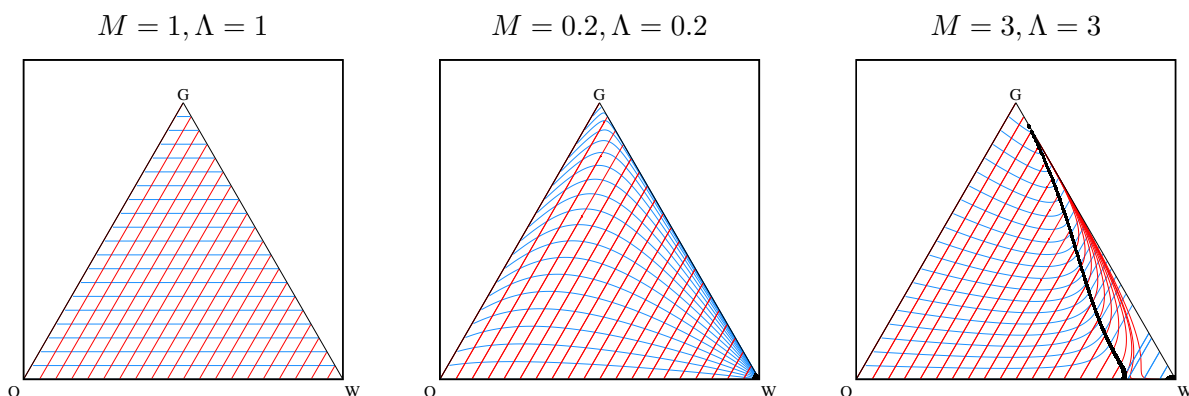
FIG. 2.5. Exemple de systèmes particuliers. A gauche toutes les phases ont la même viscosité. Au centre et à droite, \mathbf{g} et \mathbf{o} ont la même viscosité. On peut noter l'apparition d'une courbe de dégénérescence sur la figure de droite.
