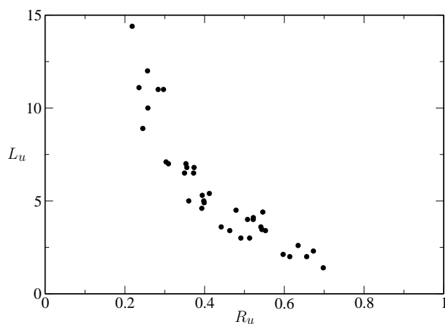
FIG. 3.4. Longueur uniforme L_u en fonction du rayon R_u . Les différentes expériences ont été faites pour des débits totaux différents, variant de 0.1 à 1 \text{ cm}^3 \cdot \text{s}^{-1} .
