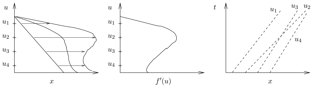
FIG. 1.2. Évolution d'un profil dans le cas d'un auto-raissement. A gauche : trois profils u(x) pour des instants différents, le troisième profil ne peut pas être une solution. Au centre : courbe des vitesses f'(u) , cette fonction n'est pas monotone. A droite : courbes caractéristiques de u_1, u_2, u_3 et u_4 . On note que les caractéristiques u_2 et u_3 se croisent, on doit avoir l'apparition d'un choc.
