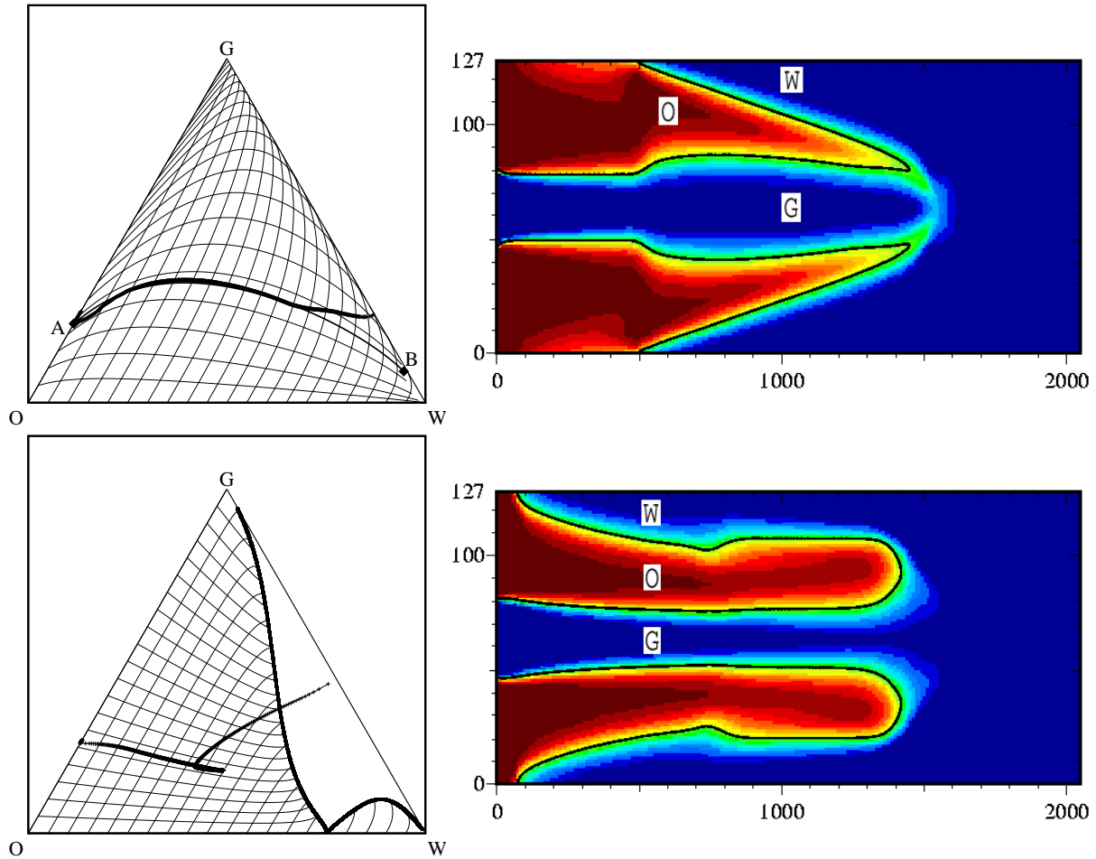
FIG. 4.1. Déplacement de deux fluides miscibles. Le fluide rouge ( \circ ) est injecté par l'extérieur, le fluide bleu ( \mathbf{w} , \mathbf{g} ) étant au centre. En haut, le fluide rouge est plus visqueux que le bleu. En bas, le fluide rouge est moins visqueux. Ce système peut être décrit par un modèle triphasique, similaire au cas M = 1 et \Lambda = 0.1 pour la simulation du haut et M = 1 et \Lambda = 10 pour celle du bas. Les autres paramètres sont : u_0 = 16 \cdot 10^{-4} , D_0 = 5 \cdot 10^{-5} , Pe = 4096 et Re = 4 .
