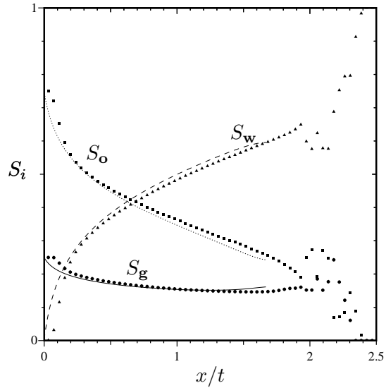
FIG. 3.8. Courbes des saturations S_g , S_o et S_w en fonction de la variable x/t (normalisée) pour la simulation de la figure 3.6.
