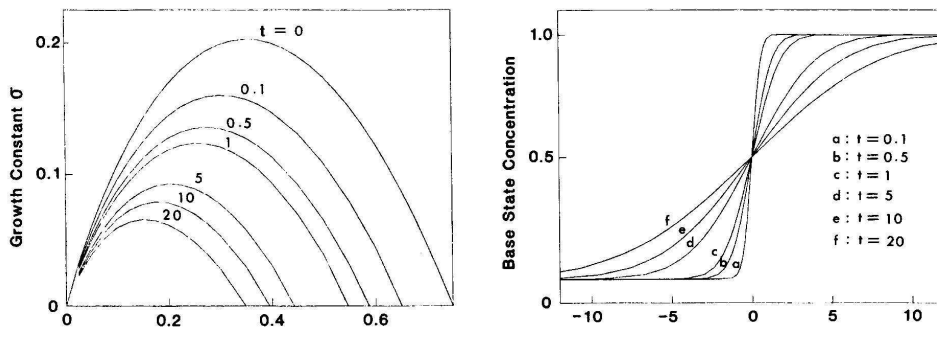
FIG. 5.3. Extrait de Tan et Homsy [88]. A gauche : taux de croissance en fonction du nombre d'onde et pour différents états de base, en milieu poreux homogène. A droite : états de bases pour différents temps t_0 . Ici, \beta = -3 . La variable temporelle est normalisée par D_0/u_0^2 et la variable spatiale par D_0/u_0 .
