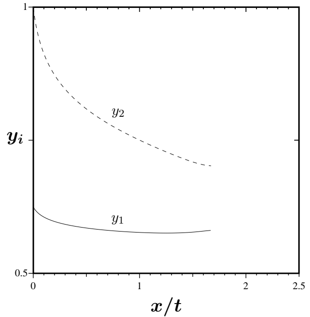
FIG. 2.9. Solution analytique du problème de Riemann dans le cas d'un système mixte : M = 1 et \Lambda = 10 . Le point de départ A correspond à S_g = 0.25 et S_o = 0.75 . La solution relie le point A au point B par une onde de raréfaction lente. Le point B est situé sur la frontière de la zone elliptique. Sur la figure du haut est représenté le chemin dans le plan (S_g, S_w) . En bas à gauche sont représentées les saturations de chacune des phases en fonction de la variable x/t . En bas à droite sont représentées les positions des interfaces g - o (ligne continue) et o - w (ligne pointillée) en fonction de x/t .
