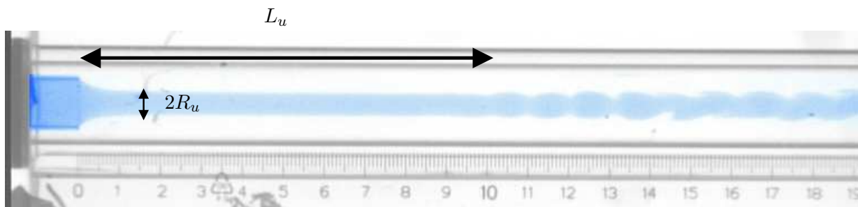
FIG. 3.3. Configuration des fluides w et o pour des débits d'injection respectifs : 0.27 \text{ cm}^3 \cdot \text{s}^{-1} et 0.68 \text{ cm}^3 \cdot \text{s}^{-1} . La longueur uniforme est notée L_u , et le rayon uniforme est noté R_u . R_u est imposé par le rapport des débits.
