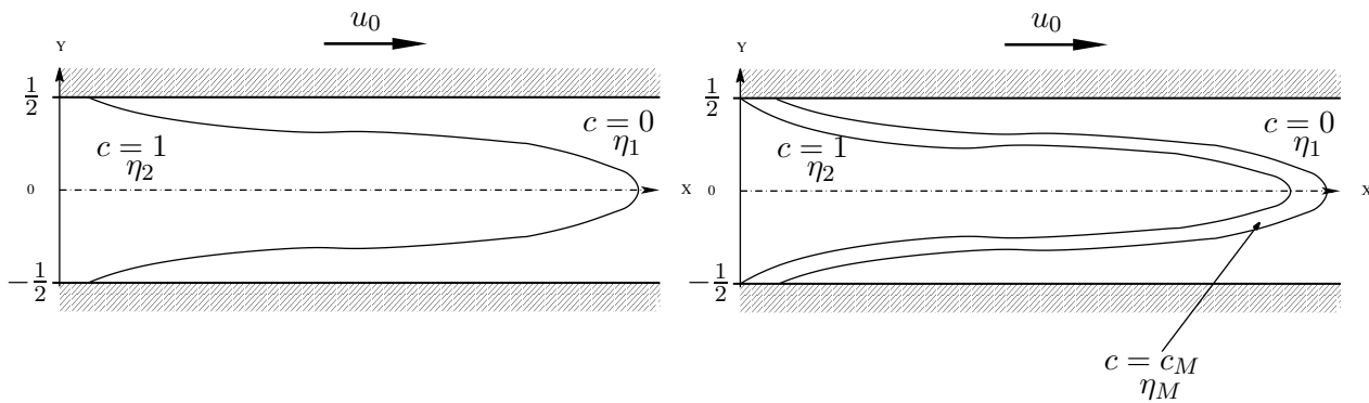
FIG. 6.2. Schéma du déplacement d'un fluide par un autre dans la tranche d'une cellule de Hele-Shaw. A gauche : il n'y a pas de mélange entre les deux fluides. A droite : le mélange entre les deux fluides fait intervenir une zone de concentration intermédiaire ( c_M ). Cette zone, dans le cas d'une loi de viscosité non-monotone, correspond à une viscosité extrême ( \eta_M ) dans le système.
