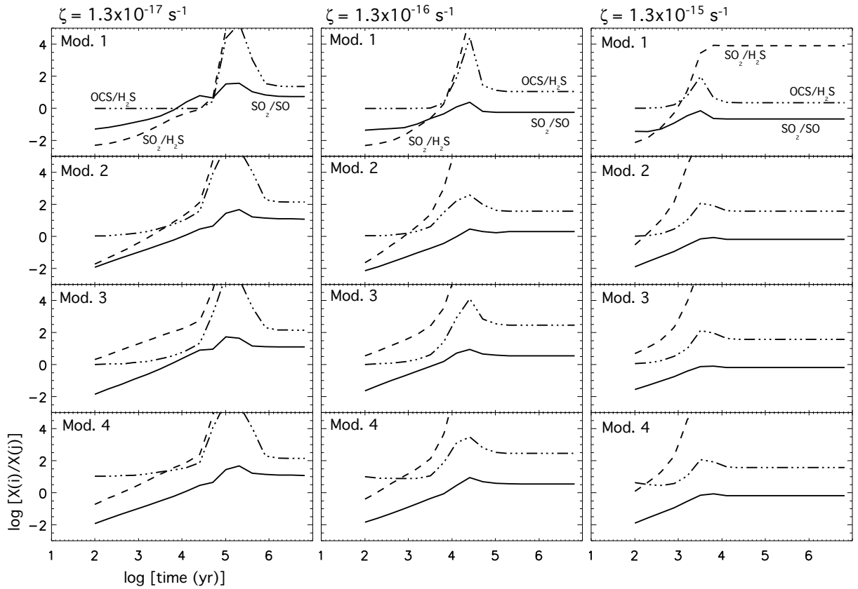
FIG. 55: Rapports d'abondance SO_2/SO , SO_2/H_2S et OCS/H_2S en fonction du temps pour une température de 100 K, pour une densité de 10^7 \text{ cm}^{-3} et pour les 4 compositions de grains (ligne 1 à 4: Modèle 1 à 4). Les trois colonnes représentent les abondances calculées avec un taux d'ionisation par le rayonnement cosmique différent. Première colonne : 1.3 \times 10^{-17} \text{ s}^{-1} (taux de référence), deuxième colonne : 1.3 \times 10^{-16} \text{ s}^{-1} et troisième colonne : 1.3 \times 10^{-15} \text{ s}^{-1} .
