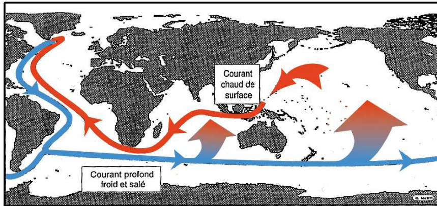
Figure 0.4 : Schéma de la circulation océanique actuelle décrit par W. Broecker. Les courants chauds de surface sont indiqués en rouge et les courants froids en profondeur sont indiqués en bleu. Il est à noter que ce schéma est une simplification extrême de la circulation océanique globale et ne décrit pas les différentes masses d'eau (formées en Atlantique nord ou autour de l'Antarctique) ni leurs mélanges. De même, la remontée des eaux en surface (en dégradé bleu-rouge sur les océans Indien et Pacifique) doit plutôt être perçue comme un phénomène de diffusion.
