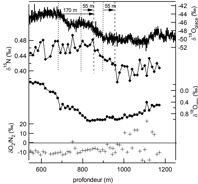
Figure 3.13 : Mesures effectuées dans la carotte de Kohnen Station (DML) sur la transition du dernier maximum glaciaire à l'Holocène (de haut en bas, \delta^{18}\text{O}_{\text{glace}} , \delta^{15}\text{N} , \delta^{18}\text{O}_{\text{atm}} et \delta\text{O}_2/\text{N}_2 ). Le \delta^{18}\text{O}_{\text{atm}} a été corrigé de l'effet gravitationnel uniquement selon \delta^{18}\text{O}_{\text{atm}} = \delta^{18}\text{O} - 2\delta^{15}\text{N} (l'erreur effectuée sur la valeur vraie de \delta^{18}\text{O}_{\text{atm}} en négligeant l'effet thermique est ici inférieure à 0,02‰). Le profil de \delta^{18}\text{O}_{\text{glace}} a été mesuré à Potsdam entre 2002 et 2004 [Oerter et al., in press ; H. Meyer et H. Oerter, AWI, comm. pers.].
