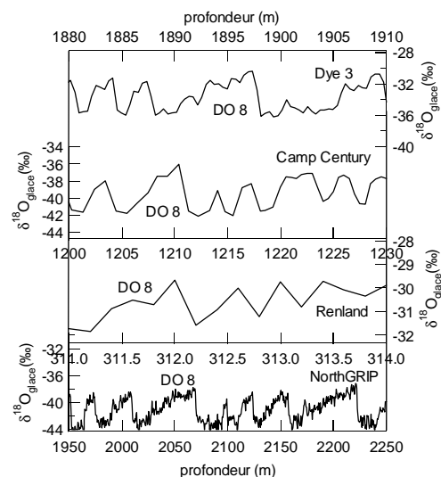
Figure 6.13 b : Comparaison des enregistrements en \delta^{18}O_{\text{glace}} sur l'événements de DO 8 à Dye 3 [Dansgaard et al., 1982], Camp Century [Johnsen et al., 1972], Renland [Johnsen et al., 1992] et NorthGRIP [NorthGRIP community members, 2004]. La résolution des mesures est la meilleure à NorthGRIP (GRIP non montré a aussi une résolution importante jusqu'à -110 000 ans).
