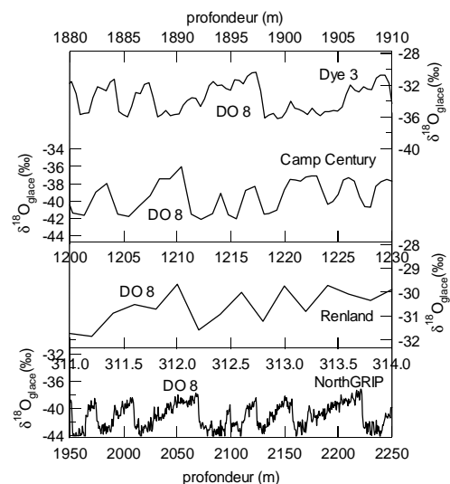
Figure 6.13 b : Comparaison des enregistrements en \delta^{18}O_{glacé} sur l'événements de DO 8 à Dye 3 [Dansgaard et al., 1982], Camp Century [Johnsen et al., 1972], Renland [Johnsen et al., 1992] et NorthGRIP [NorthGRIP community members, 2004]. La résolution des mesures est la meilleure à NorthGRIP (GRIP non montré a aussi une résolution importante jusqu'à -110 000 ans).
