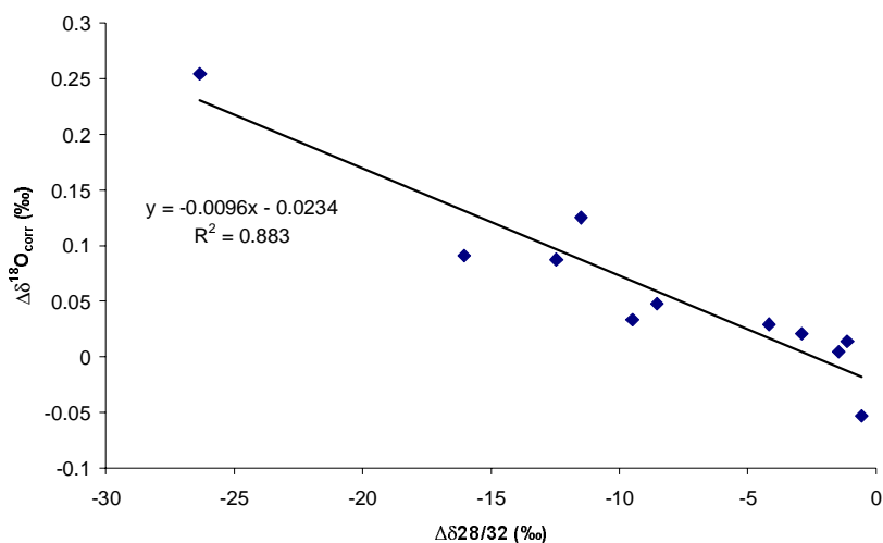
Figure 2.8 : Evolution de la différence \Delta\delta^{18}O en fonction de la différence \Delta\delta_{28/32} sur des échantillons prélevés au fond de la carotte groenlandaise de GRIP. Les différences sont calculées entre des échantillons de même profondeur. Une régression linéaire (méthode des moindres carrés) a été effectuée.
