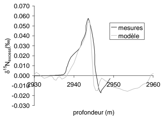
Figure 6.7 b : sur l'événement 24, variation de \delta^{15}N_{excess} obtenue d'après les mesures (moyenne glissante sur 3 points) et modélisée avec une amplitude de 16°C pour le réchauffement. Le profil de \delta^{15}N_{excess} modélisé a été décalé de 2 mètres pour faire correspondre les deux pics (la datation utilisée actuellement comme forçage pour les événements de Dansgaard-Oeschger 23 et 24, ss06 de S. Johnsen, doit être améliorée)
