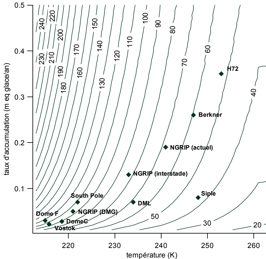
Figure 3.12 : Evolution de la zone de fermeture des pores donnée par le modèle de Jean-Marc Barnola [Goujon et al., 2003] en fonction du taux d'accumulation et de la température moyenne annuelle. Les principaux sites étudiés ont été reportés sur ce graphique avec leurs caractéristiques de surface. Pour NorthGRIP, qui est le site le plus étudié dans cette thèse, nous avons reporté les caractéristiques pour le dernier maximum glaciaire et pour la période chaude d'un événement de Dansgaard-Oeschger moyen (interstade). Les caractéristiques de NorthGRIP en période glaciaire sont les mêmes que celles de plusieurs sites en Antarctique actuellement.
