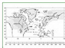
1 : Carte des environs de l'Atlantique nord en période glaciaire
