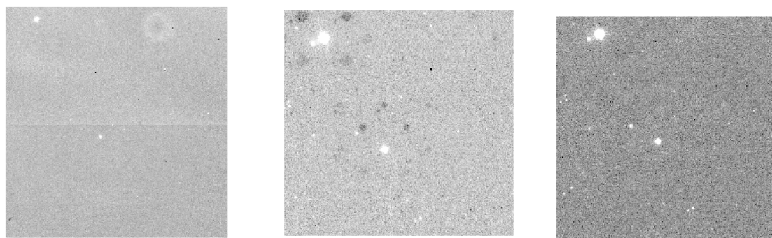
FIG. E.1 – Images NTT de l'objet DENIS-001000, de gauche à droite : sans traitement, après traitement mais présentant un problème de ciel, après traitement corrigé.
