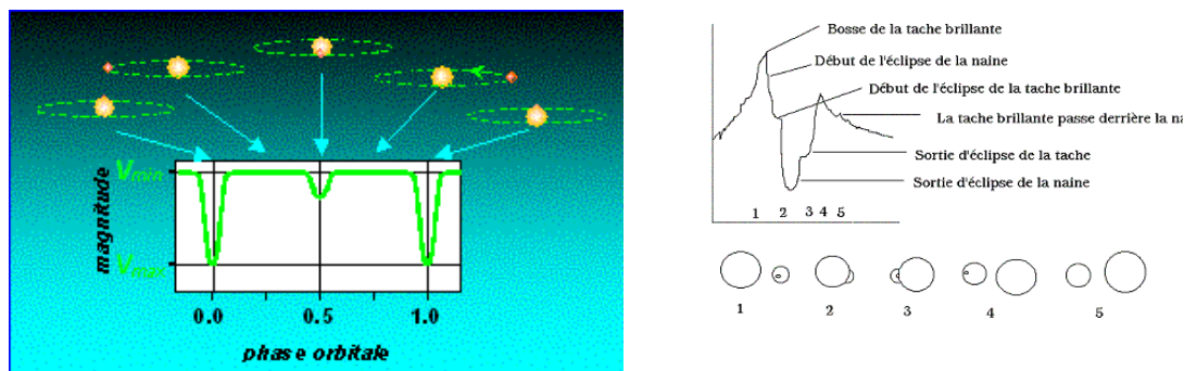
FIG. B.2 – A gauche (source : wwwrc.obs-azur.fr ) : variations de luminosité d'une étoile double du à la présence d'un compagnon. Dans la figure de droite (source : www.astrosurf.com ), on distingue en plus le phénomène annexe d'occultation d'une tache présente sur le compagnon.
