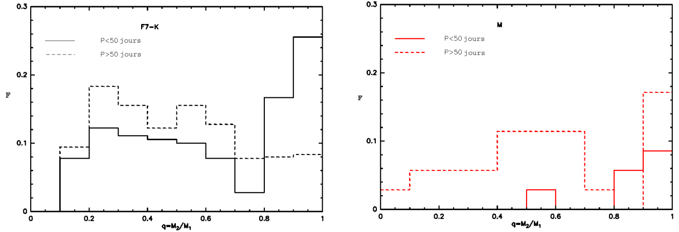
FIG. 9.3 – Distribution en rapport de masse des binaires par rapport à la période. A gauche : Etude des naines F à K (Halbwachs et al. 2003); à droite : notre étude.
