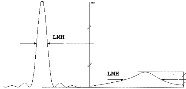
FIG. C.3 – Définition de la largeur à mi-hauteur (LMH) caractérisant la qualité d'une image. A gauche, coupe d'une image parfaite, théorique. A droite, la coupe d'une image dont la résolution est limitée par la turbulence.
