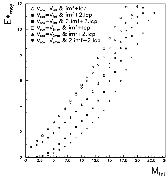
FIG. 5.3 – Xe+Sn , 80 \text{ MeV}/A : Représentation de l'énergie d'excitation moyenne E_{moy}^* (en \text{MeV}/A ) en fonction de la multiplicité totale M_{tot} . Différents calculs sont testés en considérant plusieurs hypothèses (sur la vitesse de la source V_{sou} et sur l'origine des particules). La courbe la plus réaliste est tracée avec les points noirs et correspond à V_{sou} = V_{imf} et E^* calculée avec les fragments à l'avant de l'ellipsoïde et les particules légères à l'avant de la source.
