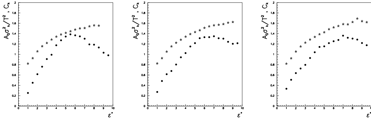
FIG. 5.10 – Xe+Sn , 65-80-100 MeV/A : Même présentation que celle de la figure (5.9) correspondant aux événements les plus compacts pour trois énergies de bombardement différentes. Cette fois-ci, aucun signal n'est observé.
