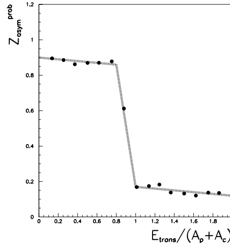
FIG. 3.12 – Xe+Sn , 80 MeV/A : Représentation de Z_{asym} = \frac{Z_1-Z_2}{Z_1+Z_2} la plus probable en fonction de l'énergie transverse normalisée \frac{E_{trans}}{A_p+A_c} exprimée en MeV/A . On observe un saut pour E_{trans} proche de 250 MeV .
