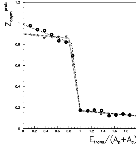
FIG. 3.24 – Au+Au, 80 \text{ MeV}/A : Représentation de Z_{asym} = \frac{Z_1-Z_2}{Z_1+Z_2} la plus probable en fonction de l'énergie transverse normalisée \frac{E_{trans}}{A_p+A_c} exprimée en \text{MeV}/A . Les points noirs correspondent au système Au+Au tandis que les étoiles reprennent le résultat de la figure (3.12) pour Xe+Sn . On observe un saut à la même E_{trans} normalisée pour les deux systèmes.
