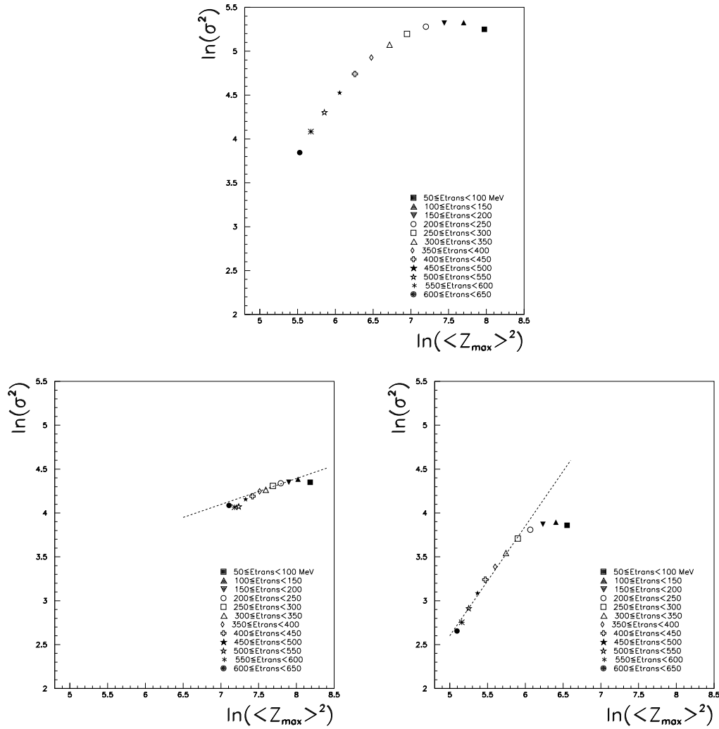
FIG. 4.10 – Au+Au, 80 \text{ MeV}/A : \ln(\sigma^2) = f(\ln(\langle Z_{max} \rangle^2)) , même présentation que la figure (4.5) : en haut quelque soit Z_{asym} , en bas à gauche pour Z_{asym} > 0,7 et en bas à droite pour Z_{asym} < 0,3 . Les valeurs obtenues sont respectivement \Delta = 0,3 et \Delta = 1,2 .
