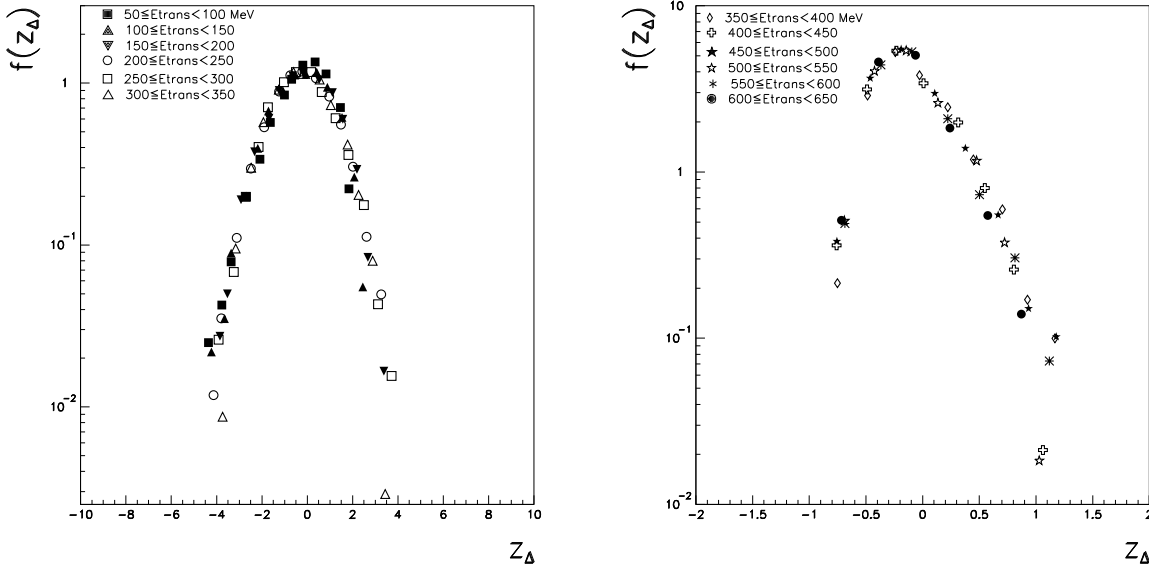
FIG. 4.9 – Au+Au, 80 MeV/A : La première figure est telle que Z_{asym} > 0,7 et \Delta = \frac{1}{2} pour E_{trans} < E_{bimod} et la seconde telle que Z_{asym} < 0,3 et \Delta = 1 pour E_{trans} > E_{bimod} . Comme pour la figure (4.4), deux familles apparaissent.
