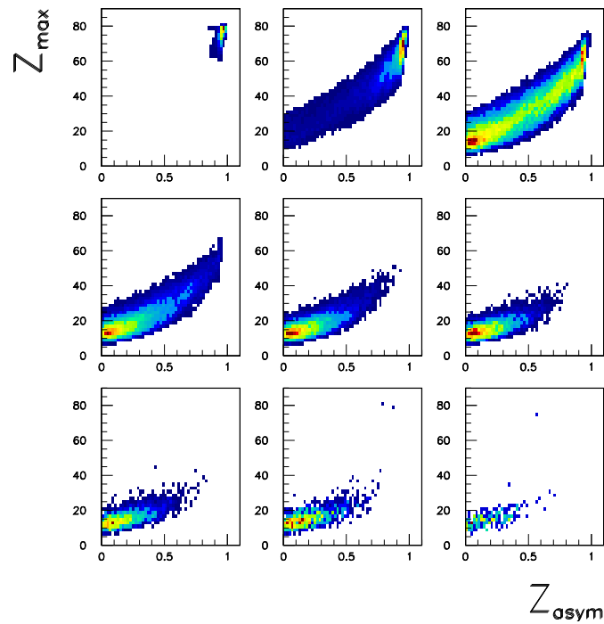
FIG. 3.30 – Au+Au, 60 \text{ MeV}/A : Môme présentation que la figure (3.27).
