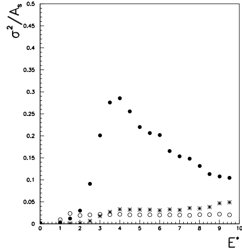
FIG. 5.12 – Au+Au, 80 MeV/A : Représentation de \frac{\sigma^2}{A_s} (exprimé en \text{MeV}^2/A ) en fonction de E^* (en \text{MeV}/A ) pour les différents termes de l'énergie cinétique : les points noirs représentent la partie coulombienne, les étoiles celle due à la masse et les points blancs donnent les fluctuations sur l'énergie d'excitation dans chaque tranche. Cette figure montre que la plus grande partie des fluctuations de E_k vient de la partie coulombienne de l'énergie.
