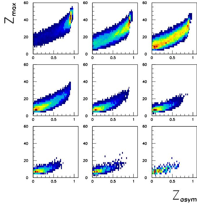
FIG. 3.29 – Xe+Sn, 100 \text{ MeV}/A : Môme présentation que la figure (3.27).
