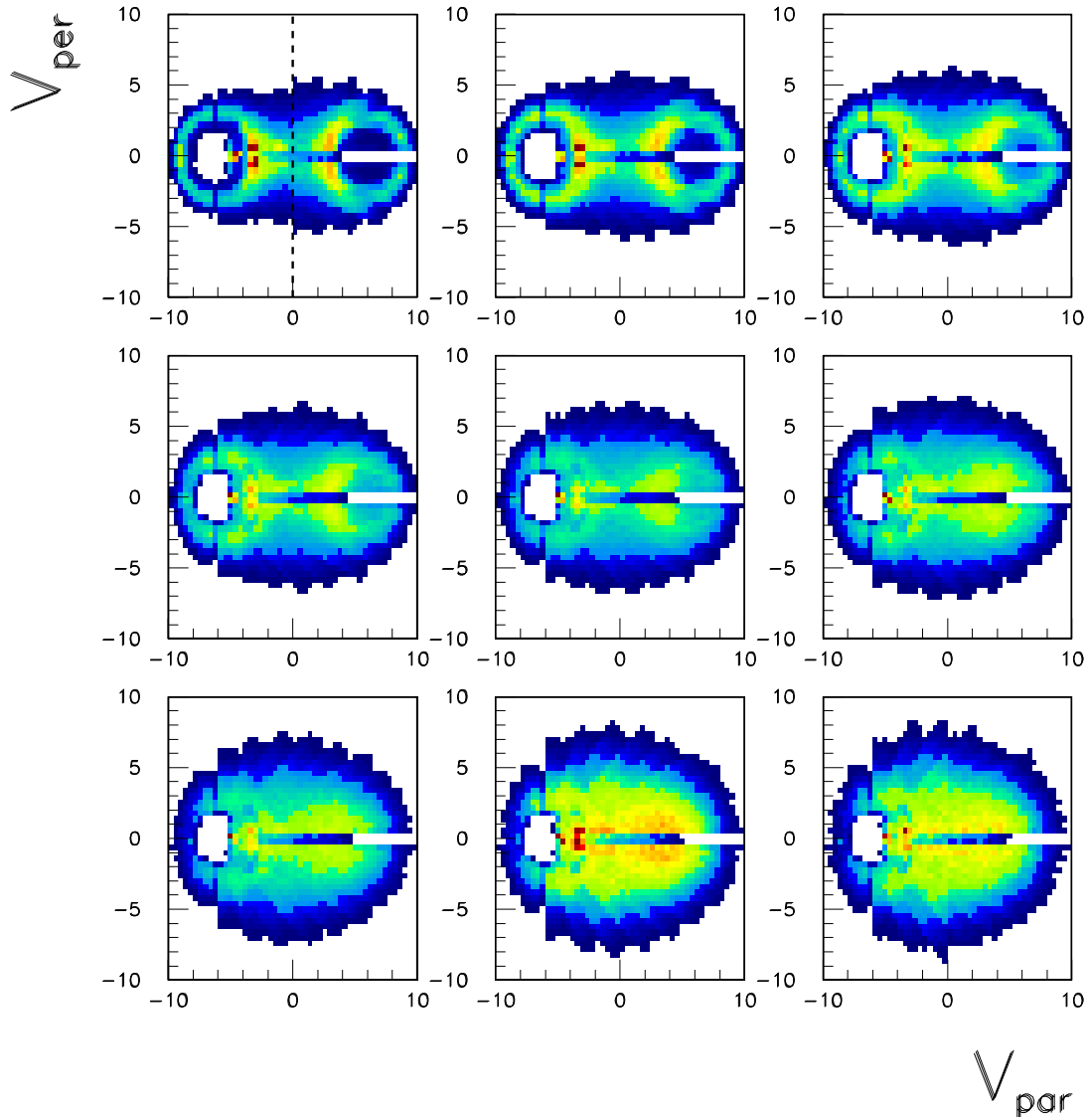
FIG. 3.6 – Xe+Sn , 80 \text{ MeV}/A : Figure représentant la composante V_{par} en fonction de V_{per} des particules alpha dans le repère du centre de masse pour les événements correctement détectés (voir texte plus loin). Les deux composantes sont exprimées en \text{cm/ns} . Chaque graphe correspond à différentes violences de collisions, les premiers étant les moins violentes (tri à l'aide de l'énergie transverse E_{trans} des particules légères à l'arrière du centre de masse de la réaction, grandeur présentée dans le paragraphe 3.3.2). Le centre de masse est repéré par la ligne en pointillé sur le premier graphe. Pour de faibles valeurs de E_{trans} , on distingue nettement deux sources ce qui prouve que les collisions sont binaires.
