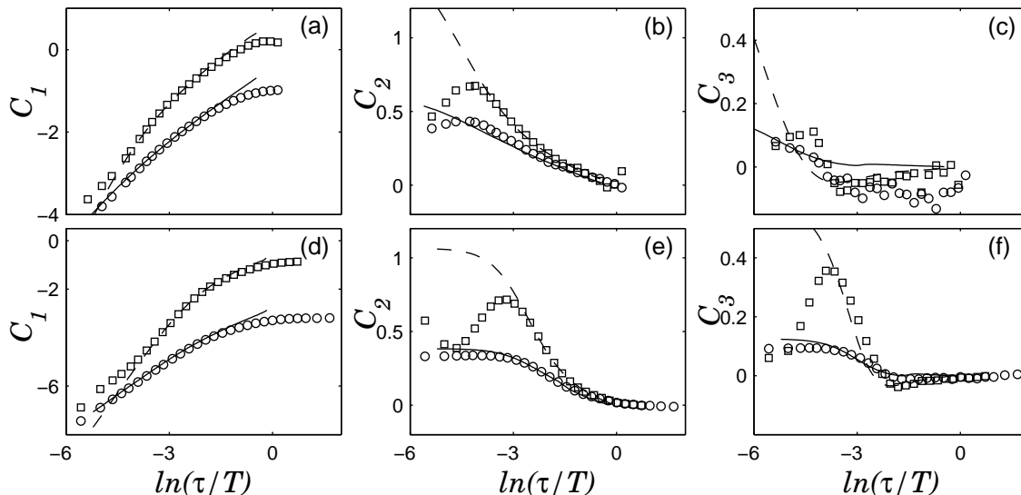
FIG. 5.2 – Représentation des trois premiers cumulants du logarithme C_n = C_{n,\delta_\tau v} - C_{n,\delta_{2\tau} v} des incréments d'ordre 1 ( \delta_\tau^{(1)} v(t) = v(t + \tau) - v(t) ) (o) et d'ordre 2 ( \delta_\tau^{(2)} v(t) = v(t + 2\tau) - 2v(t + \tau) + v(t) ) (□) en fonction de \ln(\tau/T) . Signaux expérimentaux de l'ENS Lyon ( \mathbb{R}_\lambda = 740 ) : (a) C_1 , (b) C_2 et (c) C_3 . Les cumulants théoriques sont obtenus à partir des équations (5.25) et (5.26) pour une ondelette d'ordre N = 1 (traits continus) et d'ordre 2 (traits discontinus), dans un cadre log-normal de paramètres c_2^L = 0.075 et c_1^L = 1/2 + c_2^L = 0.575 , pour un nombre de Reynolds \ln \mathbb{R}_e = 9.24 et pour une valeur du paramètre de transition \gamma = 1.08 (voir texte). Signaux numériques de DNS ( \mathbb{R}_\lambda = 140 ) : (d) C_1 , (e) C_2 et (f) C_3 . Les cumulants théoriques sont obtenus à partir des mêmes équations (5.25) et (5.26), dans un cadre log-normal de paramètres c_2^L = 0.086 et c_1^L = 1/2 + c_2^L = 0.586 , et pour un nombre de Reynolds \ln \mathbb{R}_e = 5.22 et la valeur \gamma = 1.98 .
