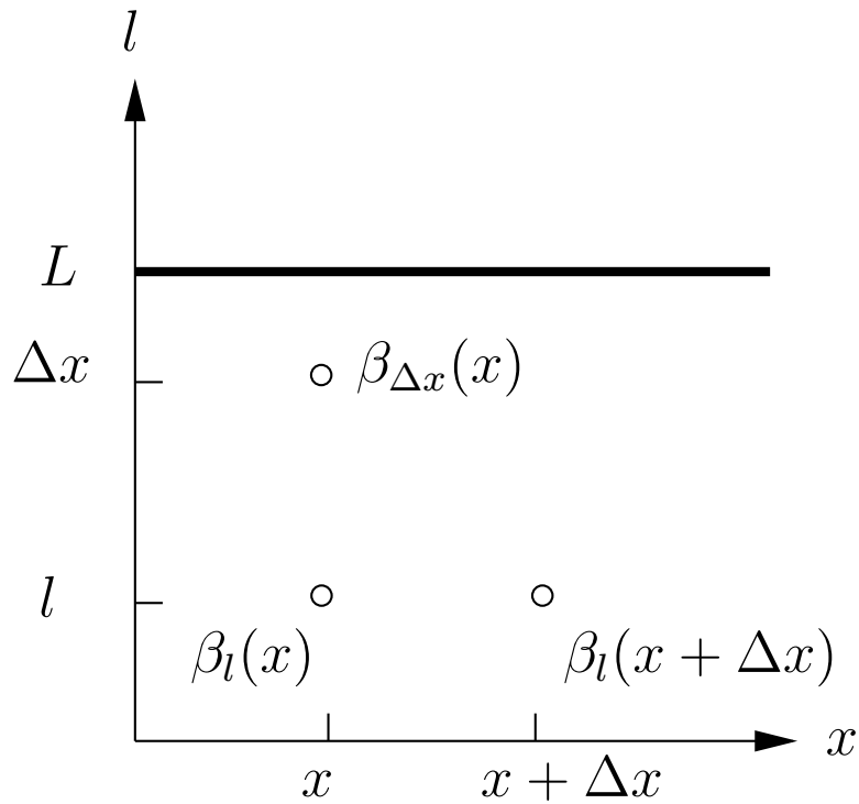
FIG. 8.2 – Représentation du demi-plan espace-échelle (x, l) . Nous indiquons par des ronds (o) les réalisations de la variable \beta_l aux points x et x + \Delta x , ainsi qu'une réalisation de \beta_{\Delta x} au point x .
