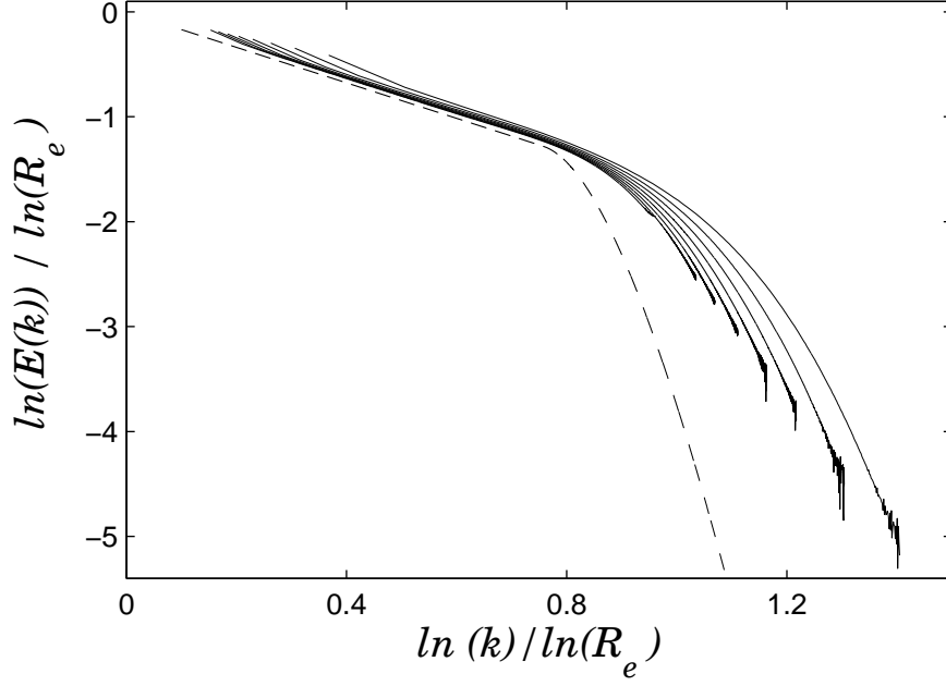
FIG. 3.11 – Représentation du logarithme du spectre de puissance normalisé par le logarithme du nombre de Reynolds, \ln E(k) / \ln \mathbb{R}_e , en fonction de \ln(k) / \ln \mathbb{R}_e . Les traits continus correspondent aux spectres calculés avec notre formalisme dans la figure 3.10. Le trait discontinu correspond à la prédiction asymptotique (Eq. (3.110)) de Frisch et Vergassola [63] à partir de la même forme quadratique (log-normale) du spectre \mathcal{D}^E(h) que celle utilisée dans la figure 3.10.
