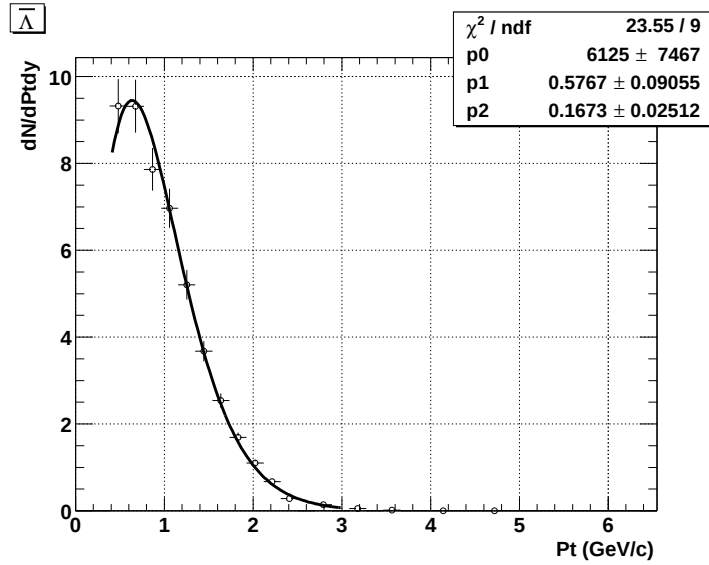
Figure 6.14: Distribution en impulsion transverse des \bar{\Lambda} et ajustement à l'aide du modèle Blast Wave. p_t est l'impulsion transverse des \bar{p} . Les paramètres p0, p1, p2 correspondent respectivement au facteur de normalisation, au flot radial \rho_0 et à la température T.
