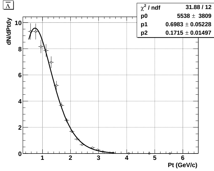
Figure 6.16: Distribution en impulsion transverse des \bar{\Lambda} ( N_{\bar{\Lambda}} ) extraite des données par la collaboration STAR et ajustement avec le modèle Blast Wave. Les paramètres p0, p1, p2 correspondent respectivement au facteur de normalisation, au flot radial \rho_0 et à la température T.
