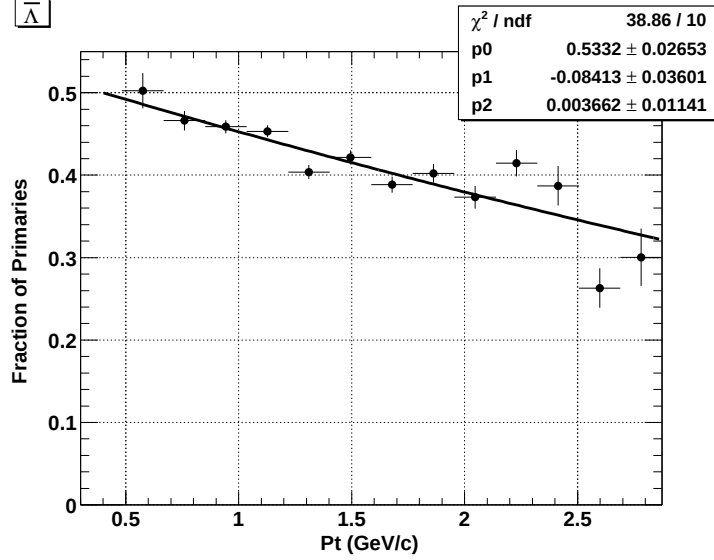
Figure 6.18: La fraction de \bar{\Lambda} primaires P_{\bar{\Lambda}} calculée et ajustée par la fonction : P_{\bar{\Lambda}} = p_2 \times p_t^2 + p_1 \times p_t + p_0 . p_2 , p_1 et p_0 sont des paramètres, p_t est l'impulsion transverse des \bar{\Lambda} .
