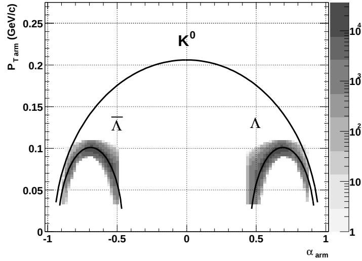
Figure 5.8: Distribution des lambdas et des anti-lambdas sélectionnés en fonction des variables d’Armenteros-Podolski. Les courbes correspondent aux calculs théoriques (voir texte).
