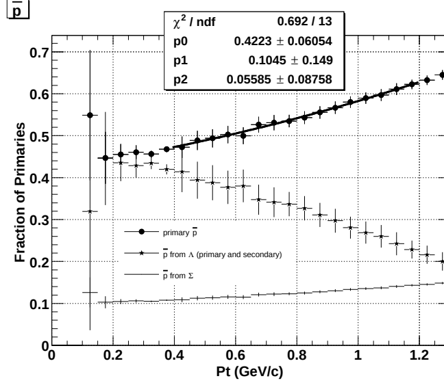
Figure 6.15: Fraction de \bar{p} primaires (points) et ajustement (droite) par la fonction P_{\bar{\Lambda}} = p_2 \times p_t^2 + p_1 \times p_t + p_0 . p_2 , p_1 et p_0 sont des paramètres, p_t est l'impulsion transverse des \bar{p} . Les contaminations dues aux \Lambda (croix) et aux \bar{\Sigma}^- (triangles) sont représentées. La contamination due aux \bar{p} issus de la désintégration des \bar{\Lambda} est dominante.
