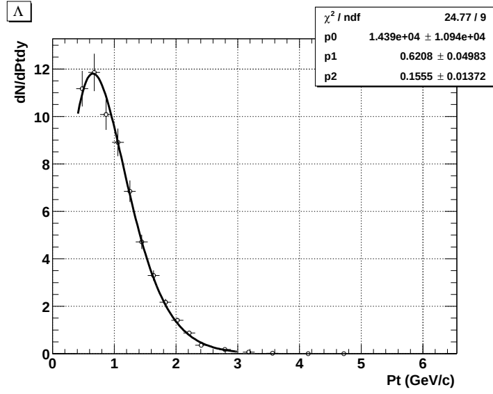
Figure 6.9: Taux de production des \Lambda et ajustement par le modèle Blast Wave. p_t est l'impulsion transverse des protons. Les paramètres p_0 , p_1 , p_2 correspondent respectivement au facteur de normalisation, au flot radial \rho_0 et à la température T .
