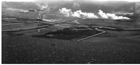
Photo I.1 : Site d'exploitation géothermale du Krafla (Islande). Photo : A. Finizola.
