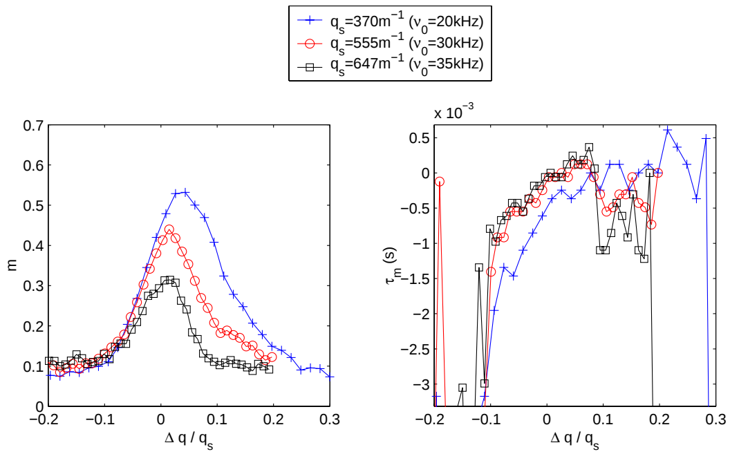
FIG. 3.13 – Taux de corrélation m et retard \tau_m des modules autour de modes de Fourier croissants. série CASCADE : bvps7-20k;30k et 35k
