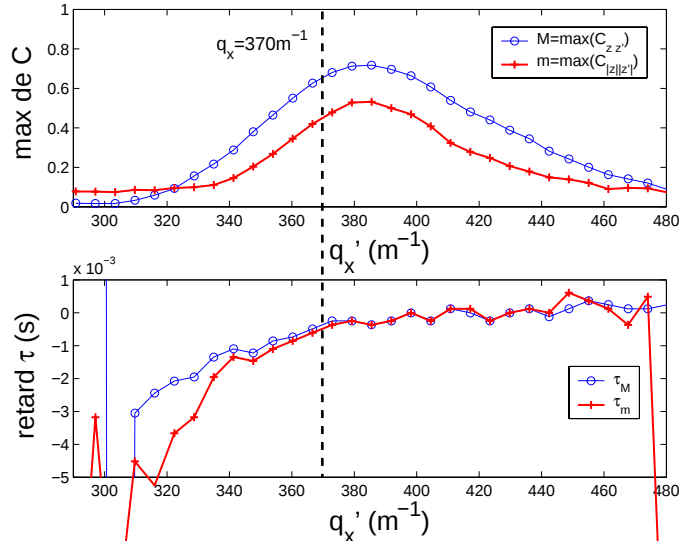
FIG. 3.4 – Evolution, tirée de FIG. 3.3, du maximum d’intercorrélacion des complexes et des modules (en haut) et du retard entre les deux voies (en bas). L’accord est atteint lorsque la voie 2 émet à \nu'_0 = 30.5 \text{ kHz} (au lieu des 29.4 \text{ kHz} théoriques prévus).
