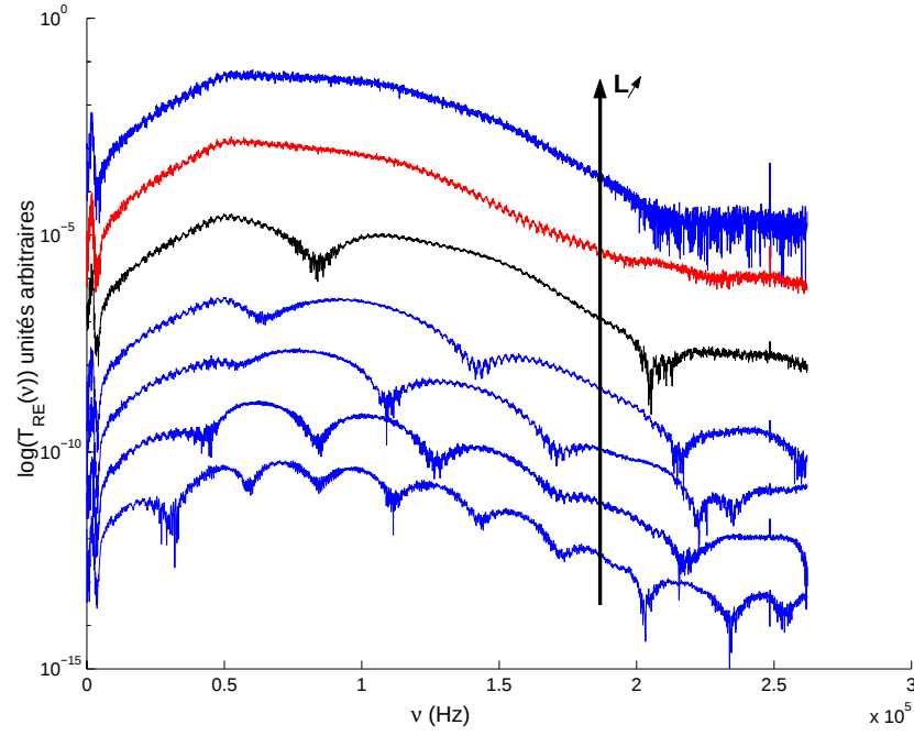
FIG. 1.16 – Fonction de transfert T_{RE} sur l'axe, pour différentes tailles de cavité entre L = 20 et L = 170\text{cm} . Les courbes ont été volontairement traduites pour plus de clarté, spectres sur 8192 points.
