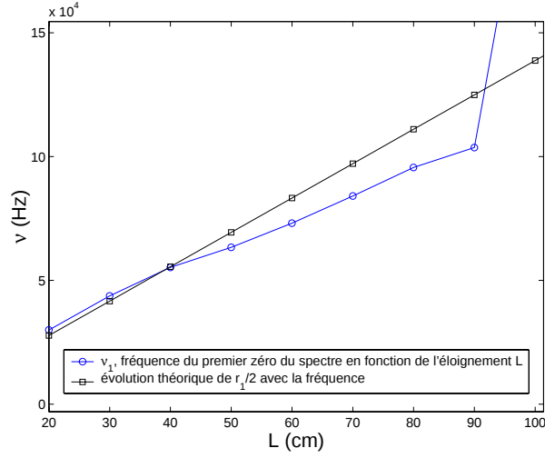
FIG. 1.18 – Fréquence de la première extinction \nu_1 de la fonction de transfert en fonction de l'éloignement.
