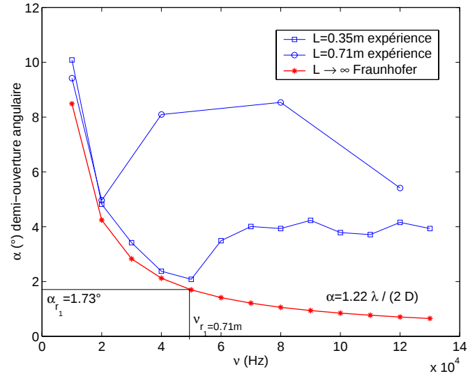
FIG. 1.26 – Demi-ouverture angulaire \alpha en fonction de la fréquence d'émission \nu . D = 0.14 m
