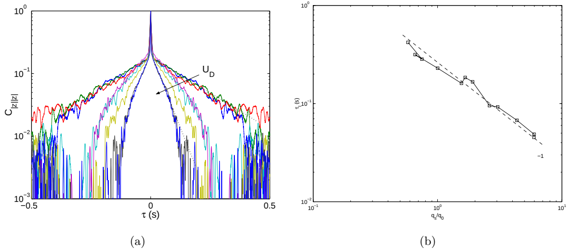
FIG. 2.12 – (a) Autocorrélations obtenues pour différentes vitesses de la soufflerie. (b) Evolution du temps long de décorrélation en fonction de U_D . Série UVARIE
