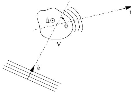
FIG. 1.1 – Configuration-type d’une expérience de diffusion acoustique : une onde plane, de fréquence \nu_0 rencontre une distribution de vorticit  contenue dans un volume V . Celle-ci interagit avec l’onde incidente en  mettant une onde diffus e qui sera d tect e sous un angle \theta .
