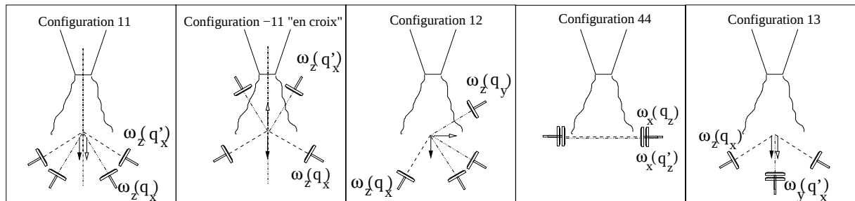
FIG. 3.1 – D finition et appellations des configurations g om triques utilis es pour l'interf rom trie utilisant deux voies de mesures.
