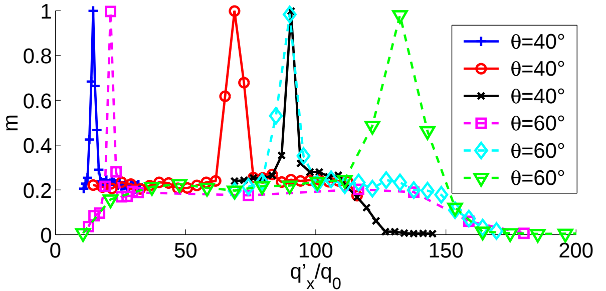
FIG. 3.19 – Maximum de corrélation m dans deux configurations géométriques et pour différentes valeurs du mode fixe q_x .
