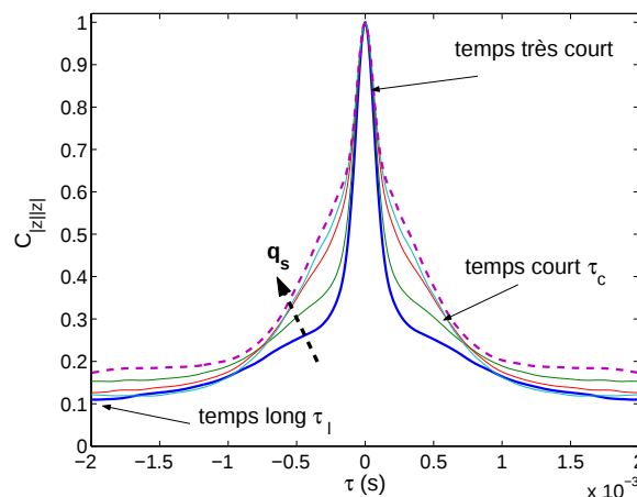
FIG. 2.19 – Vue agrandie aux temps courts de 5 autocorr lations successives du CERN pour le R_\lambda = 3450 . A mesure que l'on augmente le nombre d'onde, on constate l'importance progressive du temps court \tau_c analogue au temps court du LEGI, prenant le pas sur la partie aux temps tr s courts. manip CP114 q_s/q_0 \in [58 - 79]
