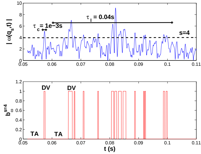
FIG. 4.8 – Principe du seuillage-binarisation opéré sur le module du signal (normalisé par son écart-type). Le signal binaire b_\omega^s définit les variables aléatoires DV et TA de durée de vie et de temps d'attente, ici pour le seuil s = 4 . Fichier extrait de la série QMONOI-40 pour q_s/q_0 = 70
