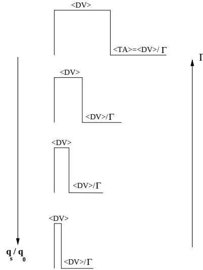
FIG. 4.18 – Effet de l'intermittence (caractérisée par le facteur d'intermittence \Gamma ) : déformation à haut Reynolds du motif élémentaire moyen à travers les échelles. \langle DV \rangle et \langle TA \rangle décroissent simultanément mais avec des lois d'échelles différentes : à l'échelle du motif moyen, le temps d'attente entre deux événements s'allonge.
