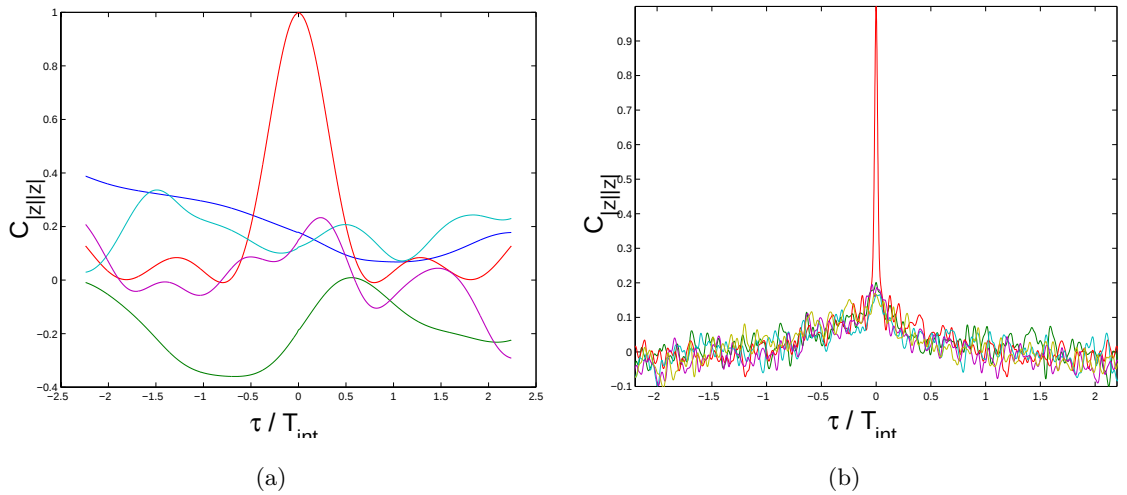
FIG. A.7 – Cor relation crois e entre : (a)le nombre d'onde q=3 et les 5 nombres d'onde dans son voisinage imm diat (b)le nombre d'onde q=70 et les 5 nombres d'onde dans son voisinage imm diat
