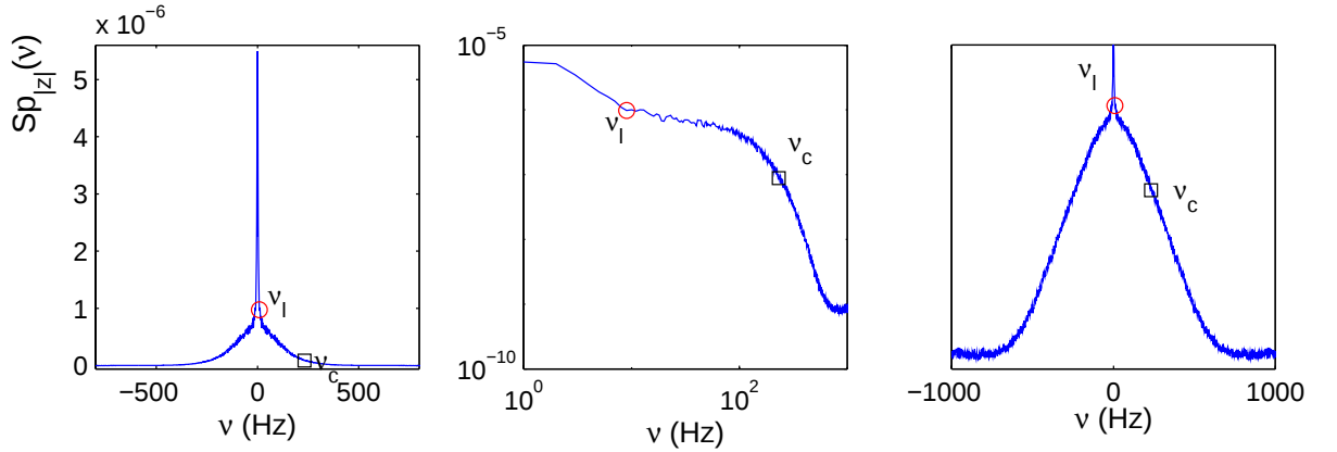
FIG. 2.8 – Exemple type d’un spectre du module Sp_{|z|} , repr sent  successivement en coordonn es lin-lin, log-log et enfin log-lin. Spectre calcul  sur 4096 points   partir d’un fichier de 1Mpts. Fichier extrait de la s rie UVARIE pour U_D \approx 4.3 \text{ m.s}^{-1} . Les symboles \circ et \square correspondent   la figure 2.9
