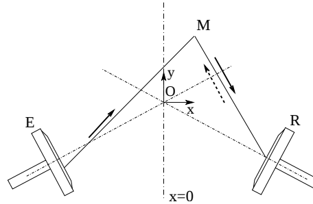
FIG. 1.40 – Configuration du calcul numérique du champ acoustique U en tout point M
