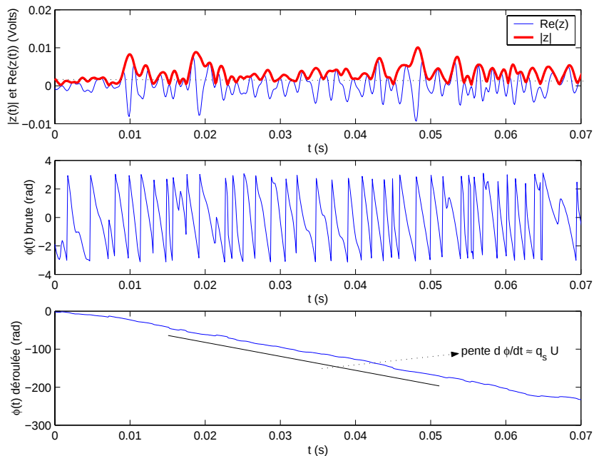
FIG. 1.5 – Signaux de diffusion par la vorticit   issus de mesures sur une soufflerie    air de diam  tre d = 20 mm, d  livrant un jet de vitesse    la buse \approx 100 m.s -1 . En haut et en gras figure le module du signal complexe. Au centre, la phase (brute) oscille entre -\pi et \pi . En bas, l'op  ration de d  roulage de cette phase souligne la d  croissance continue de la phase, dont la pente moyenne permet le calcul de la vitesse Doppler moyenne.
