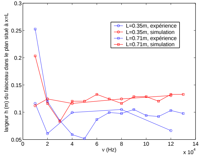
FIG. 1.25 – Evolution de la largeur à mi-hauteur de la figure de diffraction dans les plans L = 0,35 m et L = 0,71 m pour les expériences et les simulations.
