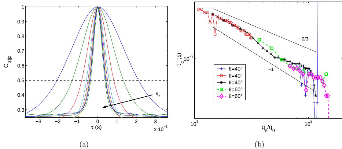
FIG. 2.15 – (a) Autocorrélations typiques (détail des temps courts) pour des nombres d'onde croissants entre q_s/q_0 = 15 et 100 - correspond aux symboles * de la figure de droite. (b) Evolution de \tau_c en fonction du nombre d'onde adimensionné q_s/q_0 . Série QMONOI-40 et QMONOI-60
