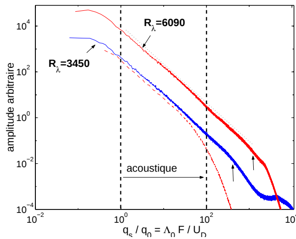
FIG. 2.7 – CERN : Spectres (loglog) de vitesse longitudinale u_x issus des mesures par fil chaud supra-conducteur pour les deux débit d'Hélium extrêmes : Q_m = 82 et 250 \text{ g/s} . \Lambda_0 = 0.11 \text{ m}
