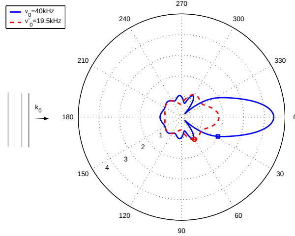
FIG. 1.29 – Diagrammes de rayonnement ( |f| , en linéaire) pour une bille de rayon R = 8 mm et deux fréquences d'émission ( \nu_0 = 40 et 19,5 kHz) ; correspondant à q_s R = 2.8 pour les deux configurations étudiées (symboles \square : \theta = 28^\circ et \circ : \theta' = 60^\circ ).
