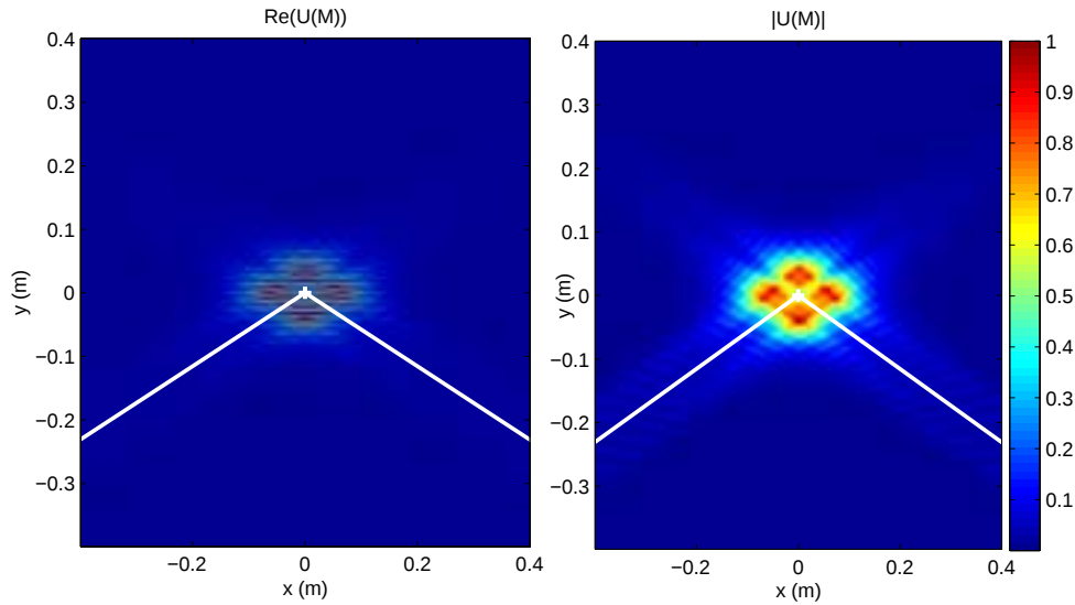
FIG. 1.41 – Simulation numérique du champ U(M) produit par le couple émetteur-récepteur en configuration de diffusion avec, à droite le module du champ (échelle de couleurs linéaire) image de la sensibilité s(x, y) du volume de mesure en tous points. À gauche la phase du champ est représentée plus explicitement par la partie réelle de U(M) . \theta = 60^\circ , \nu_0 = 100 kHz, D = 0,14 m et L = 0,71 m ( r_1 = 2L ). Grille de 800 \times 800 points pour une résolution de 1 mm
