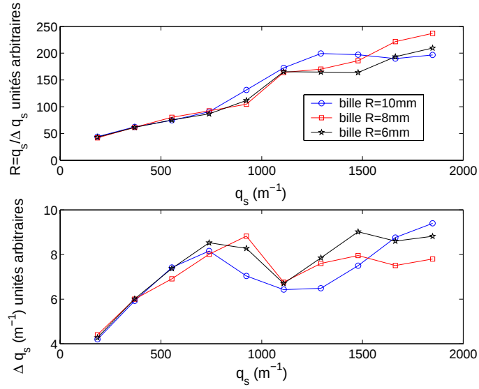
FIG. 1.39 – Variations de la résolution R et de l'incertitude \delta q en fonction de \mathbf{q_s} dans la configuration de la voie 2 ( \theta' = 60^\circ , L = 0.71 m) pour les trois billes.
