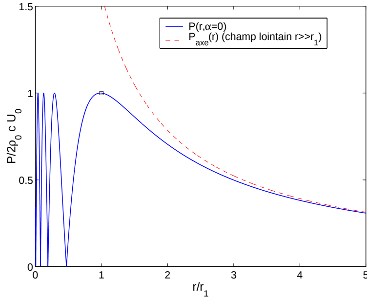
FIG. 1.13 – Amplitude de la pression sur l'axe P(r, 0) (formule 1.12) en fonction de l'éloignement adimensionné par r_1 . En tirets, tendance asymptotique de la pression en champ lointain P_{axe}(r) (formule 1.11). Calcul réalisé pour un piston de diamètre D = 14\text{cm} émettant à \nu_0 = 20\text{kHz}
