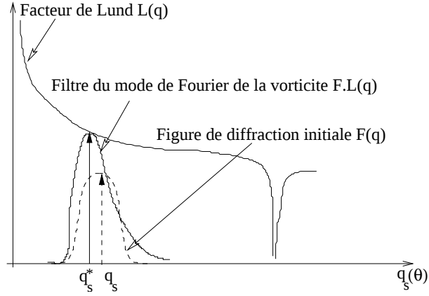
FIG. 1.50 – Déformation attendue de la figure de diffraction par le facteur de Lund \mathcal{L}(\theta) dans le cas de la diffusion de la vorticité. On a supposé un filtre d'échelle \mathcal{F} initialement symétrique, visant le mode q_s = 4\pi\nu_0 \sin(\theta/2)/c . En réalité, on vise un mode q_s^* plus petit, avec un filtre \mathcal{L}.\mathcal{F} asymétrique.
