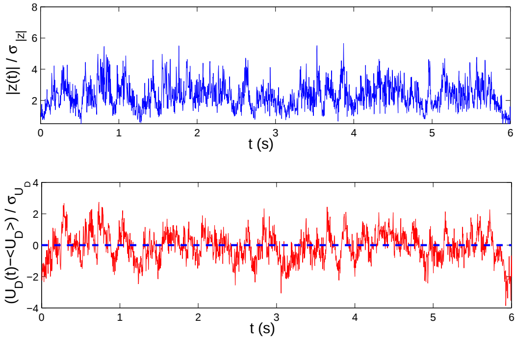
FIG. 2.37 – Comparaison entre en haut le module du signal de diffusion et en bas la vitesse issue de la WVRID pour le même fichier que FIG. 2.33.
