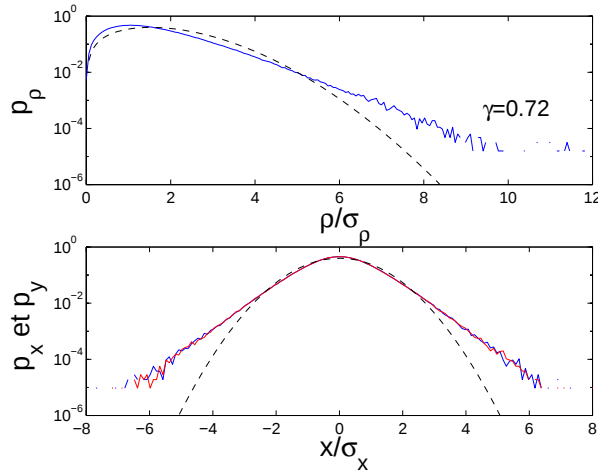
FIG. 4.1 – pdf du module de la vortacité (en haut) et des parties réelles et imaginaires (en bas). Calcul sur 200 classes, pour q_s = 2310\text{m}^{-1} , manip QMONOI-60 fichier de 32s (1Mpts)
