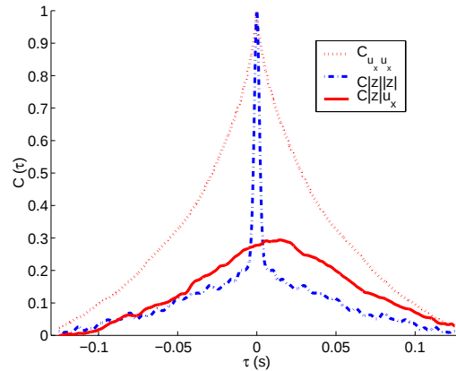
FIG. 2.41 – Autocor lation du signal u_x , de |z| et intercor lation entre le module et la vitesse u_x
