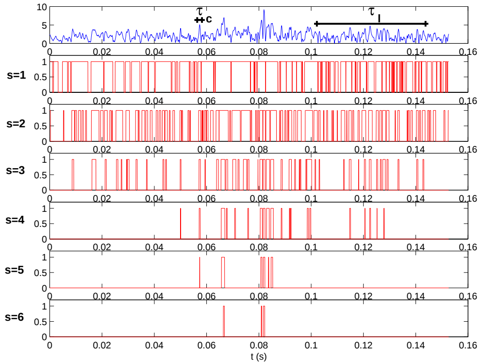
FIG. 4.8 – Principe du seuillage-binarisation opéré sur le module du signal (normalisé par son écart-type). Le signal binaire b_\omega^s définit les variables aléatoires DV et TA de durée de vie et de temps d'attente, ici pour le seuil s = 4 . Fichier extrait de la série QMONOI-40 pour q_s/q_0 = 70
