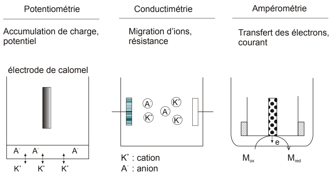
Figure 1.5. Détection électrochimique
