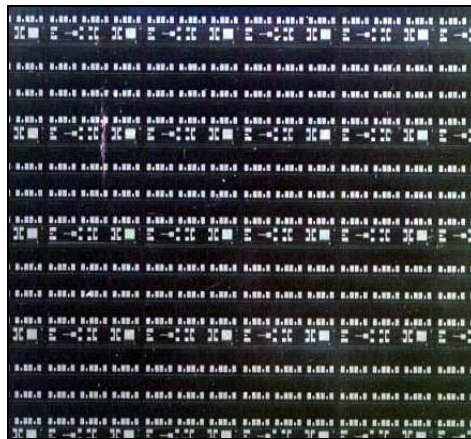
Figure 2.28. ISFETs en wafer
