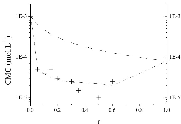
FIG. 1.18: Evolution de la CMC du système CTAOH-C13COOH en fonction du rapport molaire r. La courbe en pointillés large correspond au modèle d'un mélange idéal. Celle en pointillés fin correspond au modèle de Rubingh et Holland pour un coefficient d'interaction de -10 k_B T
