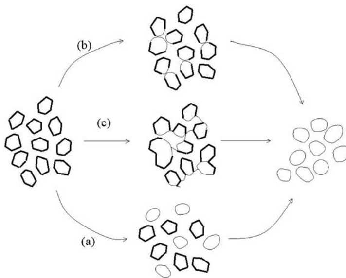
FIG. 3.28: Proposition de phases intermédiaires
