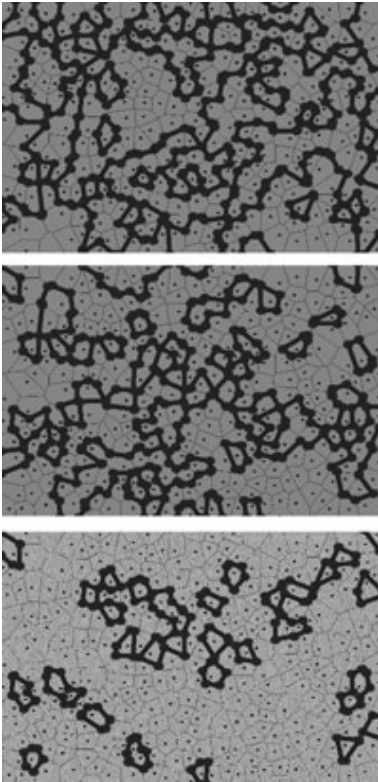
FIG. 3.30: Transition régulière d'une phase éponge (haut) à une suspension de vésicules (bas) en diminuant le nombre de connexions dans le cas d'un modèle à 2 dimensions[167]
