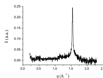
FIG. 5.18: Mise en évidence du réseau hexagonal des chaînes par diffusion de rayons X
