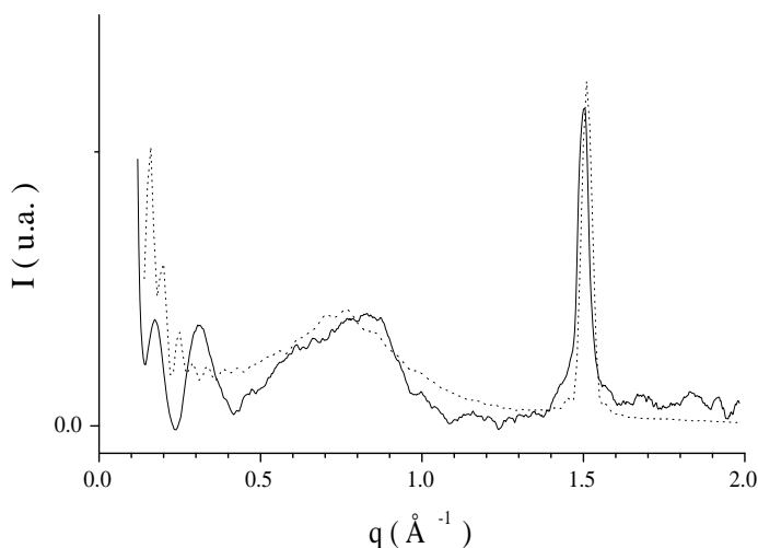
FIG. 4.23: Comparaison de la courbe expérimentale (trait continu) obtenue pour un échantillon ( r=0.55 ; C=13\% ) et de la courbe déduite de la simulation de Monte Carlo (trait pointillé) pour r=0.55 , \alpha=0.82 , R=1.5\text{\AA} et h=21.5\text{\AA} . La distance entre premiers voisins est adaptée au pic de diffraction q_{100} . On remarque la différence entre les positions du maximum de la bosse diffuse pour l'expérience et le calcul.
