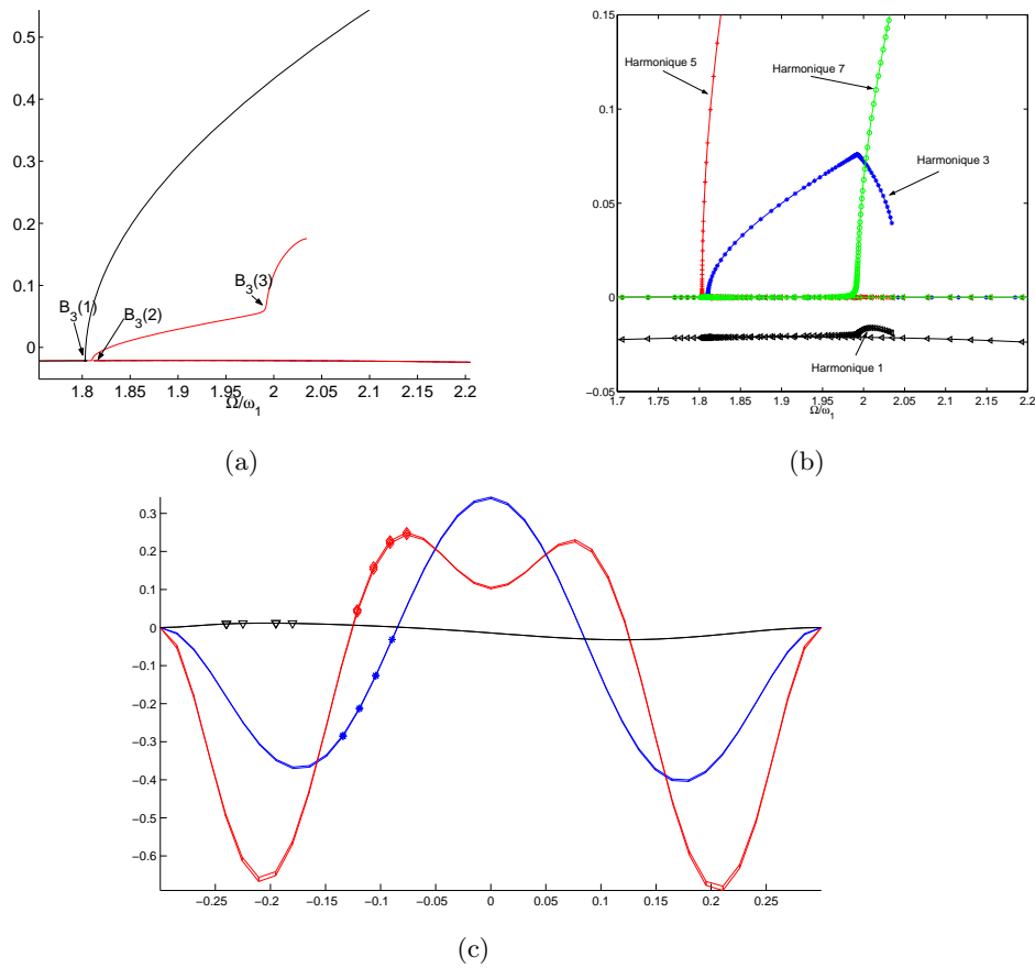
FIGURE V.9 - Réponse forcée de la poutre bi-encastrée dans la zone B_3 de la figure V.8 - (a) q_0/h - (b) Harmoniques : q^1/h ( \triangleright ), q^3/h (*), q^5/h (+) et q^7/h (o) (les autres étant nulles) - (c) Déformées correspondantes pour \Omega < 330 rad/s ( \nabla ), 330 < \Omega < 362 rad/s (*) et \Omega > 362 rad/s, ( \diamond ).
