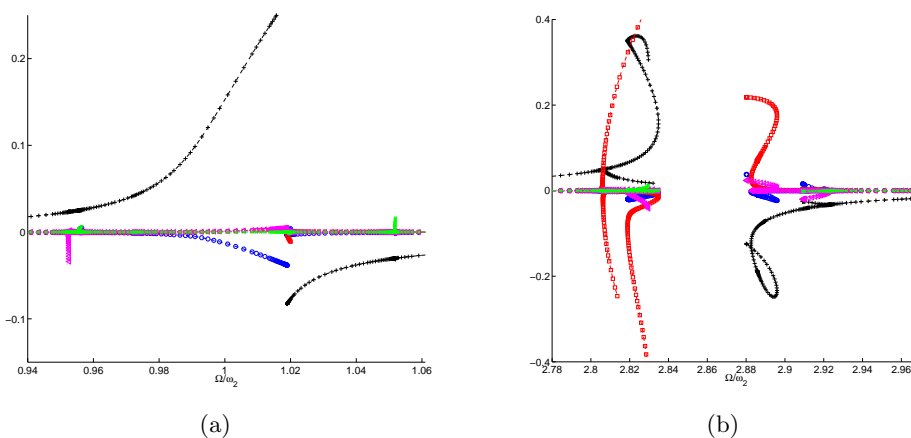
FIGURE V.23 - Réponse forcée du gong, harmoniques, (bleu, o) : q^0/h , (noir, +) : q^1/h , (rouge, \square ) : q^2/h , (magenta, \triangle ) : q^3/h , (vert, \times ) : q^4/h - (a) À proximité de \omega_1 - (b) Vers \omega_2
