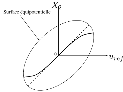
FIGURE I.2 - Approche Rosenberg, ligne modale pour un système à deux degrés de liberté, u_2 = X_2(u_{ref}) : courbes passant par l'origine et finissant sur les surfaces équipotentielles pour un niveau d'énergie fixé. - - cas linéaire, — cas non linéaire.
