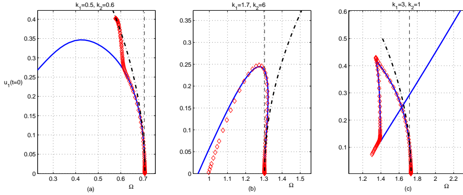
FIGURE I.8 - Premier mode du système à deux ressorts. (...) : mode linéaire, traits pleins : EHMAN, (-.-) : TOUZÉ et al. (2003), \diamond continuation des orbites périodiques. (a) : \omega_{01} = \sqrt{0.5} , \omega_{02} = \sqrt{6} , (b) : \omega_{01} = \sqrt{1.7} , \omega_{02} = \sqrt{6} , (c) : \omega_{01} = \sqrt{3} , \omega_{02} = 1 ,
