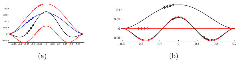
FIGURE V.4 - Réponse libre de la poutre bi-encastée autour de \omega_1 - Déformées relevées pour diverses valeurs de la fréquence, en A, B, F et G (voir les points sur la figure V.3), pour H=8 - (a) q_0/h en A(□), B(+), F(◁) et G(o)- (b) q^1/h en F (o) et q^5/h en F (□) et G (×) .
