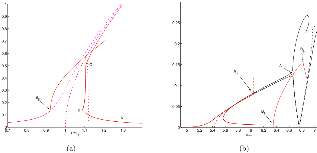
FIGURE V.10 - Réponse forcée de la poutre bi-encastree. |\frac{q_0}{h}| en fonction de la pulsation d'excitation, à proximité des modes (a) : 1 (b) : 3. (- -) : mode non linéaire, (-) réponse forcée pour H=6 ou 8 , (-.-), réponse forcée pour H=4
