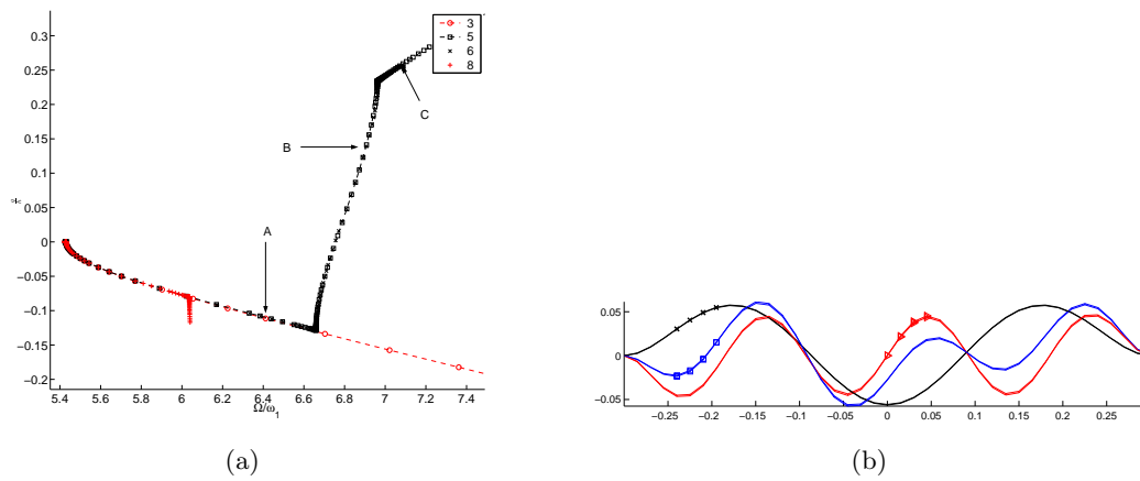
FIGURE V.7 - Réponse libre de la poutre bi-encastree à proximité de \omega_3 - (a) q_0/h à proximité de \omega_3 pour H=3,5,6,8 (b) Déformées pour H=6 en A ( \times ), B ( \triangleleft ) et C ( \square ).
