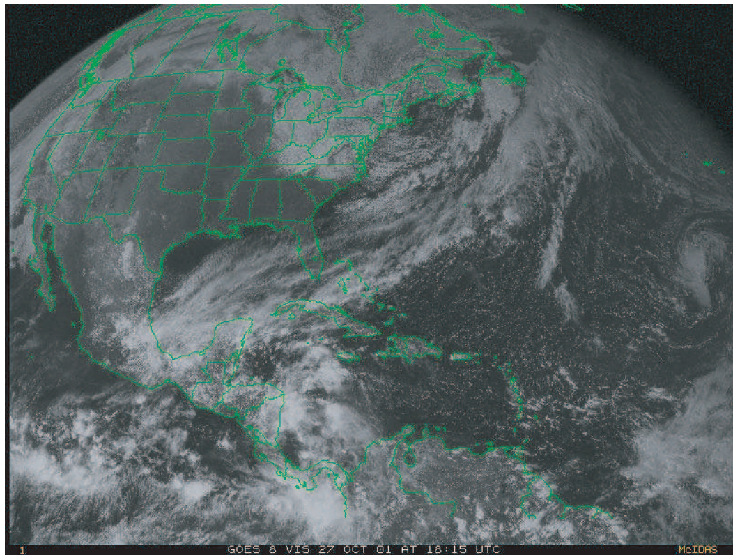
Figure n°108 : Analyse de la photo satellite du 27/10/2001, GOES 8, est, vis, 18h15 T.U (D'après carte de la NOAA, "Tropical surface analysis, Atlantic", 18h00 T.U) (D'après carte de la GEIC, "Systemas principales", 11h45 heure locale)
