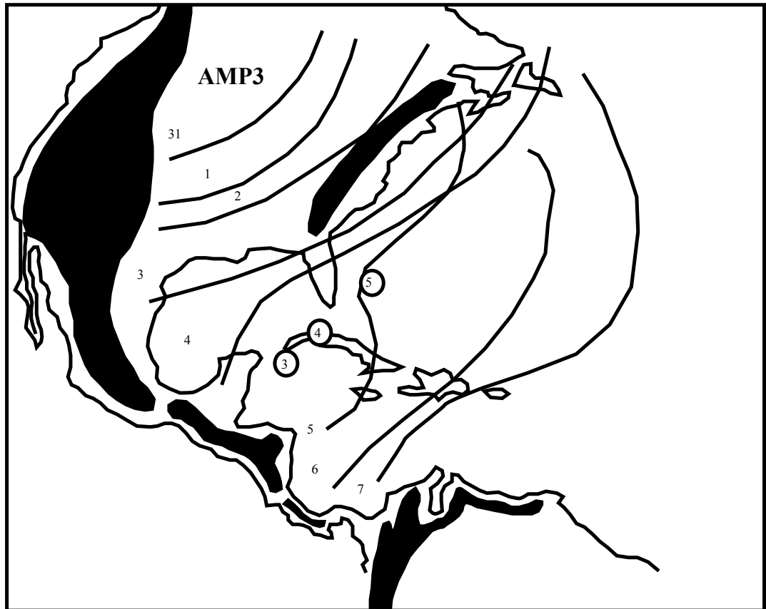
Fig. n°121 : Carte récapitulative de l'évolution de surface de l'AMP3, trajectoire de "Michelle" du 31 octobre au 7 novembre 2001
