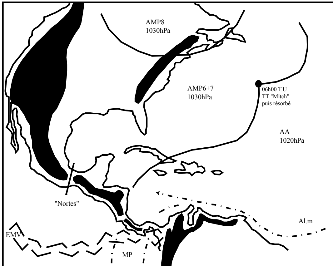
Figure n°139 : Analyse de la photo satellite du 7/11/1998, GOES 8, est, vis, 18h15 T.U
