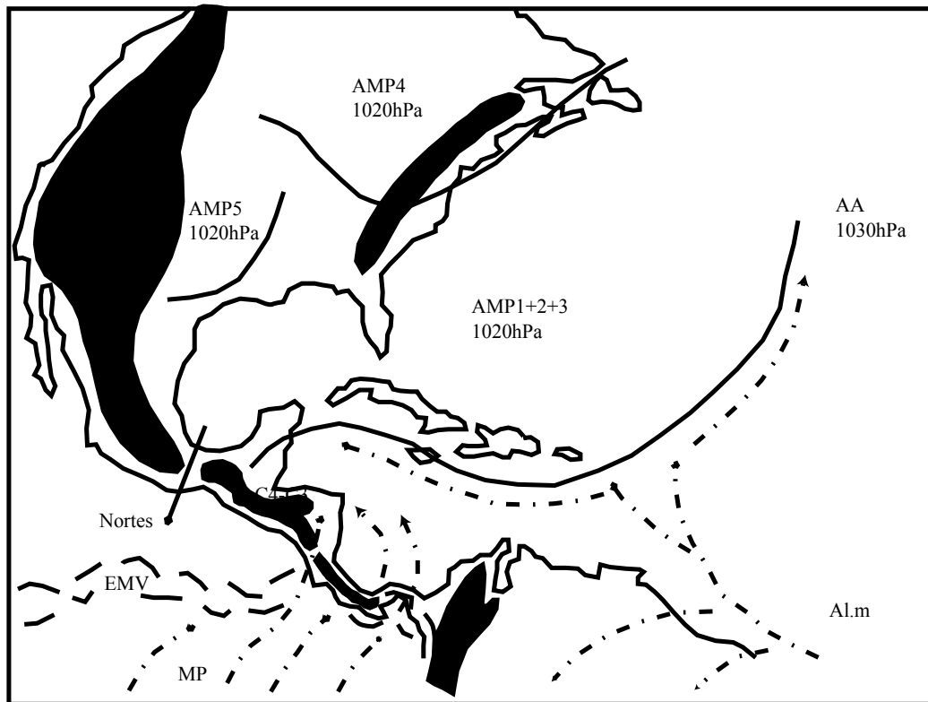
Figure n°129 : Analyse de la photo satellite du 28/10/1998, GOES 8, est, vis, 18h15 T.U
