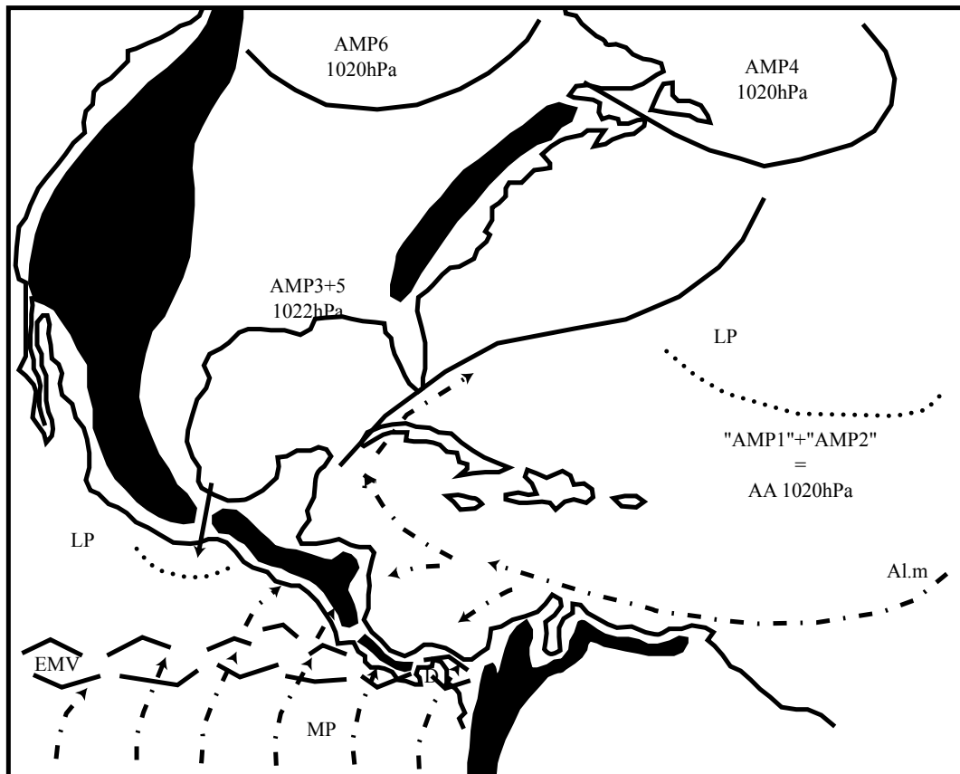
Figure n°79 : Analyse de la photo satellite du 29/5/2003, GOES 8, est, vis, 18h15 T.U (D'après carte de la NOAA, "Tropical surface analysis, Atlantic", 18h00 T.U) (D'après carte de la GEIC, "Systemas principales", 11h45 heure locale)
