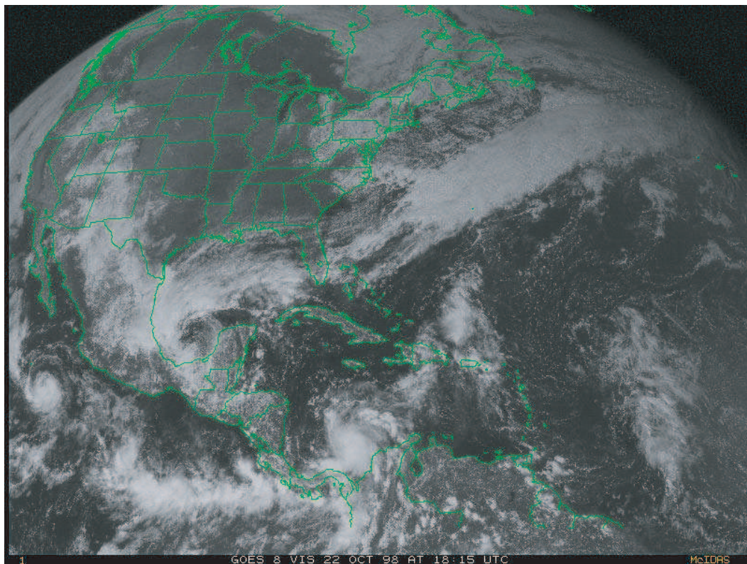
Figure n°123 : Analyse de la photo satellite du 22/10/1998, GOES 8, est, vis, 18h15 T.U (D'après carte de la NOAA, "Tropical surface analysis, Atlantic", 18h00 T.U) (D'après carte de la GEIC, "Systemas principales", 11h45 heure locale)
