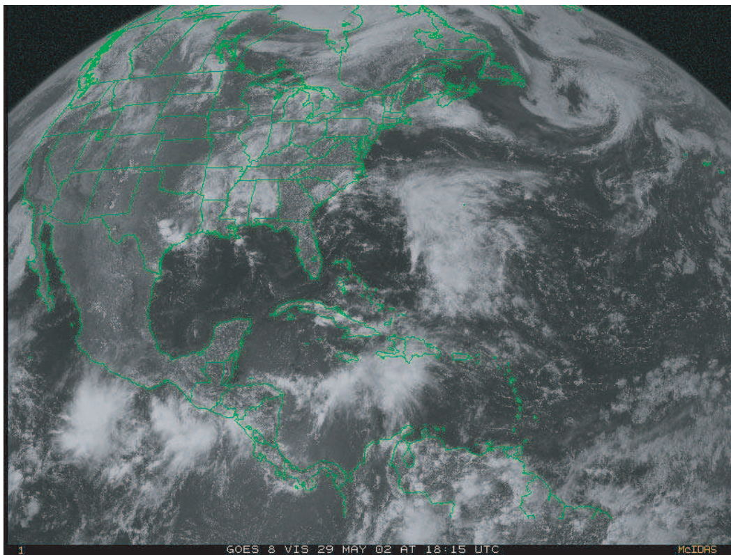
Figure n°72 : Analyse de la photo satellite du 29/5/2002, GOES 8, est, vis, 18h15 T.U
