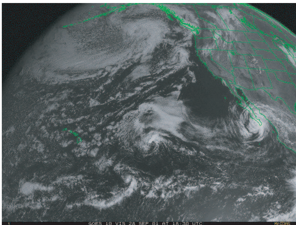
Photo satellite n°164 : GOES 10, ouest, vis, le 28/9/2001, 18h30 T.U
