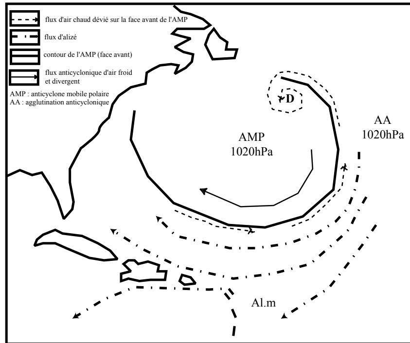
Figure n°16 : Analyse de la photo satellite du 13/12/1999 (D'après carte de la NOAA, "Tropical surface analysis, Atlantic", 18h00 T.U)
