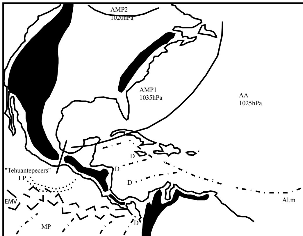
Figure n°108 : Analyse de la photo satellite du 27/10/2001, GOES 8, est, vis, 18h15 T.U (D'après carte de la NOAA, "Tropical surface analysis, Atlantic", 18h00 T.U) (D'après carte de la GEIC, "Systemas principales", 11h45 heure locale)
