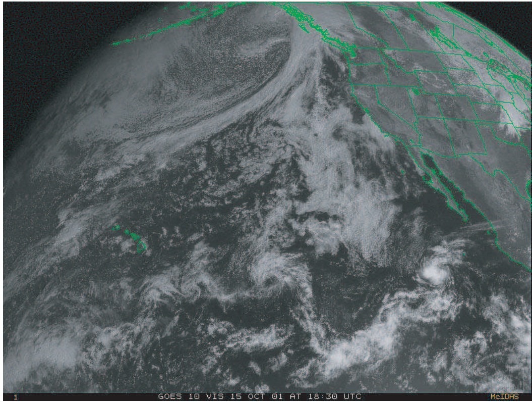
Figure n°190 : Analyse de la photo satellite du 15/10/2001, GOES 10, ouest, vis, 18h30 T.U
