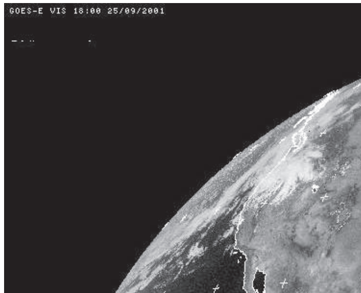
(GOES 10, est, vis, le 25/9/2001, 18h00 T.U)
