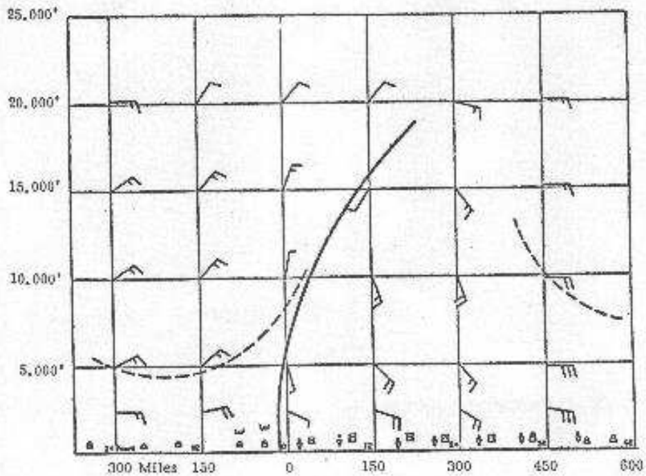
Fig. n° 24 : Modèle d'une « onde d'est » ; coupe verticale le long du segment A-B sur la figure précédentes (Riehl, 1954)
