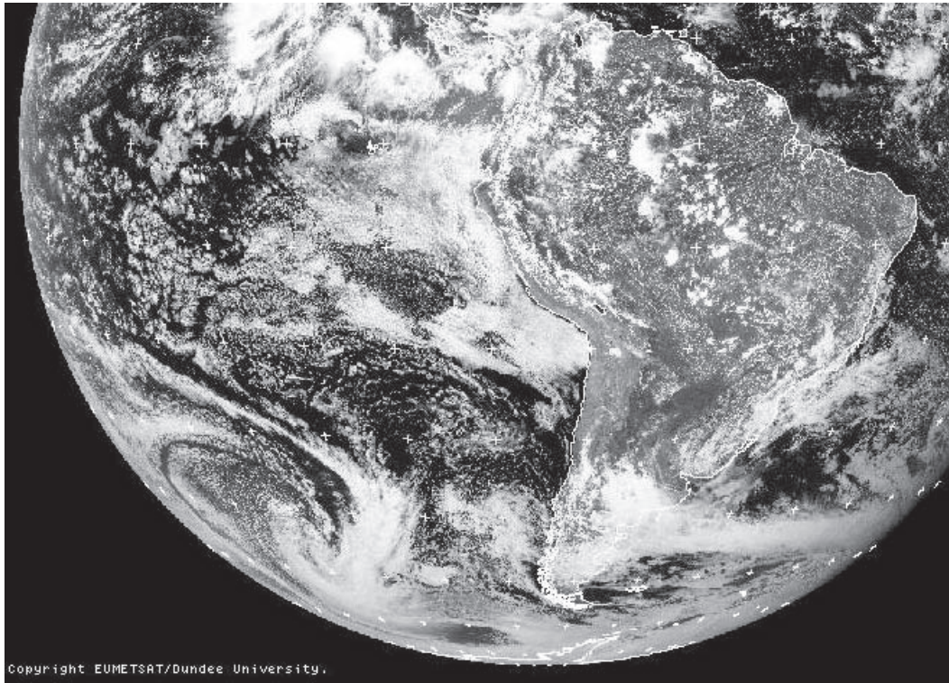
Figure n°15(B) : Analyse de la photo satellite du 23/9/2001 (D'après carte de la NOAA, "Weather pub fax", 18h00 T.U)
