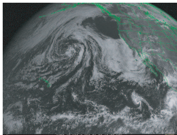
Photo satellite n°171 : GOES 10, ouest, vis, le 3/10/2001, 18h30 T.U
