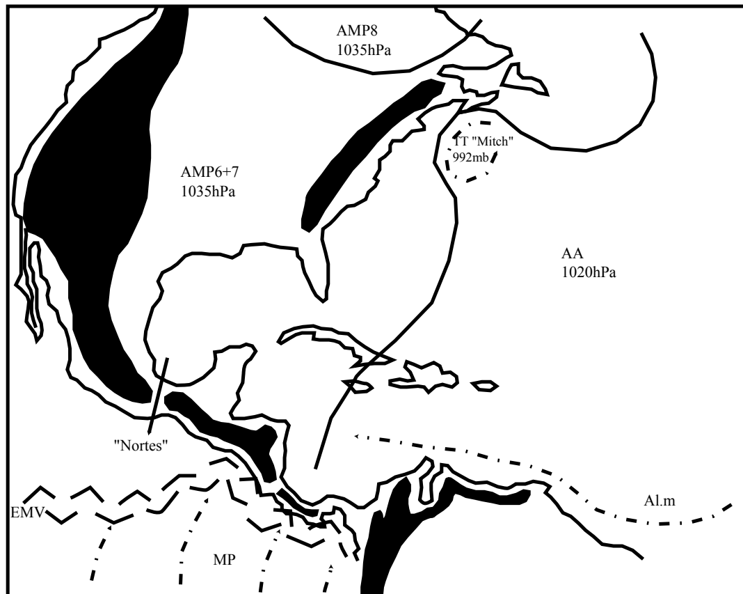
Figure n°138 : Analyse de la photo satellite du 6/11/1998, GOES 8, est, ir, 12h15 T.U (D'après carte de la NOAA, "Tropical surface analysis, Atlantic", 18h00 T.U) (D'après carte de la GEIC, "Systemas principales", 11h45 heure locale)
