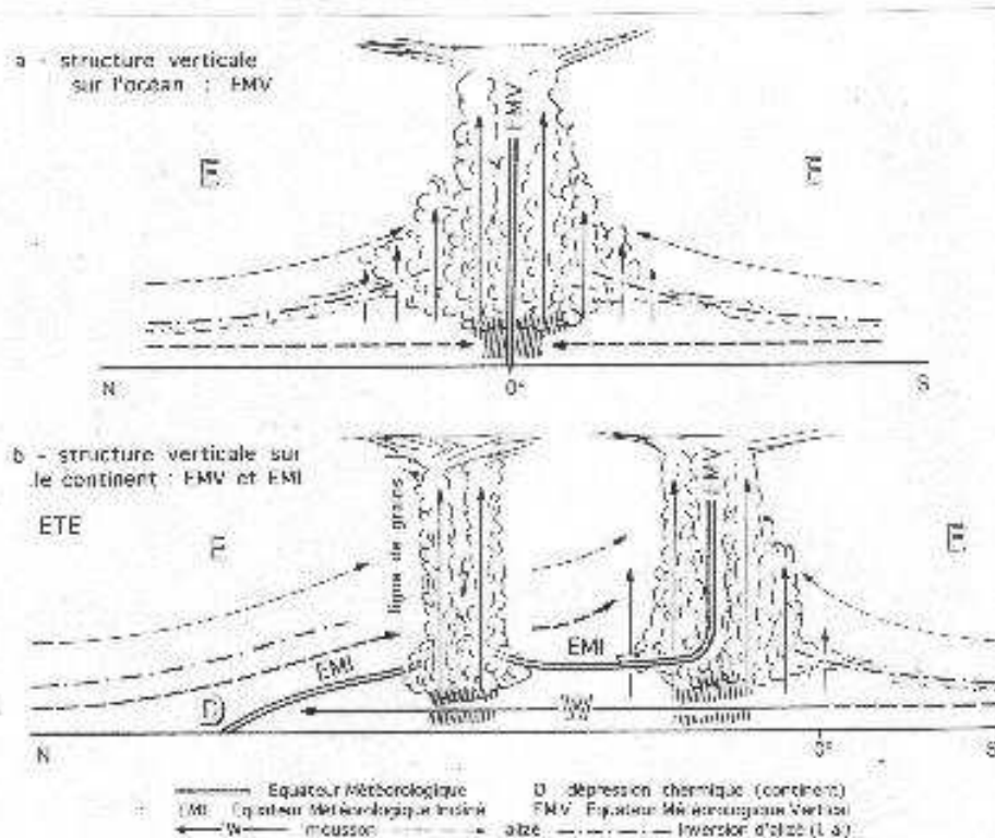
Fig. n°20 : « Structure verticale de l'équateur météorologique : a – océan, b – continent (M. Leroux, 2000)
