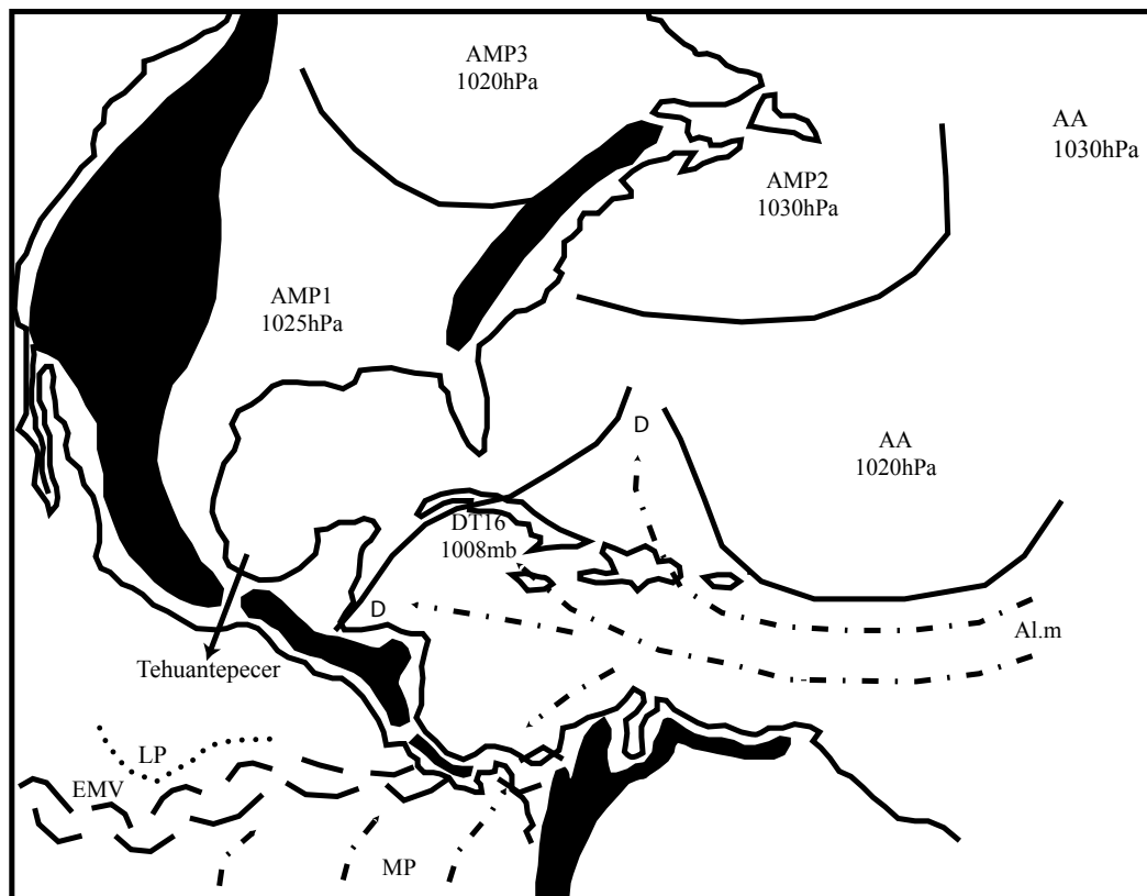
Figure n°142 : Analyse de la photo satellite du 12/11/1999, GOES 8, est, vis, 18h15 T.U (D'après carte de la NOAA, "Tropical surface analysis, Atlantic", 18h00 T.U) (D'après carte de la GEIC, "Sistemas principales", 11h45 heure locale)
