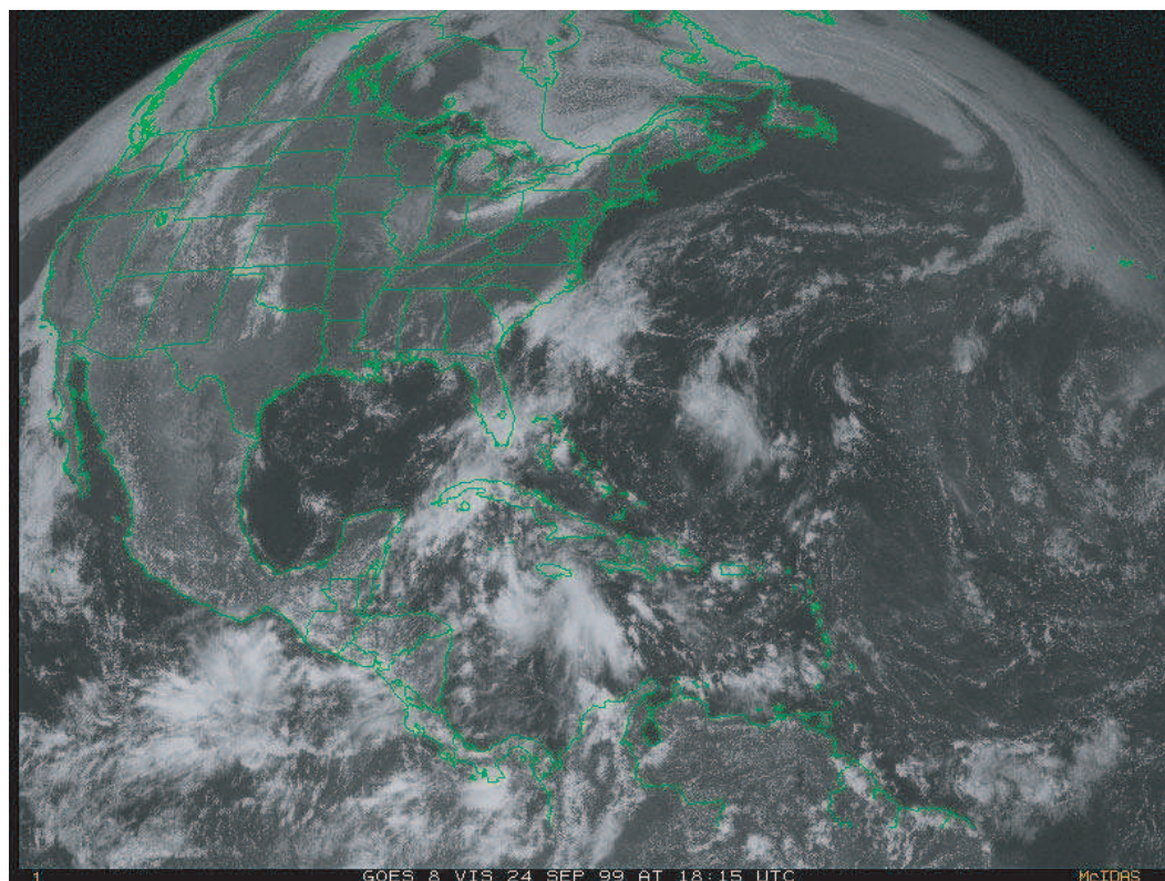
Figure n°52 : Analyse de la photo satellite du 24/9/1999, GOES 8, est, vis, 18h15 T.U (D'après carte de la NOAA, "Tropical surface analysis, Atlantic", 18h00 T.U) (D'après carte de la GEIC, "Systemas principales", 11h45 heure locale)
