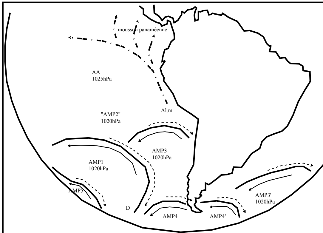
Figure n°15(C) : Analyse de la photo satellite du 24/9/2001 (D'après carte de la NOAA, "Weather pub fax", 18h00 T.U)
