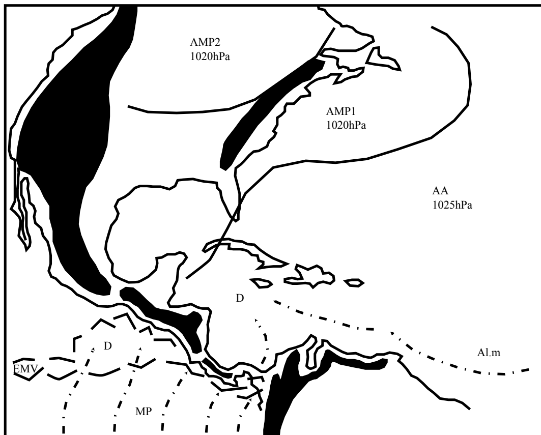
Figure n°52 : Analyse de la photo satellite du 24/9/1999, GOES 8, est, vis, 18h15 T.U (D'après carte de la NOAA, "Tropical surface analysis, Atlantic", 18h00 T.U) (D'après carte de la GEIC, "Systemas principales", 11h45 heure locale)
