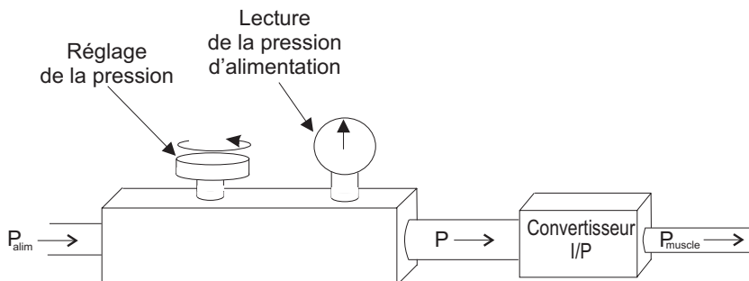
FIG. 5.28 – Système d'alimentation en air
