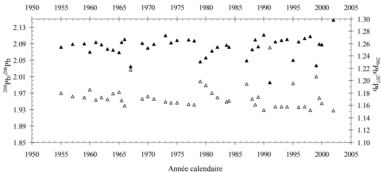
Figure 34 : Evolution, sur la période 1955-2002, des rapports 208 Pb/ 206 Pb (axe de gauche : ▲) et 206 Pb/ 207 Pb (axe de droite : Δ) mesurés dans le squelette d'aragonite de la colonie de Montastrea faveolata .
