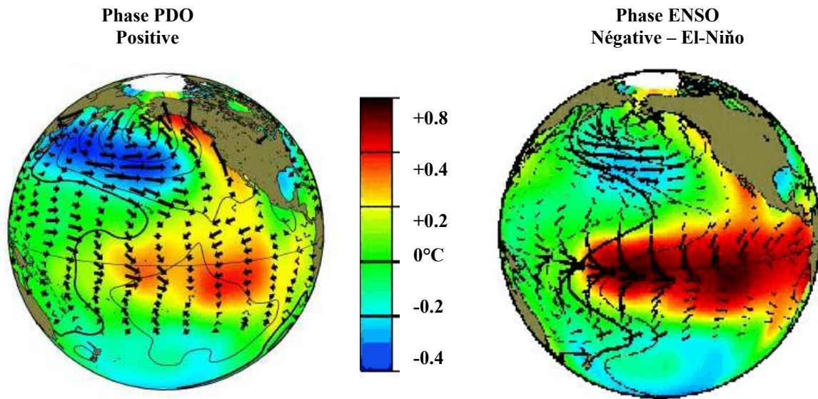
Figure 49 : Comparaison des situations climatiques de type PDO + et El-Niño. Les cartes représentent dans les deux situations les anomalies de SST (couleurs) et de flux aériens (flèches) au niveau de la mer.
