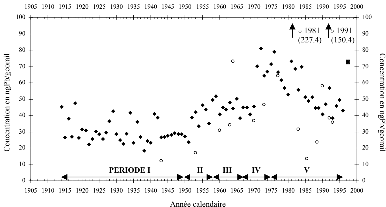
Figure 30 : Evolution des teneurs en plomb ( \text{ngPb/g}_{\text{corail}} ) dans le squelette des colonies coralliennes de l'île de Mona (■) et de La Parguera (○).
