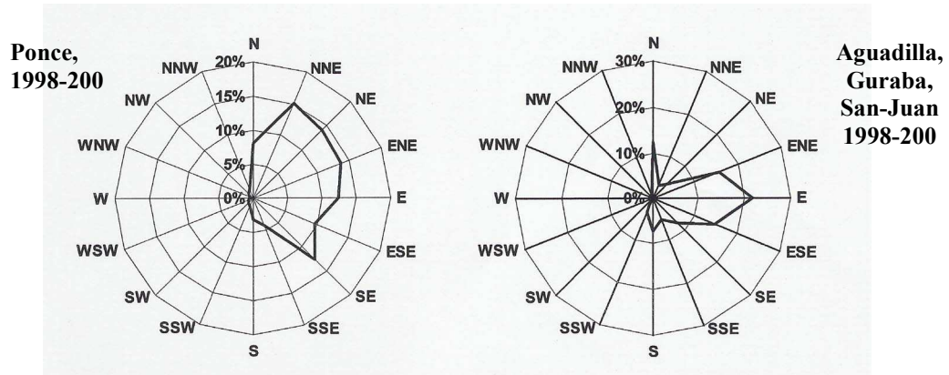
Figure 17 : Roses des vents pour la ville de Ponce entre 1998 et 2002 et sur 3 autres sites de Porto-Rico (Aguadilla, Gurabo et San-Juan ; Altaii et Farrugia, 2003).
