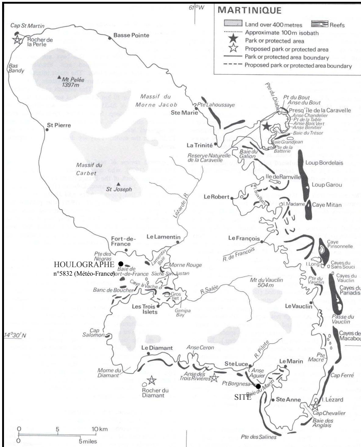
Figure 26 : Positions géographiques de la colonie de Montastrea faveolata récoltée en Juin 2002 lors de la mission « CEREGE Caraïbe » et du houlographe Météo-France (5832) sur l'île de la Martinique.
