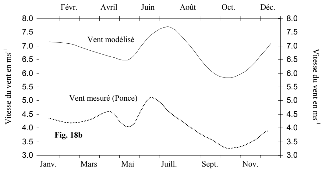
Figure 18 : -18a- Historique mensuel de l'intensité des vents modélisée sur une grille de 2° de latitude et de longitude centrée sur l'île de Mona (64°W, 17°N) entre 1950 et 1998 (source Ocean Atmosphere Mean Wind Speed dataset, Nyberg, comm. perso.) -18b- Evolution annuelle de l'intensité des vents calculée à partir des données modélisées et comparaison avec les données mesurées à la station météorologique de la ville de Ponce (Est La Parguera – source Altaii et Farrugia, 2003).
