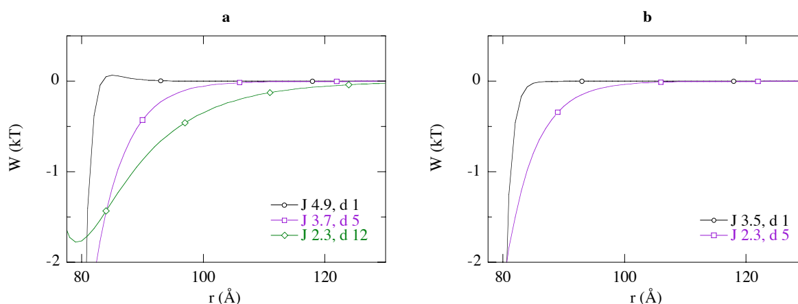
Figure 6.14 : Résultante des potentiels électrostatique et attractif de type Yukawa utilisés pour modéliser les facteurs de structure expérimentaux de la Hm MalDH en (a) (\text{NH}_4)_2\text{SO}_4 0.25 M, MPD 40% et (b) (\text{NH}_4)_2\text{SO}_4 3 M, MPD 0% (réf. D22 00.10). Le potentiel de volume exclu n'est pas pris en compte, il ajouterait simplement un terme infiniment positif en dessous de 80 \text{\AA} et nul au-dessus pour un diamètre D de la particule de 80 \text{\AA} . La charge Z de la protéine est de 30. La profondeur J du potentiel attractif est exprimée en kT et sa portée d en \text{\AA} .
