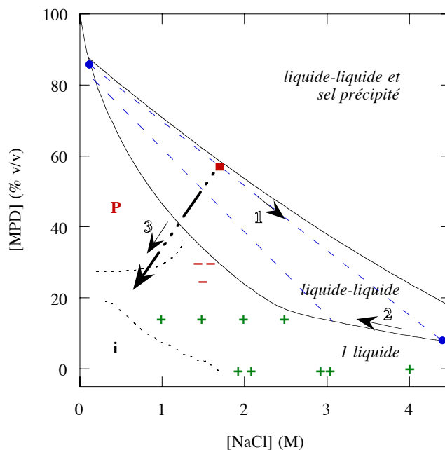
Figure 5.1 : Cheminement de la Hm MalDH dans le diagramme de phases NaCl – MPD – H 2 O lors de sa cristallisation. Les traits pleins représentent les courbes de coexistence de phases à 22°C [d’après Richard et al. , 1995]. Les courbes en pointillés délimitent les zones où la Hm MalDH est inactive (i) et où elle précipite (P) à 25.5 mg/ml à température ambiante. Les valeurs expérimentales du second coefficient du viriel A 2 sont indiquées par “++” pour des valeurs supérieures à 4 10 -5 mol.l.g -2 , par “+” pour des A 2 compris entre 2 et 4 10 -5 mol.l.g -2 et par “-” et “--” pour des A 2 d’environ -2 et -10 10 -5 mol.l.g -2 . La goutte initiale (■) est constituée de deux phases (●). Durant la dilution globale de la goutte (flèche grasse hachurée), la composition de la phase contenant la protéine suit le cheminement 1, 2 et 3.
