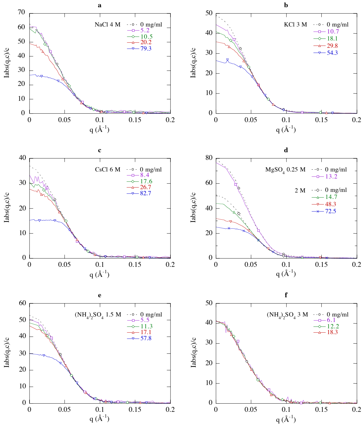
Figure 4.1 : Courbes de diffusion de neutrons par des solutions de Hm MalDH en différents sels, en fonction de la concentration en protéine c en mg/ml, à 20-25°C et pH 8-8.2. (a) NaCl 4 M (réf. D22 00.4)* ; (b) KCl 3 M (réf. D11 98.2) ; (c) CsCl 6 M (réf. D22 99.9) ; (d) MgSO 4 0.25 et 2 M (réf. D11 98.7) ; (e-f) (NH 4 ) 2 SO 4 1.5 et 3 M (réf. D22 00.10). Les courbes à concentration nulle correspondent aux facteurs de forme. Ils ont été déterminés par l'extrapolation linéaire des I_{\text{abs}}(q,c)/c , pour chaque valeur de q , sur les trois plus faibles concentrations en protéine, puis faiblement lissés. Les points à q = 0 sont extrapolés selon l'approximation de Guinier.
