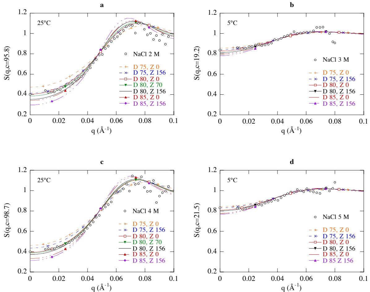
Figure 4.4 : Modélisation des facteurs de structure S(q,c) de la Hm MalDH en NaCl pH 8.2 (2 et 4 M, à 25°C : réf. D22 97.8 ; 3 et 5 M, à 5°C : réf. D11 97.4). Les "o" correspondent aux S expérimentaux et les lignes aux S calculés à partir d'un potentiel de volume exclu caractérisé par le diamètre D en Å et d'un potentiel coulombien avec une charge protéique Z . Les concentrations en protéine c sont en mg/ml. En NaCl, la température n'a pas d'effet notable sur les interactions.
