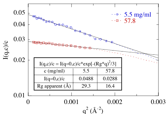
Figure 2.2 : Détermination par l'approximation de Guinier des valeurs apparentes des intensités diffusées à angle nul I(q=0,c)/c et des rayons de giration R_g pour des solutions de Hm MalDH à 5.5 et 57.8 mg/ml en (NH_4)_2SO_4 1.5 M (réf. D22 00.10 * ). Les régressions linéaires de \ln[I(q,c)/c] portent sur la partie des intensités représentées par des ronds ou des carrés, qui correspondent à un domaine angulaire plus restreint que celui respectant la condition R_g q < 1.3 .
