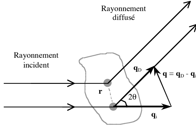
Figure 2.1 : Géométrie de la diffusion élastique : chaque diffuseur élémentaire d'une particule diffuse le rayonnement incident de vecteur d'onde \mathbf{q}_i dans toutes les directions. Les diffusions selon la direction \mathbf{q}_D de deux diffuseurs distants de \mathbf{r} sont déphasées de \mathbf{q}\mathbf{r} . Pour une diffusion élastique, q_i = q_D = 2\pi/\lambda et q = 4\pi\sin\theta/\lambda , où \lambda est la longueur d'onde et 2\theta l'angle de diffusion.
