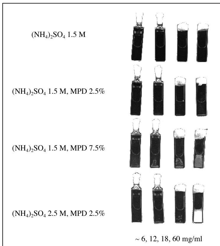
Figure 6.4 : Séries de cuves d'échantillon de Hm MalDH en sulfate d'ammonium et MPD pour la diffusion de neutrons (réf : D22 00.10). Les cuves (1.2 cm de largeur) ont été scannées sur un fond noir afin d'obtenir un meilleur contraste. Lorsque la concentration du sel ou du MPD augmente, un gel blanchâtre apparaît proportionnellement à la concentration en protéine.
