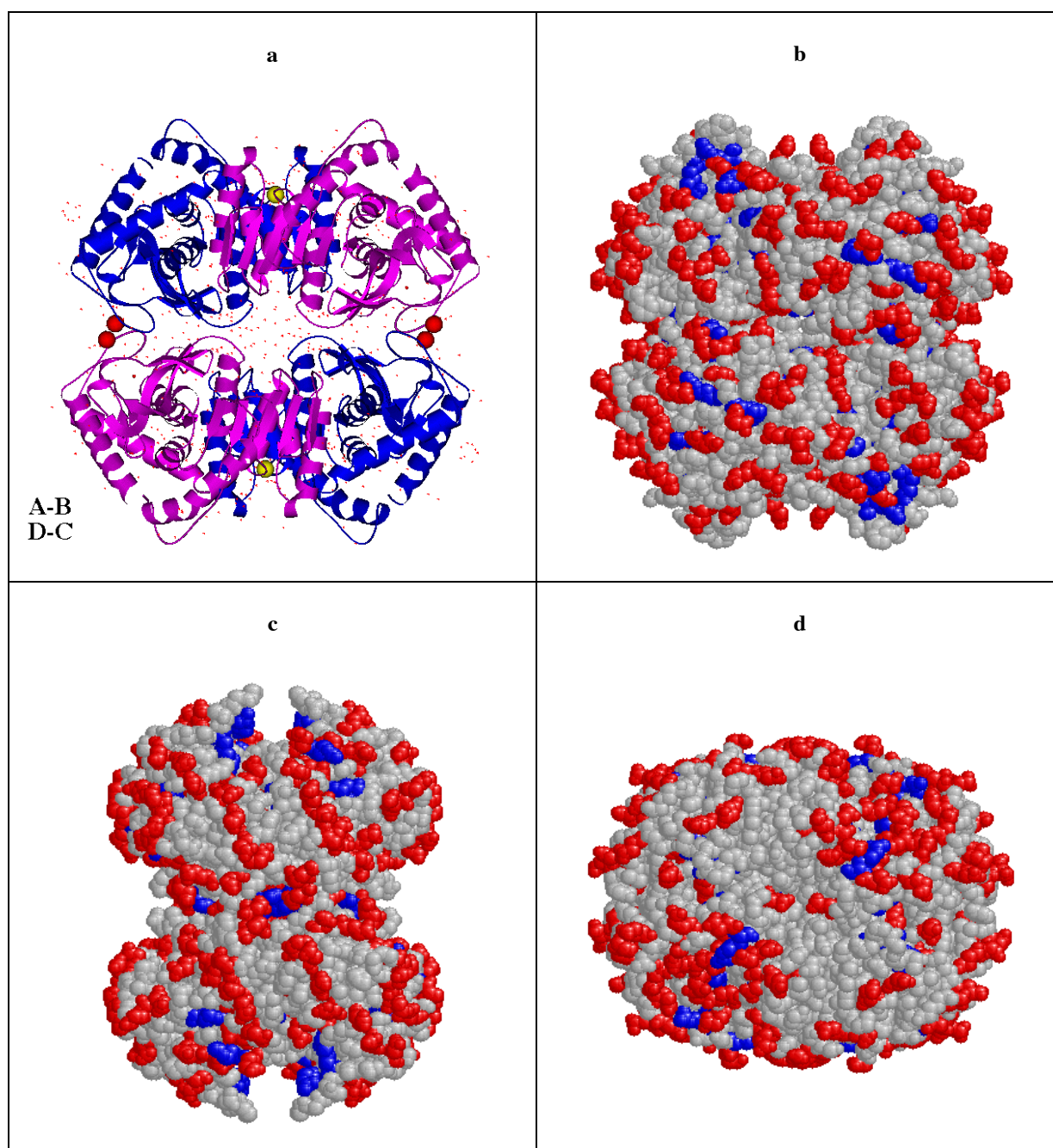
Figure 1.2 : Structure quaternaire de la Hm MalDH. (a) Représentation en ruban des quatre chaînes polypeptidiques A, B, C et D : les deux ions \text{Na}^+ (boules jaunes) participent aux ponts salins entre les monomères des deux dimères A-B et D-C et les quatre ions \text{Cl}^- (boules rouges) aux ponts salins entre les deux dimères. Les molécules d'eau sont représentées par les points rouges [Richard et al. , 2000]. Les dimensions externes du tétramère sont : A-B 77 Å, A-D 80 Å et A-C 90 Å. (b, c, d) Les atomes des résidus acides et basiques sont représentés respectivement en rouge et en bleu (vues de face, de profil et de dessus).
