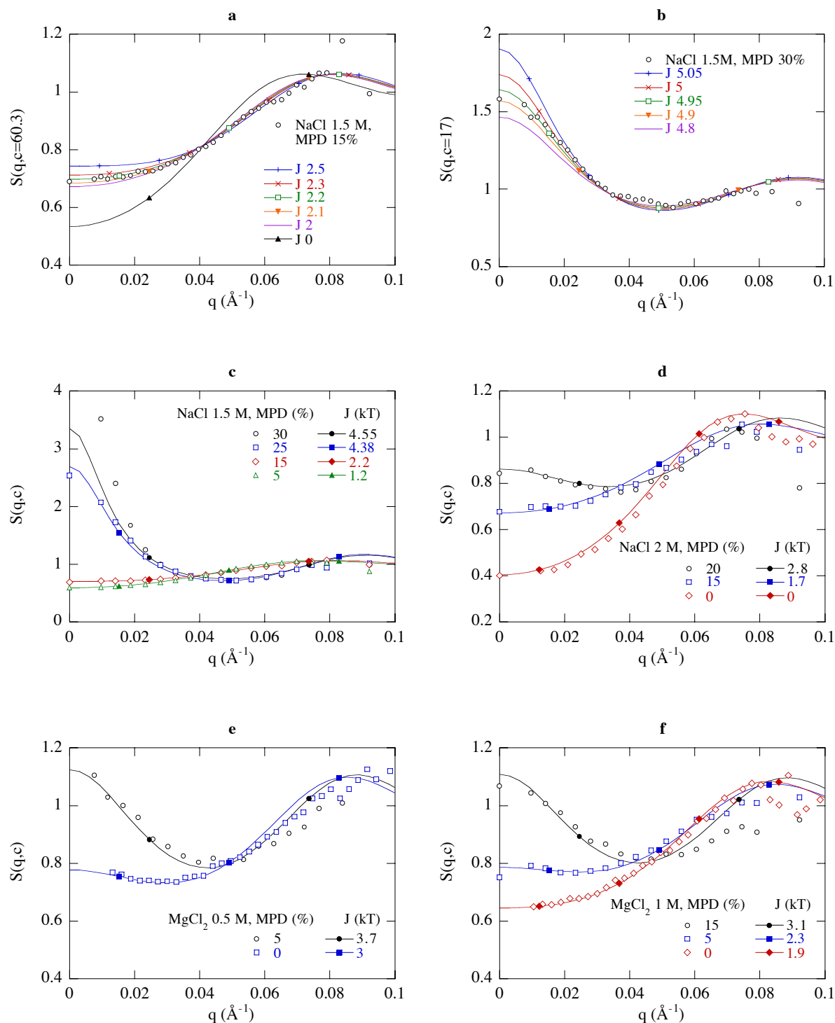
Figure 6.8 : Modélisation des facteurs de structure S(q,c) de la Hm MalDH en NaCl et \text{MgCl}_2 en présence de MPD, à pH 8-8.2 et à 20-25°C (réf. D11 99.6, sauf NaCl 2 M : D22 97.8, \text{MgCl}_2 0.5-1 M : Lure 98.12). Les symboles creux correspondent aux S expérimentaux et les lignes aux S calculés à partir d'un potentiel de volume exclu caractérisé par le diamètre D de 80 Å, d'un potentiel coulombien avec une charge protéique Z de 70 et d'un potentiel attractif de profondeur J en kT et de 5 Å de portée. Les concentrations en protéine c en mg/ml sont (de haut en bas) : (c) 50, 67.9, 60.3 et 61.3 ; (d) 65.6, 59.1 et 95.8 ; (e) 66 et 79.6 (f) 61.2, 64.5 et 79.2.
