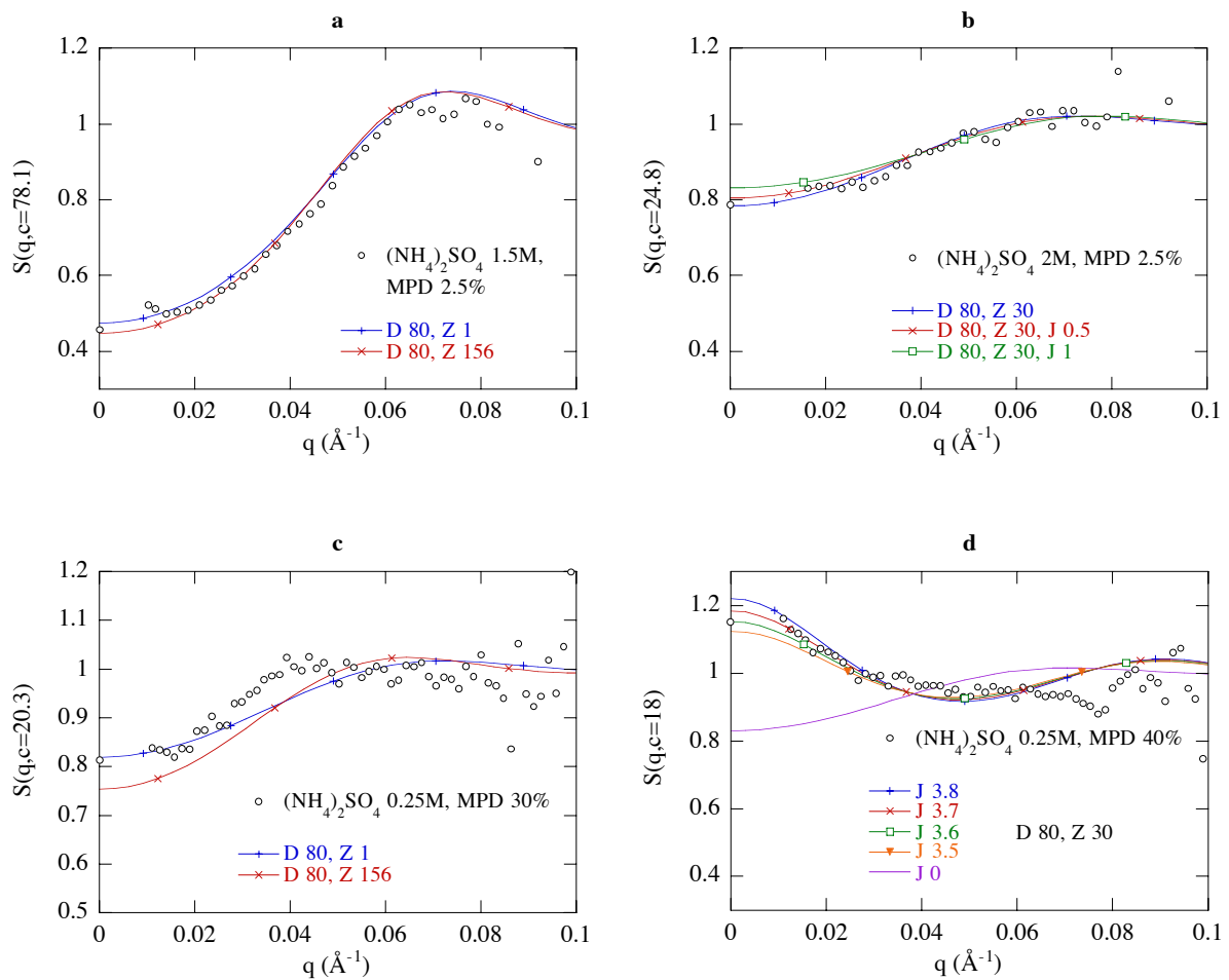
Figure 6.9 : Modélisation des facteurs de structure S(q,c) de la Hm MaldH en (\text{NH}_4)_2\text{SO}_4 en présence de MPD, à pH 8 et à 25°C (réf. D11 00.8 et D22 00.10). Les symboles creux correspondent aux S expérimentaux et les lignes aux S calculés à partir d'un potentiel de volume exclu caractérisé par le diamètre D de 80 Å, d'un potentiel coulombien avec une charge protéique Z et d'un potentiel attractif de profondeur J en kT et de 5 Å de portée. Les concentrations en protéine c sont en \text{mg/ml} .
