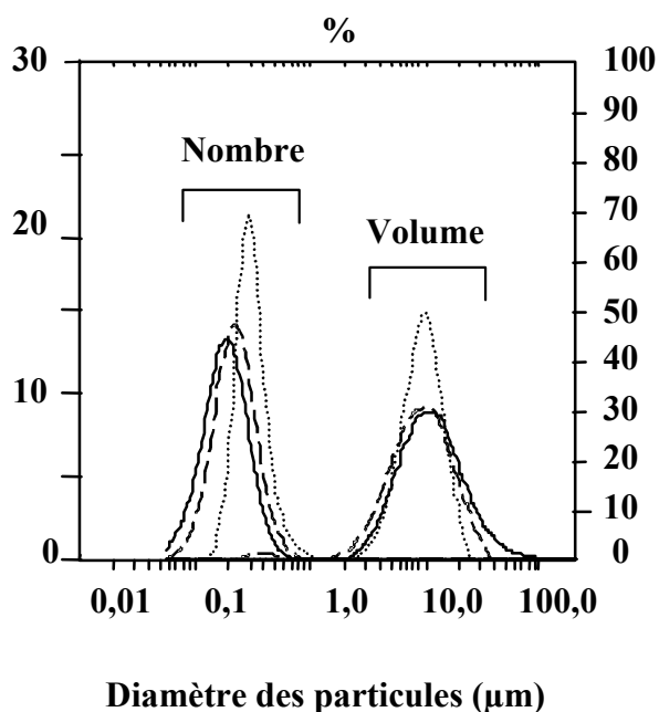
Figure 2.15 : Distribution de taille en volume et en nombre d'agrégats de \beta -lg dans une dispersion à pH 4,2 et 20°C. Concentrations protéiques : (—) 0,5%, (—) 1%, (.....) 5%.
