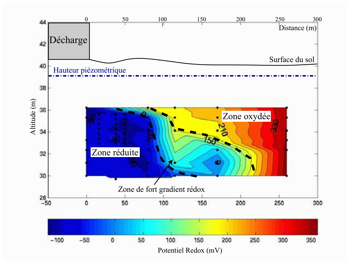
FIG. 4.3 – Carte du potentiel rédox réalisé à partir de mesures effectuées sur la décharge de Grindsted au Danemark par Bjerg et al. (1995).
