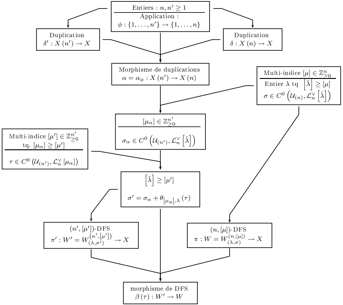
FIG. 9.2.1. Construction d'un morphisme dans la catégorie \mathcal{D} .
