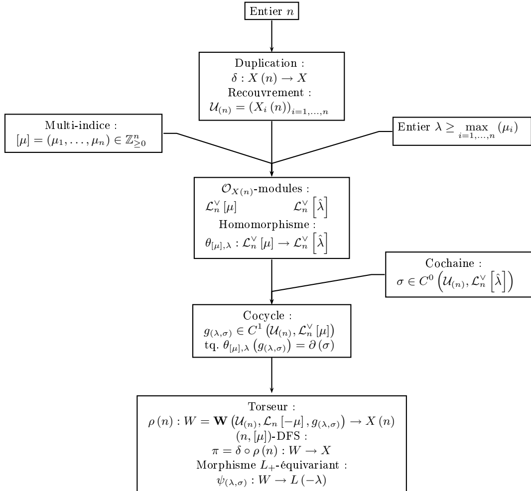
FIG. 9.1.1. Construction d'un (n, [\mu]) -DFS à partir d'une paire (\lambda, \sigma) .
