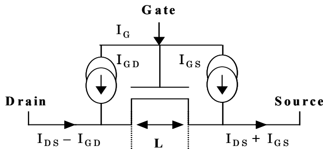
Figure III.20. Vue schématique d'un transistor NMOS avec fuite de grille (GLNMOS).
