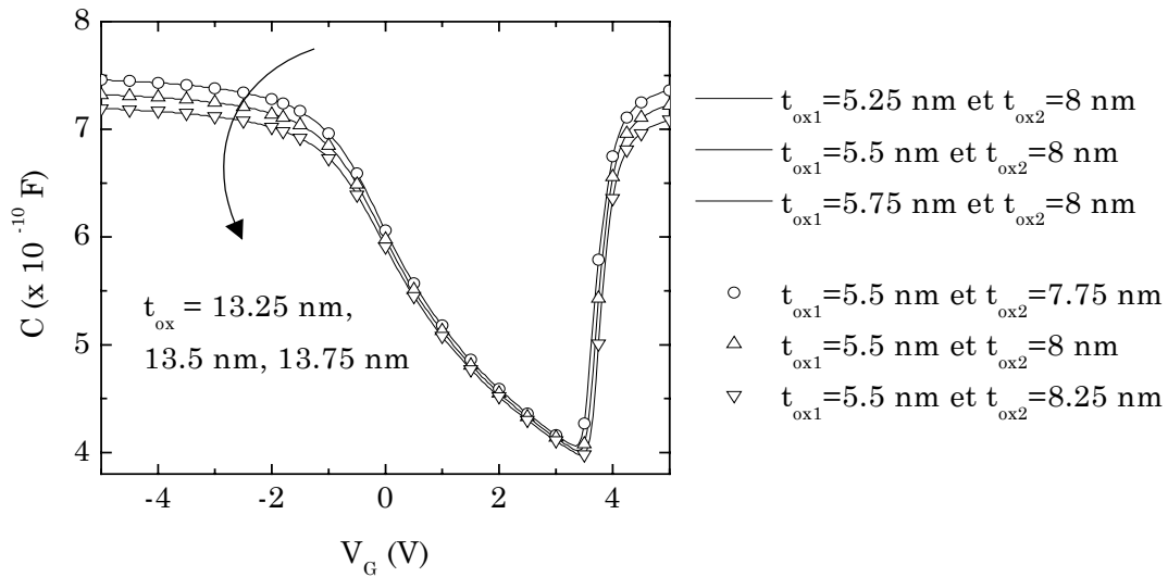
Figure IV.14. Simulation des courbes C-V de capacités à nodules en fonction de la variation des épaisseurs d'oxydes t_{ox1} et t_{ox2} . Les paramètres de simulations sont : N_A = 1.3 \cdot 10^{24} \text{ m}^{-3} , A_{eff} = 3 \cdot 10^{-7} \text{ m}^2 , V_{FB} = -1 \text{ V} , N_{dot} = 16 \cdot 10^{15} \text{ m}^{-2} , D_{dot} = 4.5 \text{ nm} .
