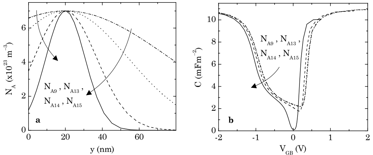
Figure II.13. Profils du dopage (a) et courbes C-V correspondantes (b) si l'on considère une gaussienne centrée à 20 nm de l'interface et de largeur variable. L'épaisseur d'isolant est de 3 nm.
