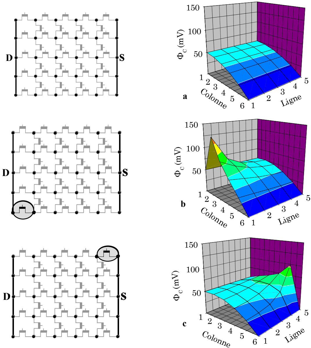
Figure III.28. Simulations de la distribution des quasi-niveaux de Fermi, \Phi_C(x,y) pour un transistor sans défaut avec t_{ox} = 1.5 nm (a) et des transistors ayant un défaut soit côté drain (b) , soit côté source (c) pour V_{DS} = 50 mV et V_{GS} = 1.2 V [Bernardini'04c].
