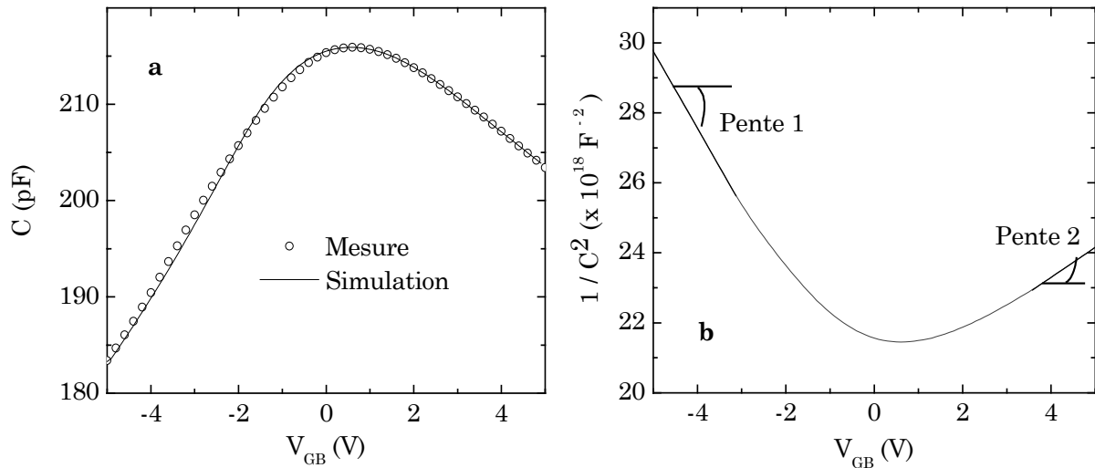
Figure II.8. Comparaison pour une capacité SOS avec poly-désertion de grille d'une courbe C - V mesurée et d'une courbe C - V simulée (a). Extraction du dopage de substrat N_{sub} et du dopage de grille N_G à partir du tracé de 1/C^2 en fonction de V_{GB} (b). Les dimensions de la capacité mesurée sont W \times L = 56000 \mu\text{m}^2 . Les paramètres extraits sont : N_{sub} = 1.721 \times 10^{25} \text{ m}^{-3} , N_G = 4.19 \times 10^{25} \text{ m}^{-3} et t_{ox} = 8.3 \text{ nm} .
