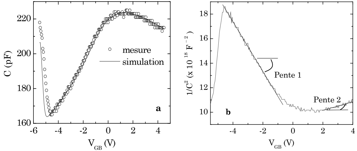
Figure II.7. Comparaison, pour une capacité MOS avec poly-désertion de grille, d'une courbe C - V mesurée et d'une courbe C - V simulée (a). Extraction du dopage de substrat N_{sub} et du dopage de grille N_G à partir du tracé de 1/C^2 en fonction de V_{GB} (b). Les paramètres de la capacité mesurée sont : t_{ox} = 11 \text{ nm} , V_{FB} = -1 \text{ V} , W \times L = 30000 \mu\text{m}^2 . Les dopages extraits sont : N_{sub} = 2 \times 10^{23} \text{ m}^{-3} et N_G = 1 \times 10^{26} \text{ m}^{-3} .
