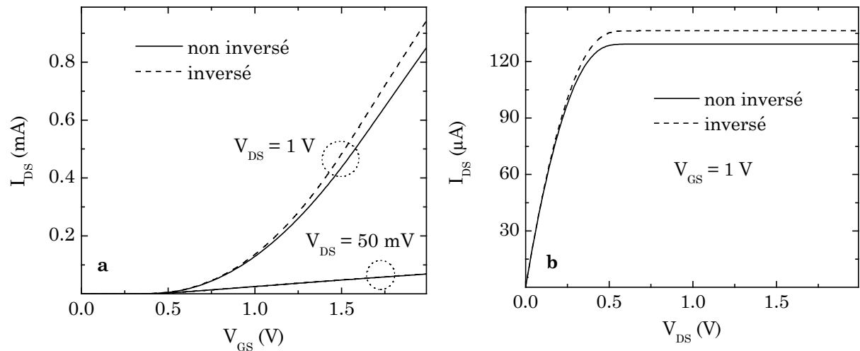
Figure III.12. Courbes I_{DS}(V_{GS}) (a) et I_{DS}(V_{DS}) (b) pour un transistor MOS à résistances d'accès dissymétriques, R_S = 100\ \Omega et R_D = 0\ \Omega , en inversant ou non source et drain. Les paramètres du TMOS sont : W \times L = 1 \times 0.5\ \mu\text{m}^2 , t_{ox} = 3\text{ nm} , N_A = 7 \times 10^{23}\text{ m}^{-3} et \mu_0 = 500\text{ cm}^2\text{V}^{-1}\text{s}^{-1} .
