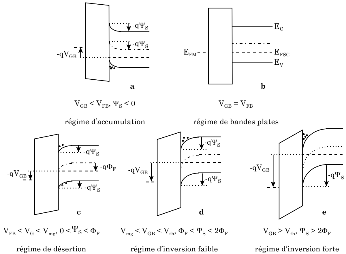
Figure I.2. Diagrammes de bandes représentant les différents régimes du semi-conducteur en fonction du potentiel appliqué : le régime d'accumulation (a), le régime de bandes plates (b), le régime de désertion (c), le régime d'inversion faible (d) et le régime d'inversion forte (e).
