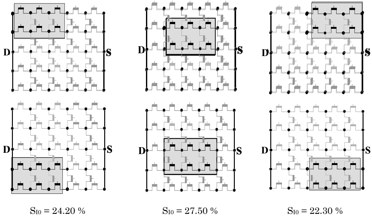
Figure III.34. Schématisation des transistors M2 affectés par une réduction de t_{ox} et pourcentages d'erreur sur le courant dupliqué I_0 (pour V_{GP} = 0V ).
