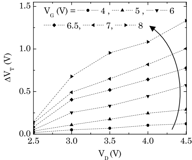
Figure IV.19. Variation de la tension de seuil d'un transistor ( W = 0.16 \mu\text{m} , L = 0.28 \mu\text{m} ) situé sur la demi-plaque 2, en fonction du potentiel de drain pour différentes tensions de grille appliquées durant un temps d'écriture égal à 10 \mu s (la lecture se fait à V_D = 50 mV).
