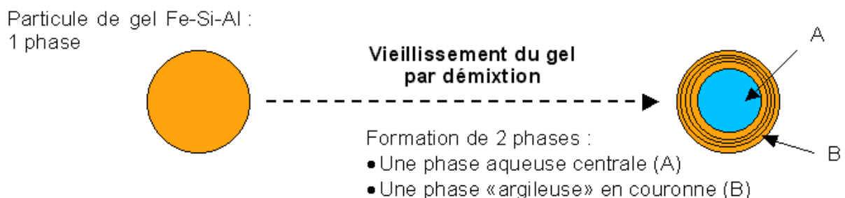
Figure 97 : Représentation simplifiée du modèle d'Eggleton pour la cristallisation de feuilletts argileux à partir d'oxyhydroxydes de Fe-Si-Al naturels (Kohler, E. et al. 2001)
