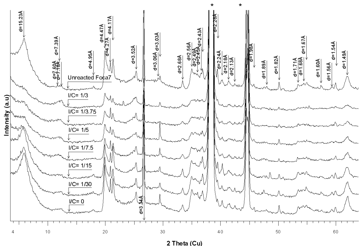
Figure 30 : Comparaison des diffractogrammes des mélanges réactionnels à celui de FoCa7 de référence. Les pics annotés d'un astérisque * sont ceux de l'aluminium dont sont faits les portoirs à échantillons. I/C correspondent aux rapports massiques Fe(0)/argile.
