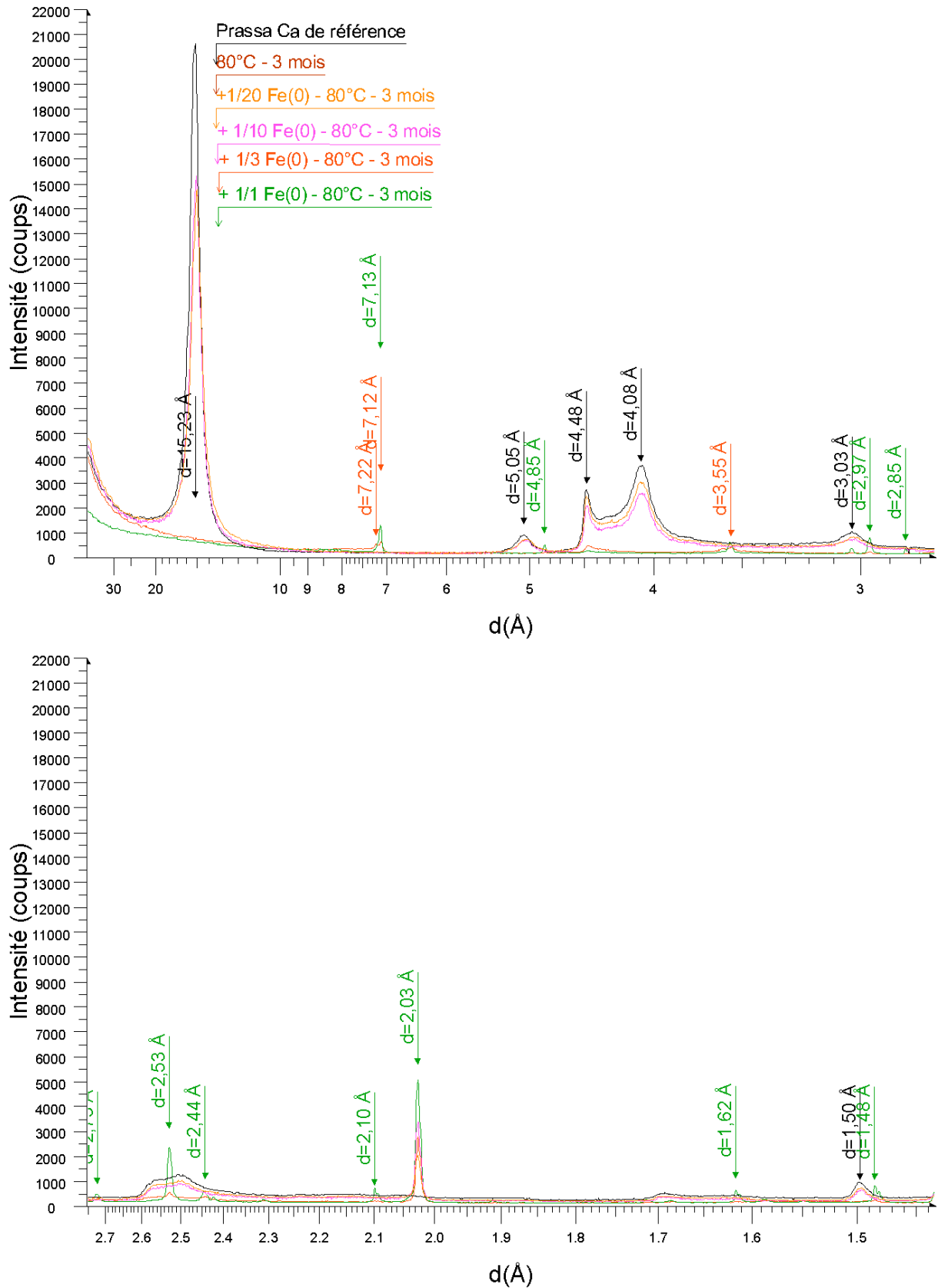
Figure 79 : Comparaison des diffractogrammes de rayons X des mélanges "PrassaCa-Fe(0), F/A variant de 0 à 1, après réaction de 3 mois à 80°C
