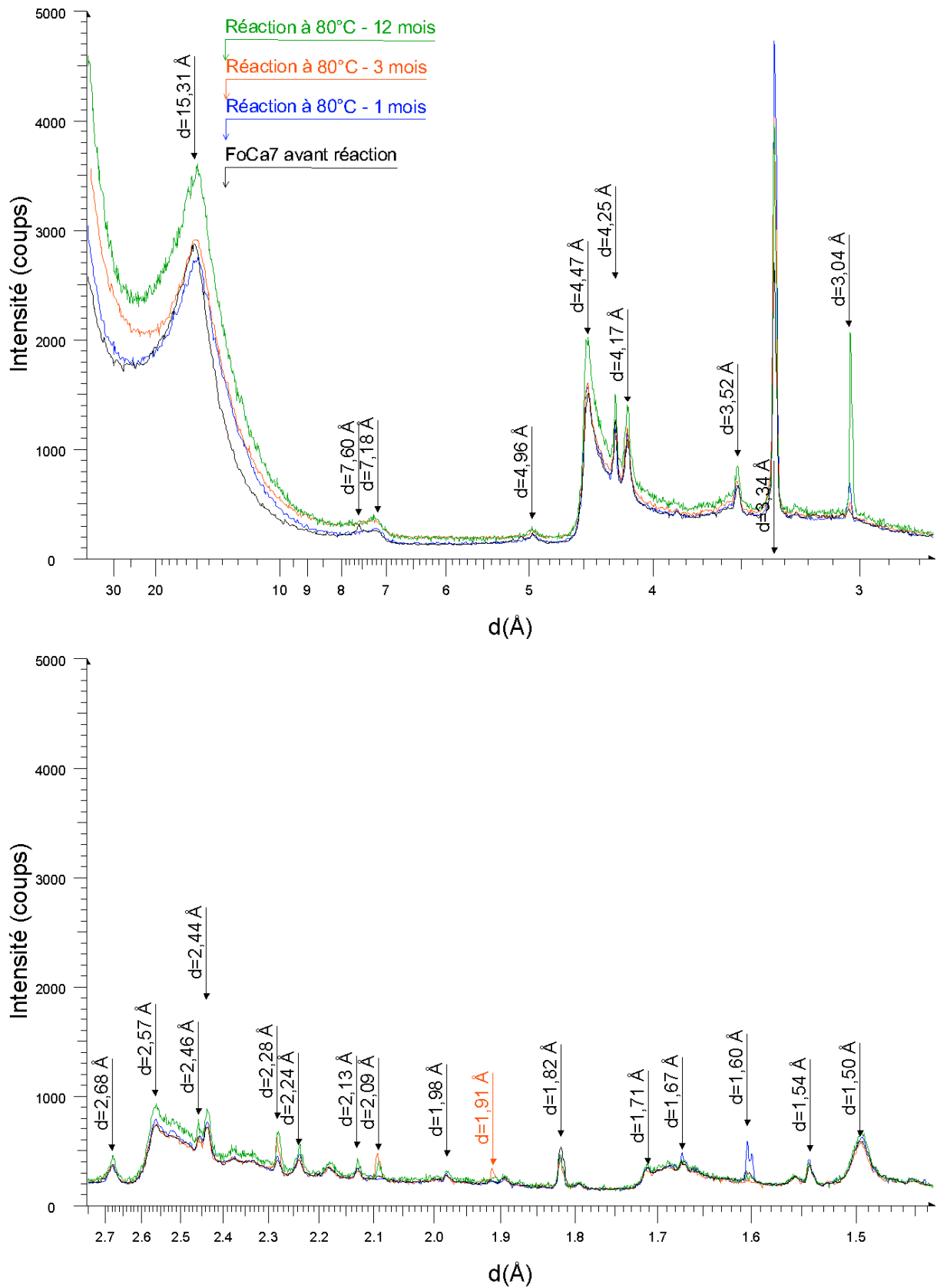
Figure 50 : Spectres DRX des essais sans fer (F/A=0) en fonction de la durée d'expérimentation comparés à FoCa7 avant réaction. Essais à 80°C.
