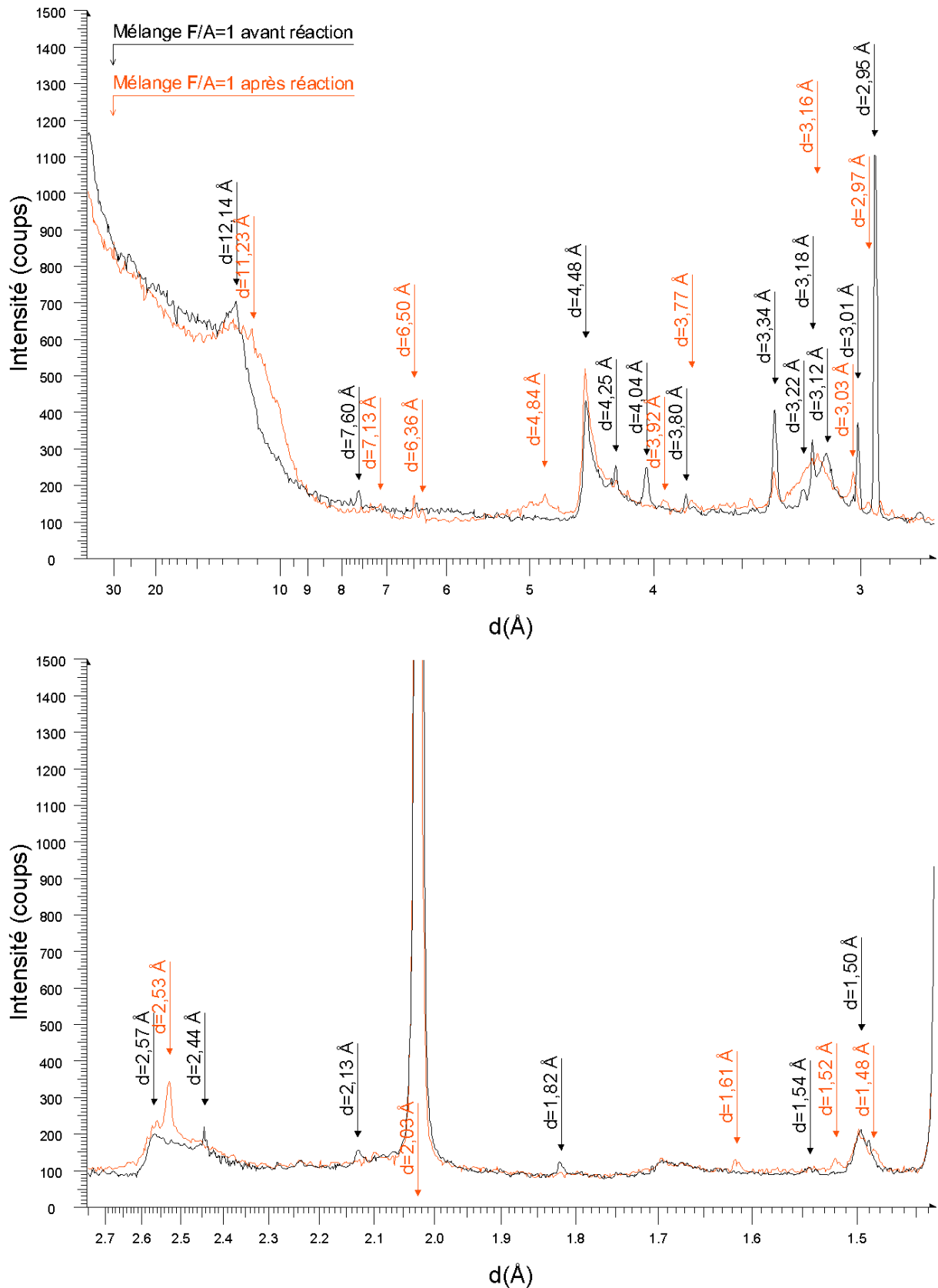
Figure 41: Comparaison du diffractogramme de rayons X du mélange « MX-80 + Fe(0) F/A=1 » avant et après réaction à 80°C pendant 3 mois.
