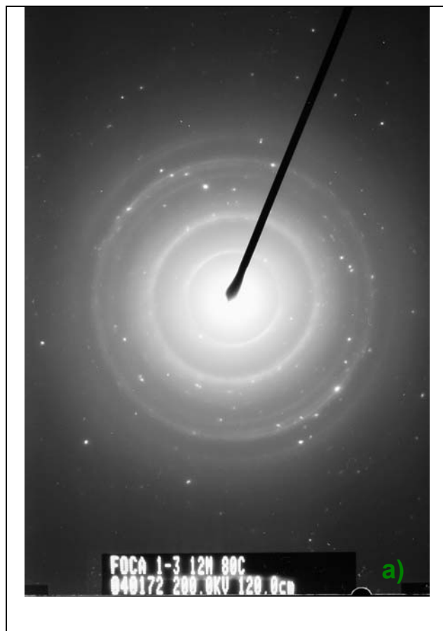
Planche 2 : Cliché de diffraction de relisque de smectite
