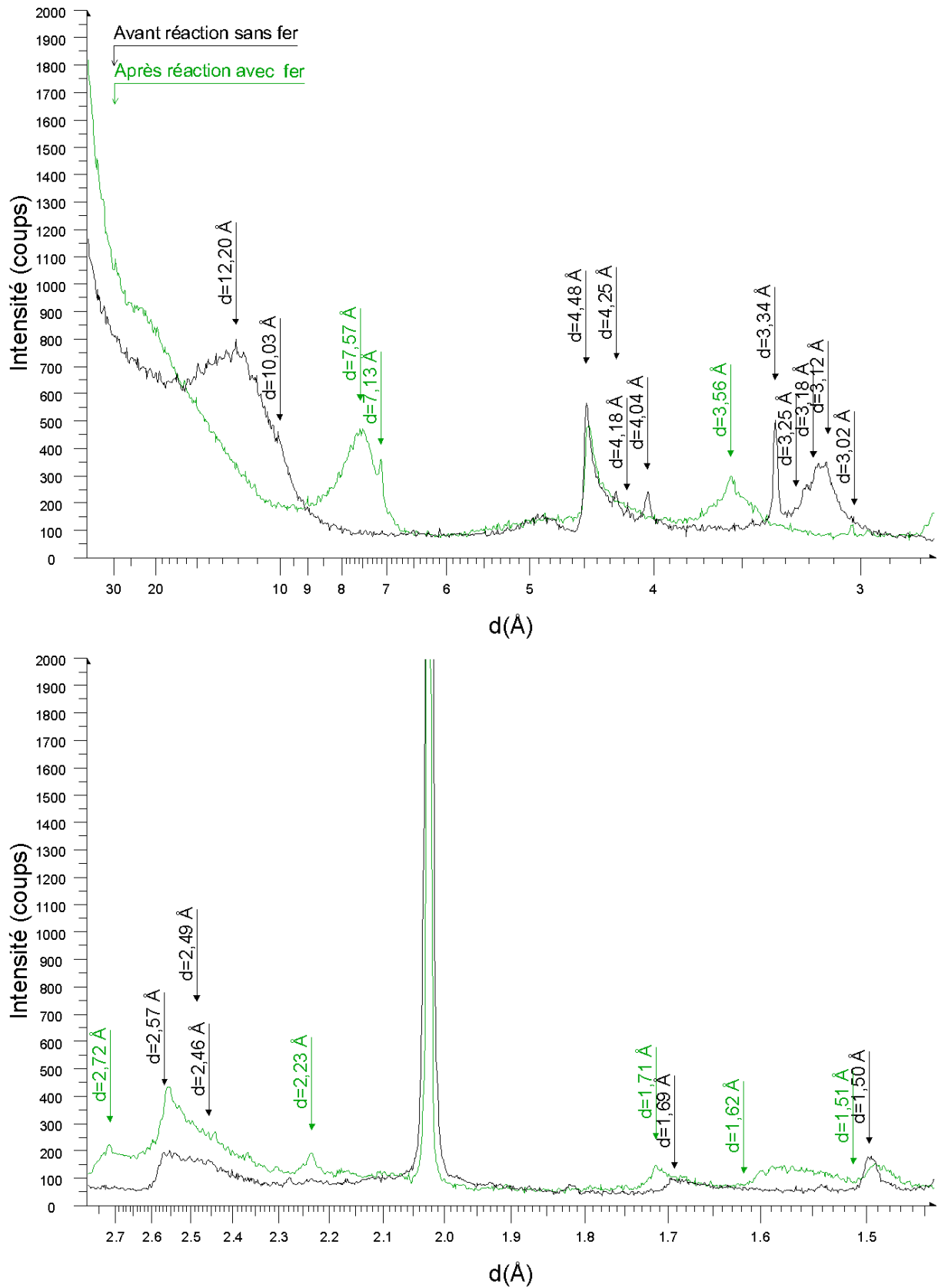
Figure 68 : Comparaison du diffractogramme de rayons X du mélange « MX80 purifiée-Fe(0), F/A=1 » avant et après réaction à 80°C pendant 3 mois
