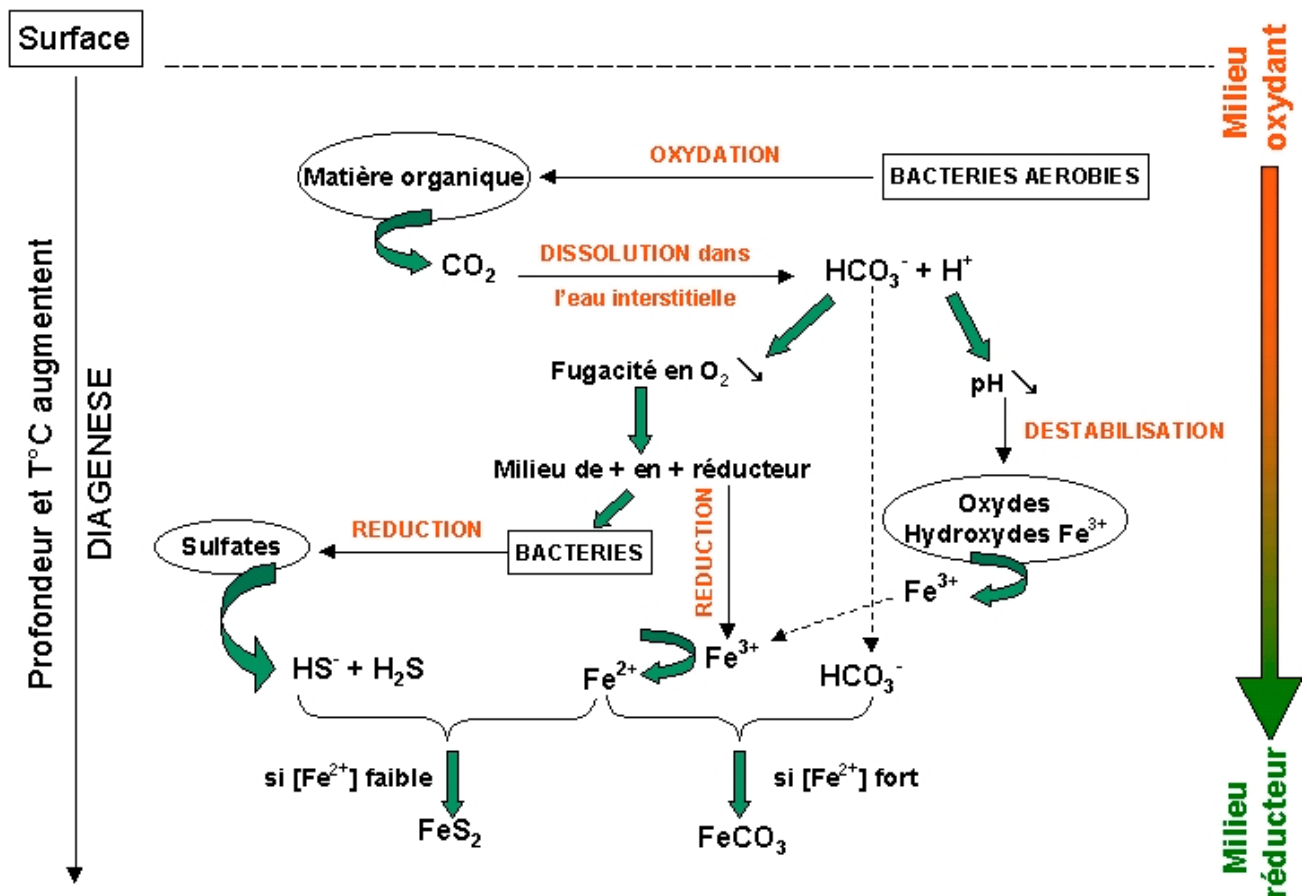
Figure 13 : Schématisation des réactions diagénétiques d'après les textes de (Dapples, E. C. 1979) et (Fairbridge, R. W. 1967)
