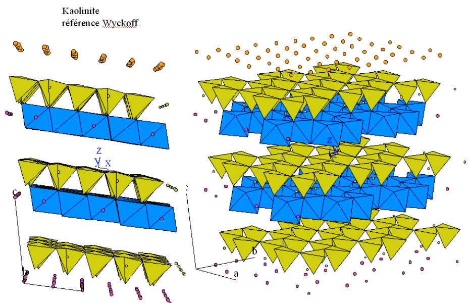
Figure 2 : Structure 3D d'une kaolinite, feuillelet à 7 Å, motif dit TO
