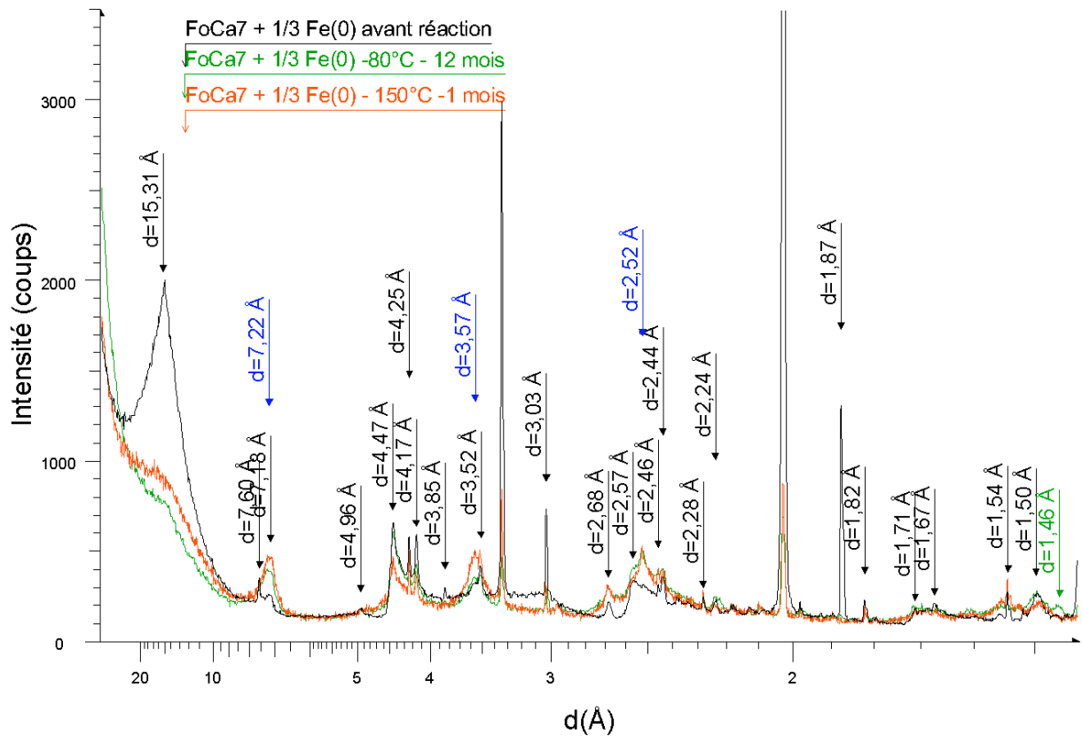
Figure 66 : Comparaison des diffractogrammes des produits de réaction du mélange "FoCa7 + 1/3 Fe(0)" après essai à 80°C pendant 12 mois ou à 150°C pendant 1 mois.
