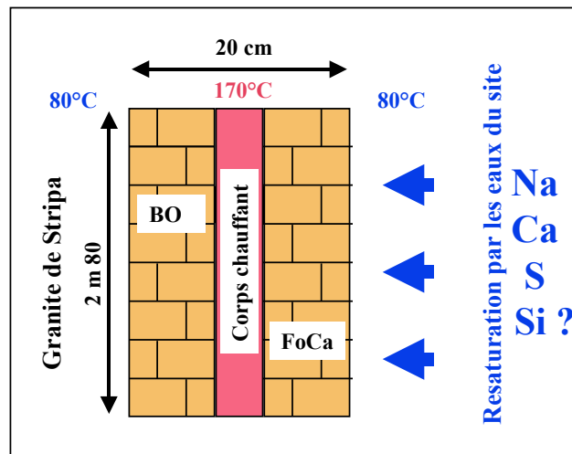
Figure 24 : Schéma de principe de l'essai in-situ Stripa (Latrille, C. et al. 2001)
