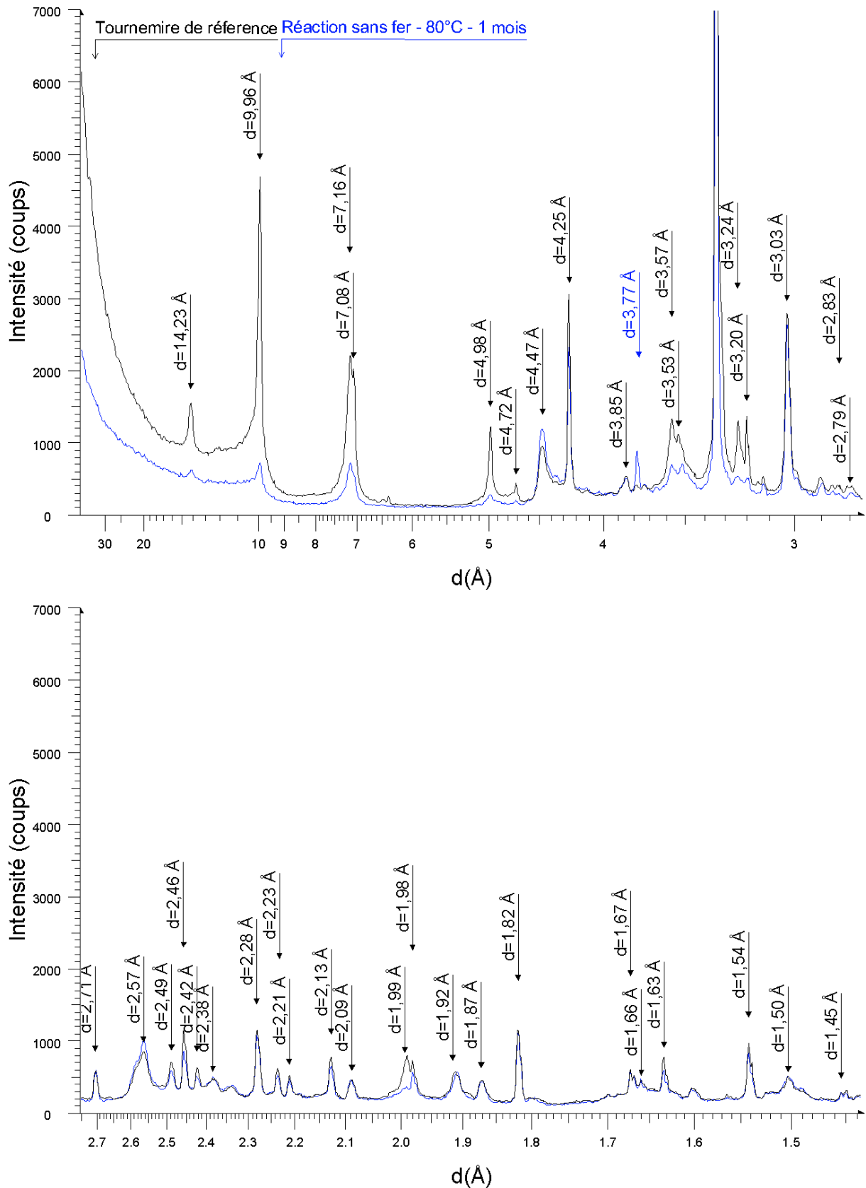
Figure 46 : Comparaison du diffractogramme de rayons X de l'argilite de Tournemire avant et après réaction sans fer ajouté à 80°C pendant 1 mois.
