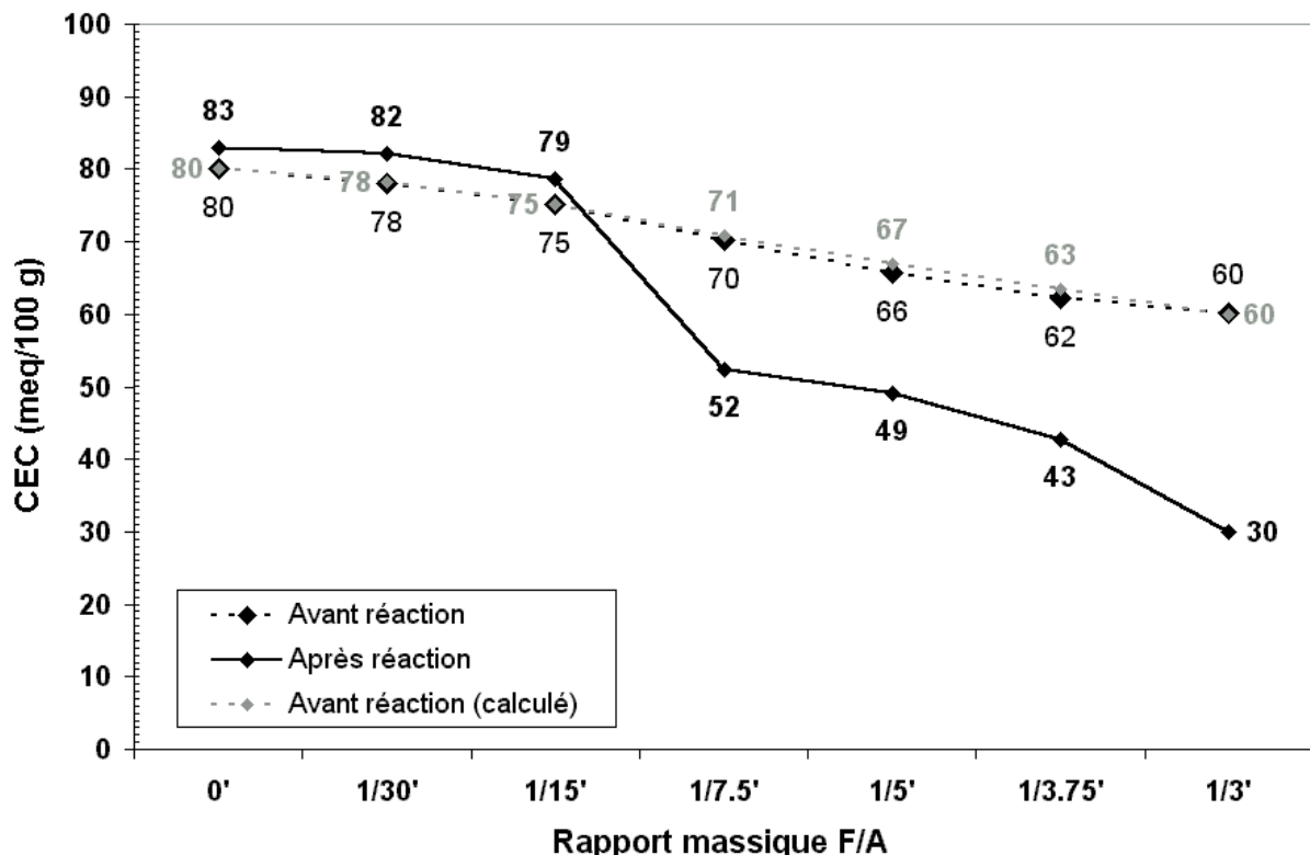
Figure 29 : CEC des mélanges réactionnels avant et après essai représentées en fonction du rapport massique Fe(0)/argile.
