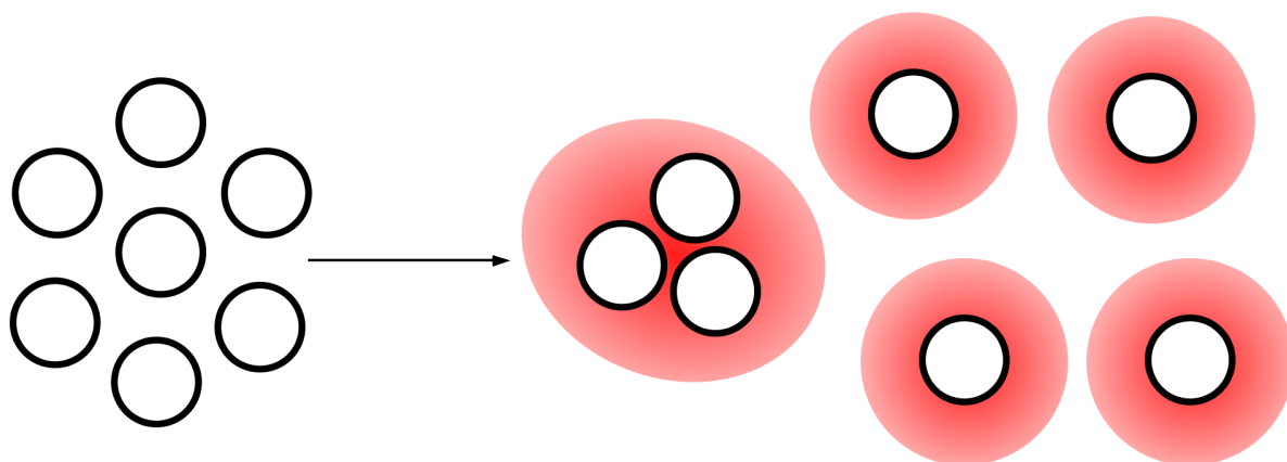
FIG. 4.14: Schéma de principe de l'individualisation des nanotubes. Gauche : Fagot de nanotube. Droite : Petit fagot et nanotubes individuels, entourés de leurs couronnes de surfactant.
