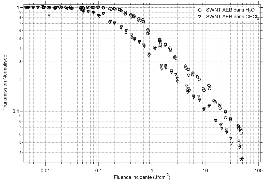
FIG. 6.3: Courbes de limitation optique d'une suspension de nanotubes de carbone mono-feuillets Arc Electrique Brut (SWNT AEB) dans l'eau et le chloroforme. La transmission linéaire des échantillons est ajustée à 70 % pour 532 nm. Banc petite ouverture F/50 , \lambda = 532 nm et \tau = 15 ns.
