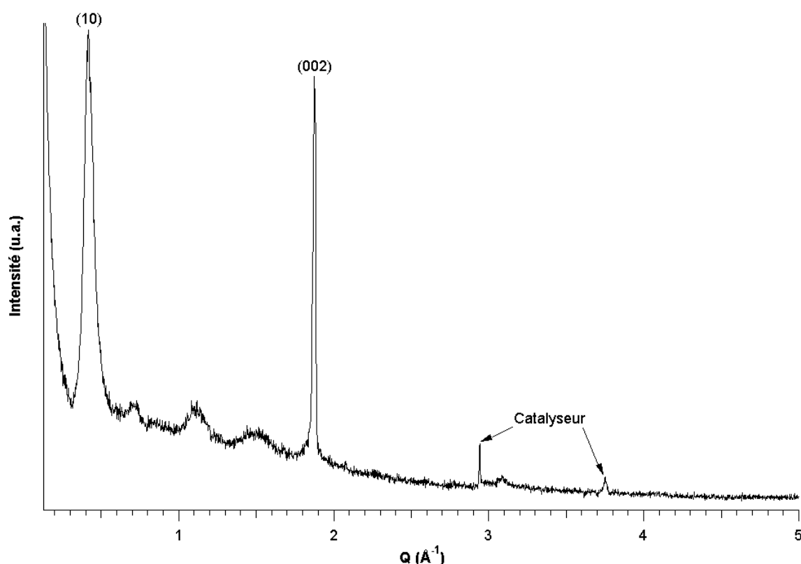
FIG. 4.6: Diffractogramme de rayon X de l'échantillon Arc Electrique Purifié.
