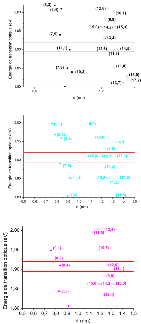
FIG. 5.8: Diagramme de Kataura calculé pour une intégrale de recouvrement \gamma_0 de 2,90 (haut), 2,83 (milieu) et 2,76 eV (bas). Ronds pleins, nanotubes semiconducteurs. Cercles, nanotubes métalliques. La ligne horizontale à 1,92 eV correspond à l'énergie du laser. La ligne du dessous correspond à l'énergie des photons diffusés en Stokes à 200\text{ cm}^{-1} .
