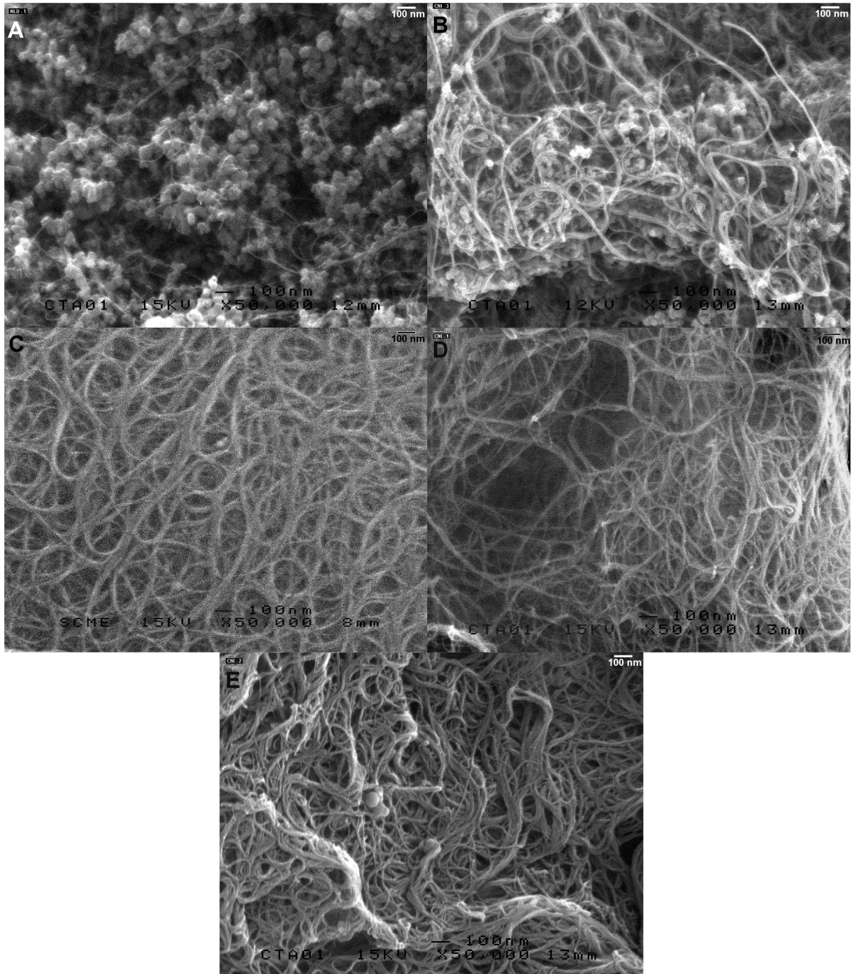
FIG. 4.1: Images de MEB des échantillons de SWNT. Grandissement 50000. A : Arc Electrique Brut. B : Ablation Laser. C : Arc Electrique Purifié. D : HiPCO Brut. E : HiPCO Purifié.
