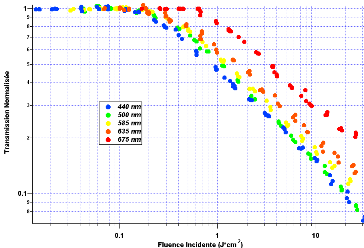
FIG. 2.7: Démonstration de l'efficacité large bande des suspensions de nanotubes. Durée d'impulsion : \tau=3,5 ns
