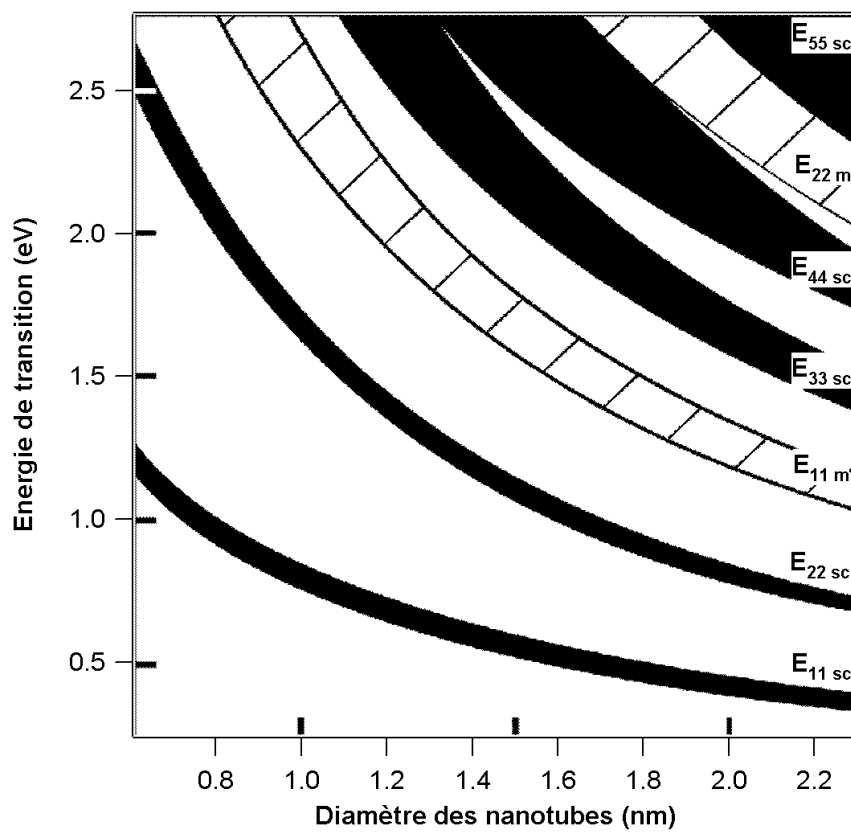
FIG. 1.12: Diagramme de Kataura. Zones noires : Transitions des nanotubes semi-conducteurs. Zones hachurées : Transitions des nanotubes métalliques. Calculs effectués avec \gamma_0 = 2,9 eV[70].
