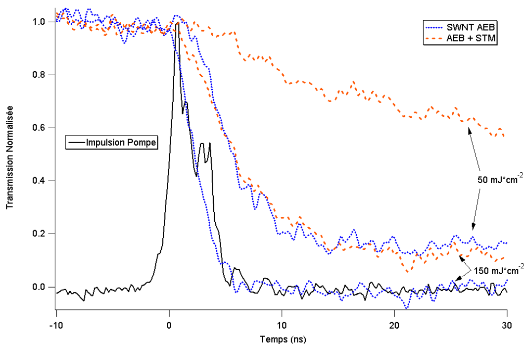
FIG. 6.25: Comparaison des transmissions de la sonde à 50 et 150 \text{mJ}\cdot\text{cm}^{-2} pour les nanotubes AEB et le mélange nanotubes / STM. Pompe à 532 nm, 4 ns.
