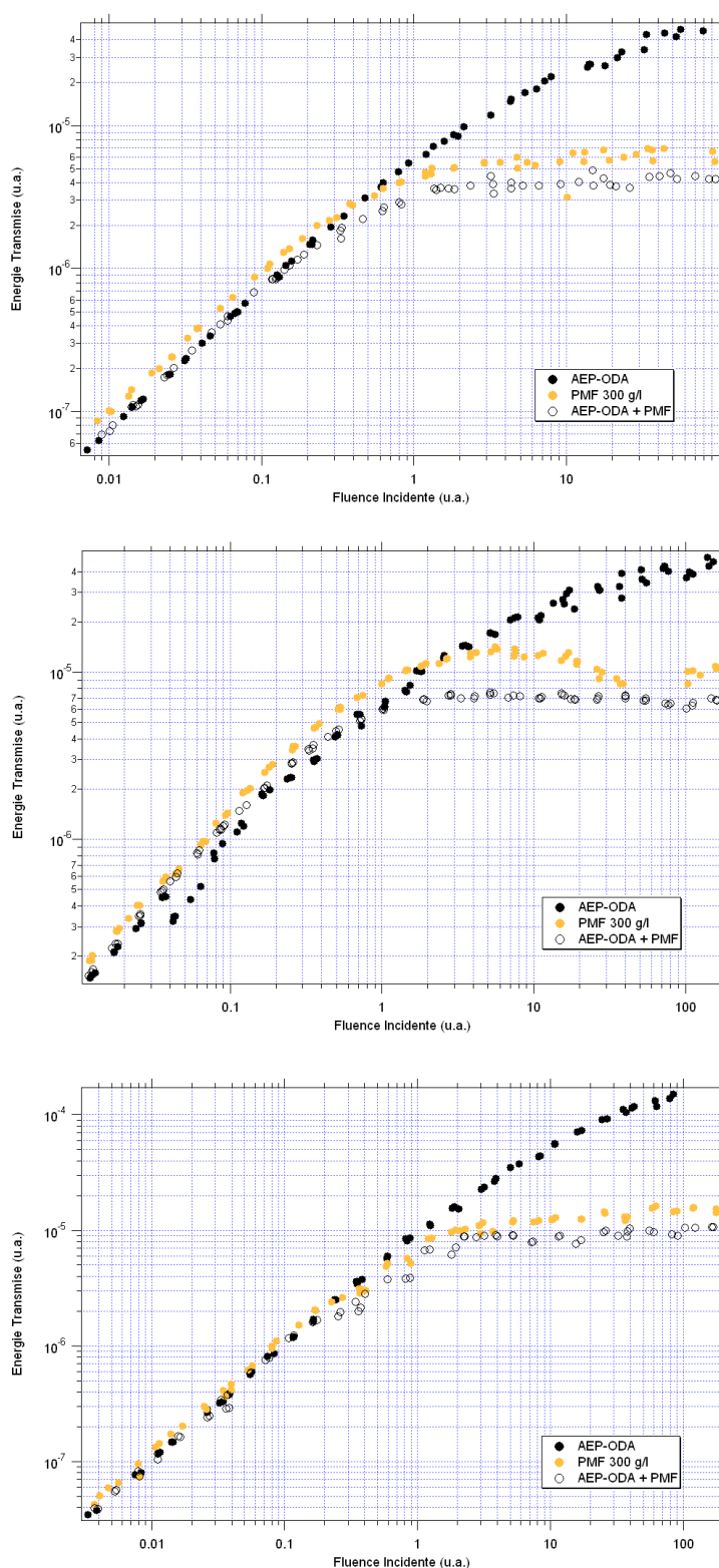
FIG. 6.30: Comparaison des énergies transmises pour une suspension de nanotubes AEP-ODA, une solution de PMF à 300 g·l -1 et la combinaison des deux limiteurs au sein de la même cuve, à 490 (haut), 532 (milieu), et 590 (bas) nm, 4 ns. Les échelles ont été normalisées par un facteur arbitraire.
