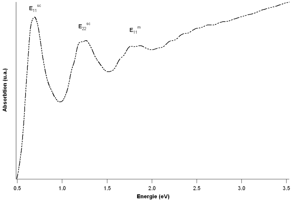
FIG. 3.10: Exemple de spectre expérimental d'absorption optique de nanotubes de carbone. Les bandes d'absorption E_{11}^{sc} , E_{22}^{sc} et E_{11}^m sont indexées.
