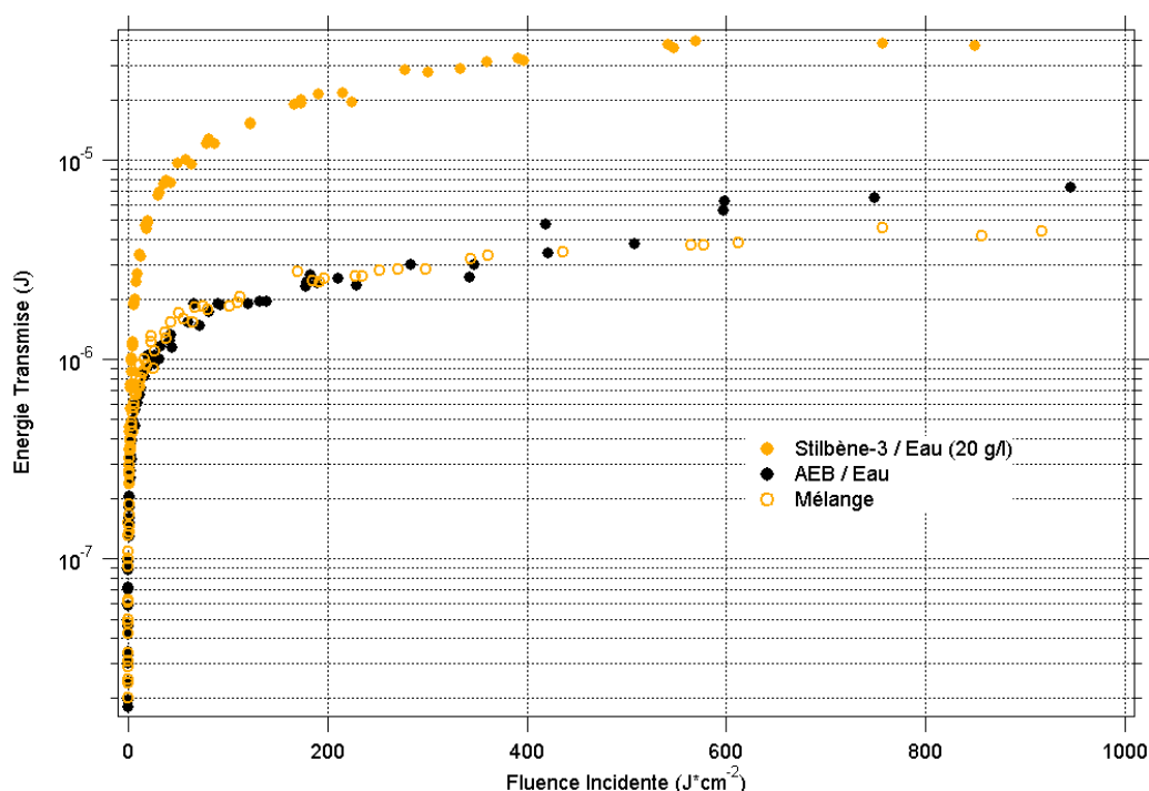
FIG. 6.20: Courbes de limitations optique sur banc OTAN, à 532 nm et 7 ns. Énergie transmise en fonction de la fluence incidente. Échantillons : stilbène-3 dans l'eau, nanotubes AEB dans l'eau et mélange nanotube / stilbène-3.
