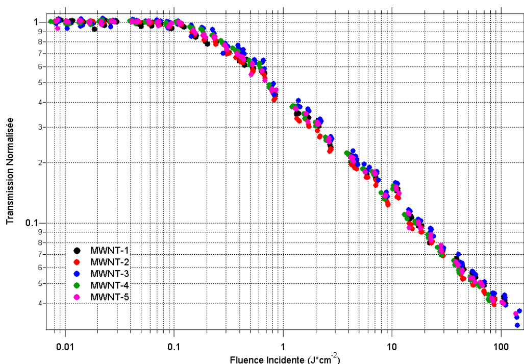
FIG. 6.7: Courbes de limitation optique en petite ouverture à 532 nm. Durée d'impulsion 15 ns. Echantillons MWNT-1, MWNT-2, MWNT-3, MWNT-4 et MWNT-5 en suspension dans l'eau.
