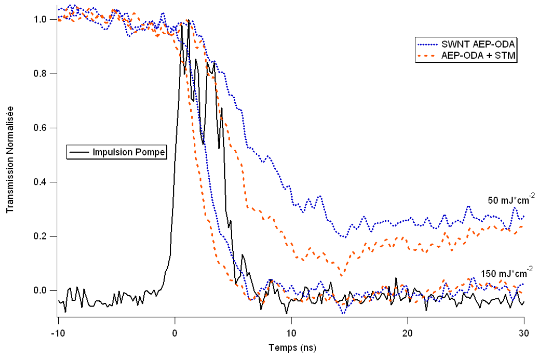
FIG. 6.27: Comparaison des transmissions de la sonde à 50 et 150 mJ·cm -2 pour les nanotubes AEP-ODA et le mélange AEP-ODA / STM. Pompe à 532 nm, 4 ns.
