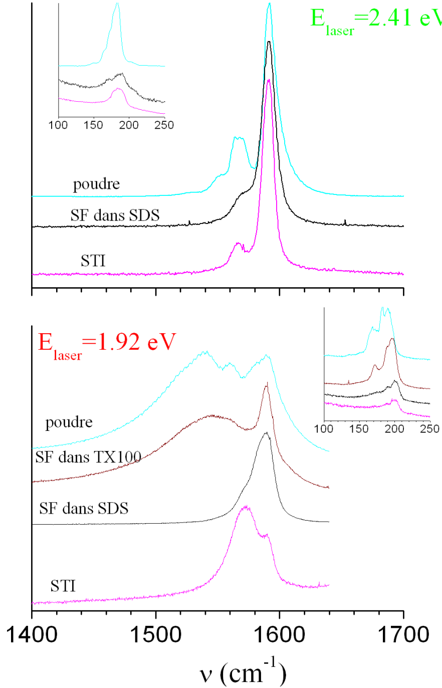
FIG. 5.11: Modes TM de la poudre, des suspensions de fagots (SF) avec le SDS et le triton X-100, et des suspensions de tubes individualisés (STI) pour l'échantillon AEP à 1,92 et 2,41 eV. Les spectres sont normalisés et déplacés le long de l'axe vertical. Les spectres RBM correspondants sont représentés en insert.
