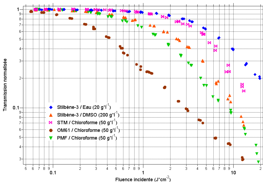
FIG. 6.23: Courbes de limitation optique des solutions d'absorbeurs à deux photons. Banc petite ouverture, 532 nm, durée d'impulsion 15 ns.
