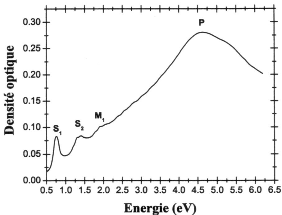
FIG. 1.13: Spectre d'absorption optique de dépôt de nanotubes. S_1 et S_2 : bandes semiconductrices ; M_1 : bande métallique ; P : raie plasmon
