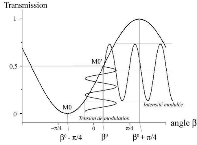
Figure III-17 : Principe de la modulation électro-optique en régime dynamique
