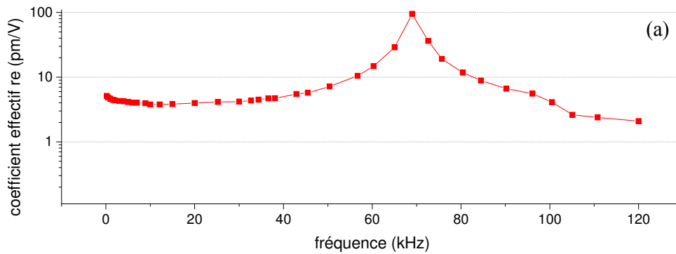
Figure IV-50 : Evolution en fréquence du paramètre r_e (PM1814A)
