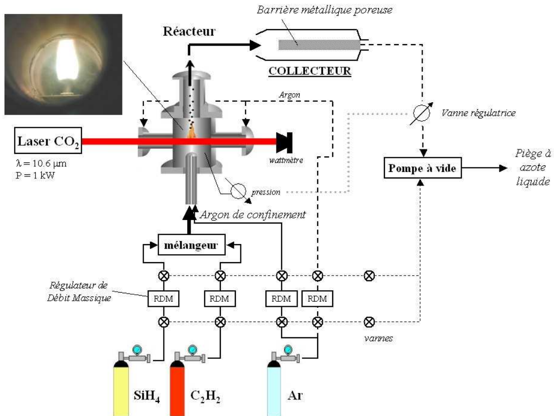
Figure II-1 : Dispositif expérimental de pyrolyse laser en phase gazeuse
