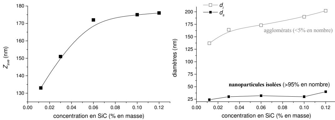
Figure IV-29 : Effet de concentration sur la dispersion – SiC 237 bs dans l'eau
