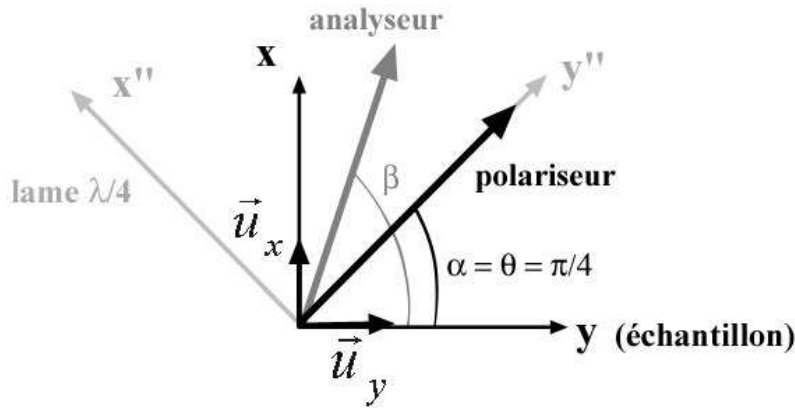
Figure III-15 : Orientation des axes et des composants optiques
