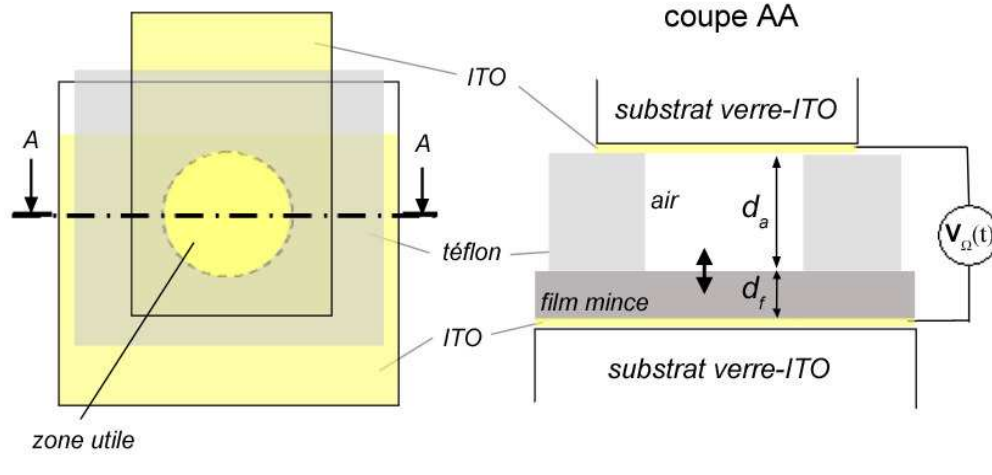
Figure IV-56 : Schéma du dispositif sandwich ITO/composite/air/ITO
