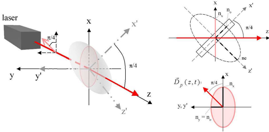
Figure III-13 : Configuration à 45° pour la caractérisation électro-optique des films minces
