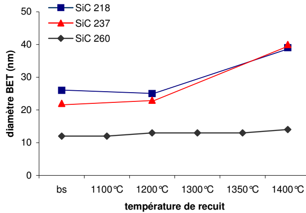
Figure IV-1 : Evolution des diamètres BET en fonction du recuit
