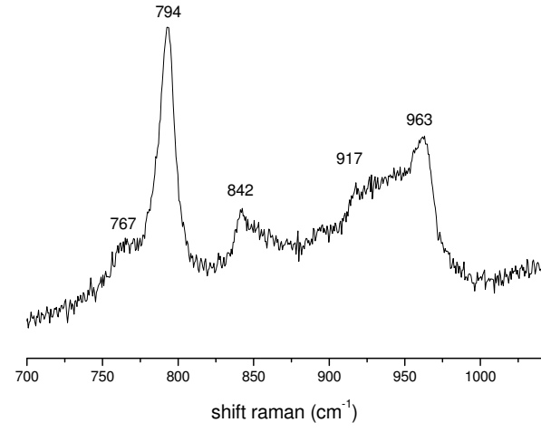
Figure IV-20 : Spectre Raman résolu de la bande Si-C (SiC 237/1400°C)
