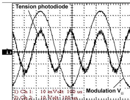
Figure IV-55 : Modulation à la fréquence double
