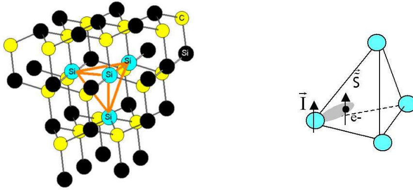
Figure IV-25 : Site tétraédrique d'une lacune chargée dans l'environnement SiC (défaut DI)
