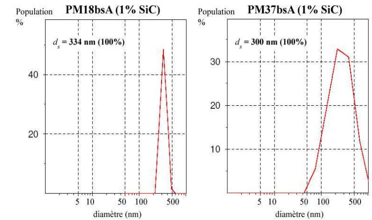
Figure IV-36 : Distributions de tailles des nanopoudres brutes dans PMMA et chloroforme
