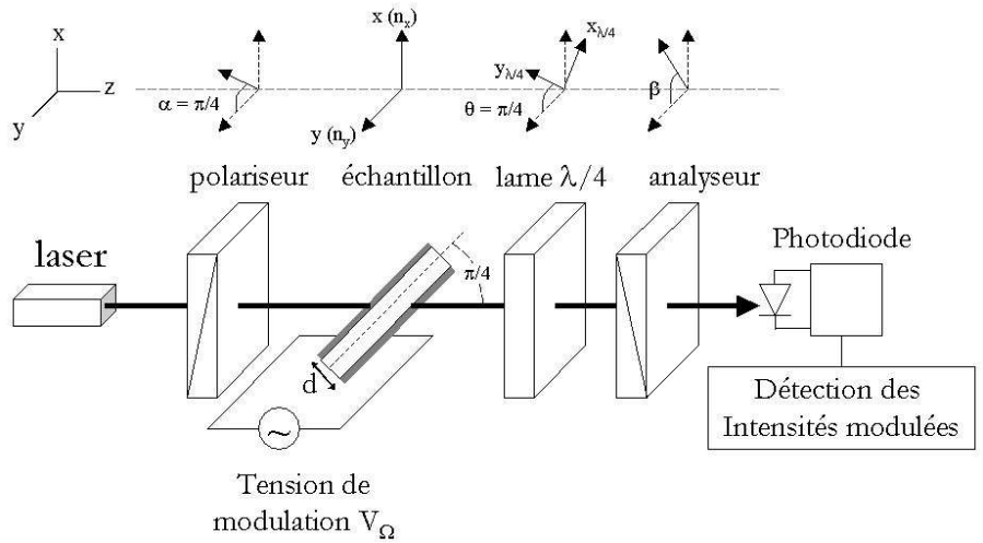
Figure III-18 : Principe de la mesure par la méthode de Sénarmont en régime dynamique
