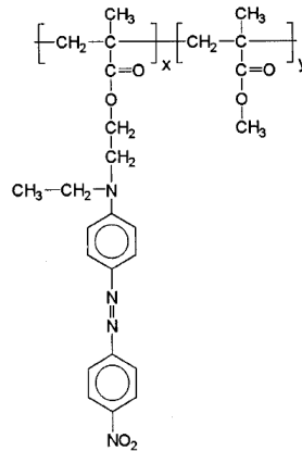
Figure I-5 : Structure du copolymère DRI-MMA/MMA
