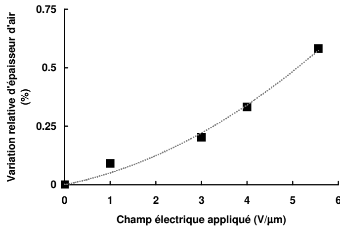
Figure IV-52 : Variation relative du chemin optique dans la couche d'air en fonction de la tension appliquée
