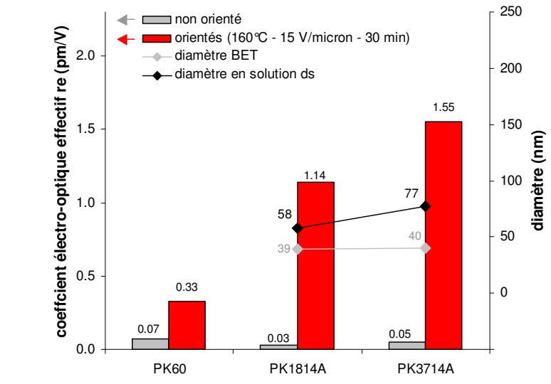
Figure IV-68 : Paramètres r_e et diamètres caractéristiques pour le système SiC-PVK
