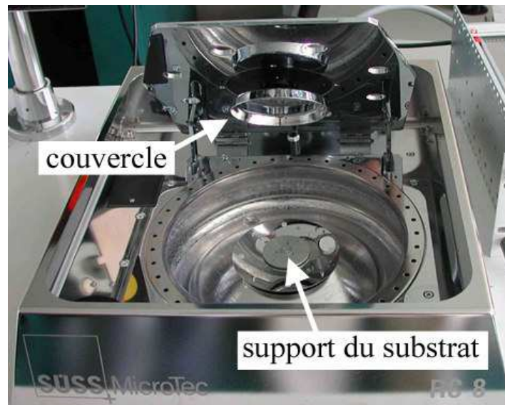
Figure II-3 : le dispositif de dépôt des films minces : le spin-coater
