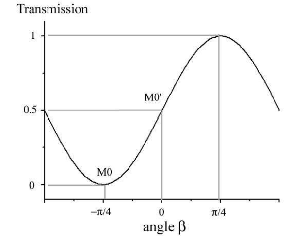
Figure III-16 : Transmission du montage de Sénarmont en fonction de l'angle de l'analyseur
