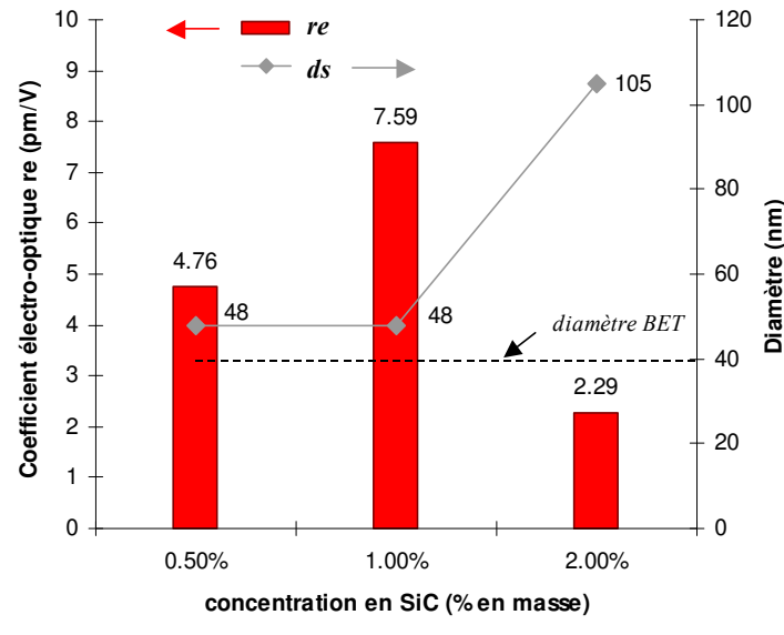
Figure IV-62 : Corrélation entre les diamètres des particules en solution et le coefficient r_e
