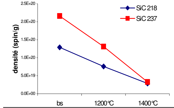
Figure IV-23 : Densité en défauts paramagnétiques en fonction du recuit
