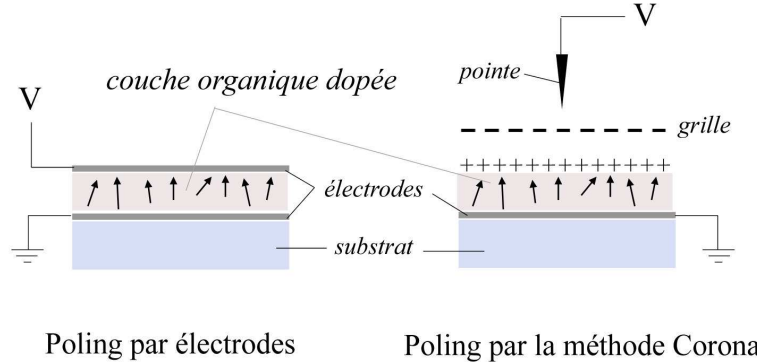
Figure I-4 : Principe des procédures de poling par électrode et par la méthode corona
