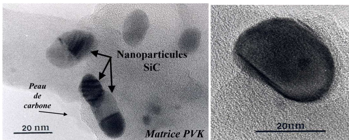
Figure IV-43 : Images MET de particules de SiC 218 dans PVK [Bouclé02]
