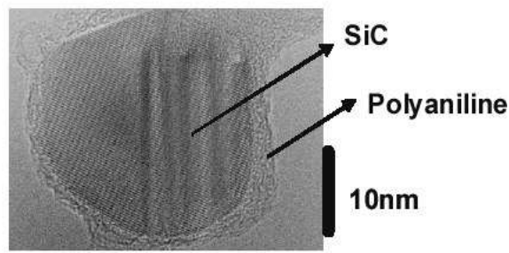
Figure b : Particule de SiC fonctionnalisée enrobée par la polyaniline
