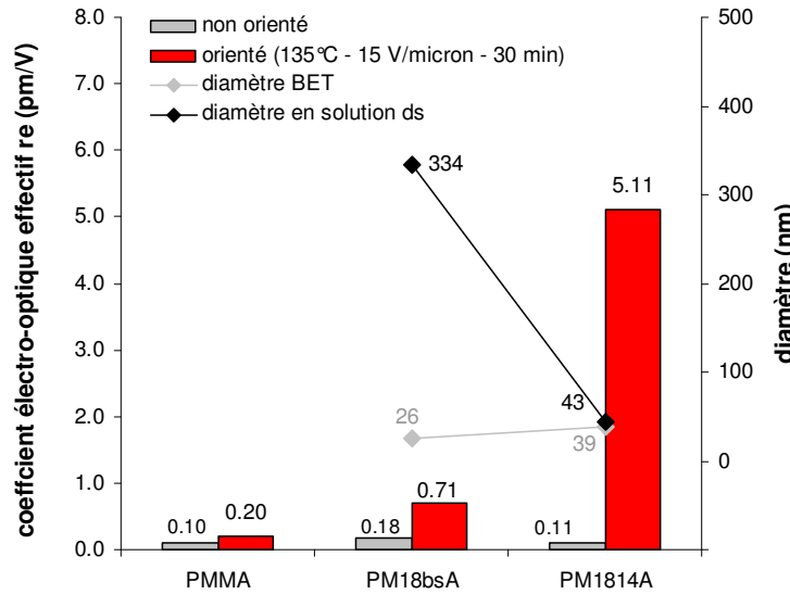
Figure IV-65 : Paramètre électro-optique linéaire r_e des films à base de SiC 218 dans PMMA
