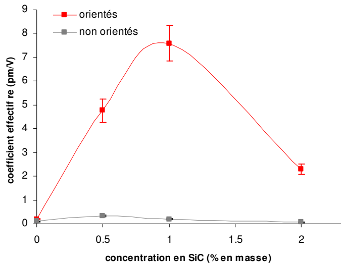
Figure IV-61 : Effet de concentration sur r_e (PMMA-SiC237/1400°C)
