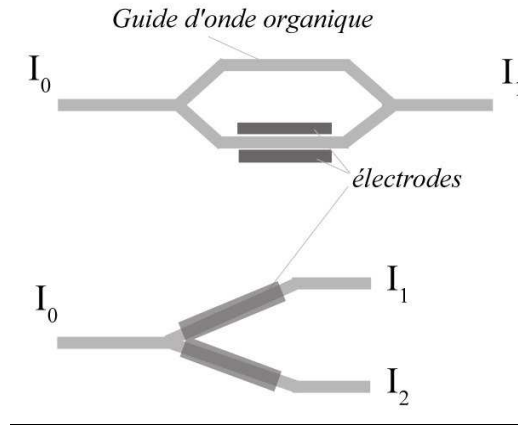
Figure I-7 : Structures typiques de modulateurs organiques (Mach-Zehnder en haut, Y-branch en bas)
