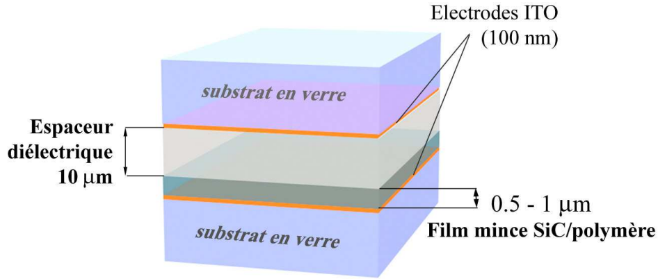
Figure II-5 : Structure des échantillons sandwich ITO/composite/espaceur/ITO
