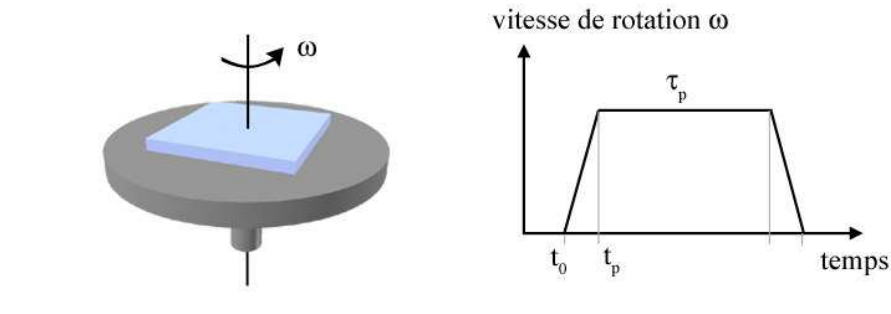
Figure II-2 : Principe du dépôt de films minces par spin-coating
