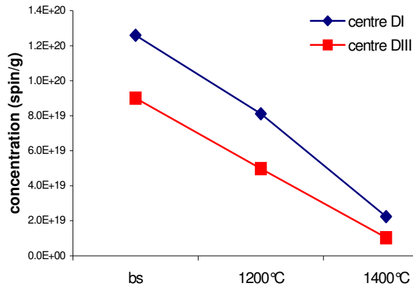
Figure IV-26 : Teneur en défauts DI et DIII au cours du recuit (SiC237)
