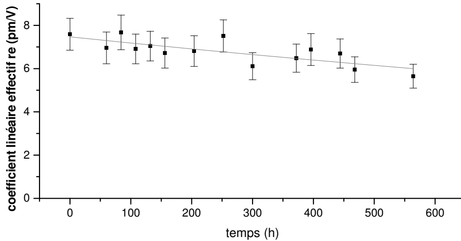
Figure IV-71 : Evolution dans le temps du paramètre r_e (PMMA-SiC237/1400°C 1%)
