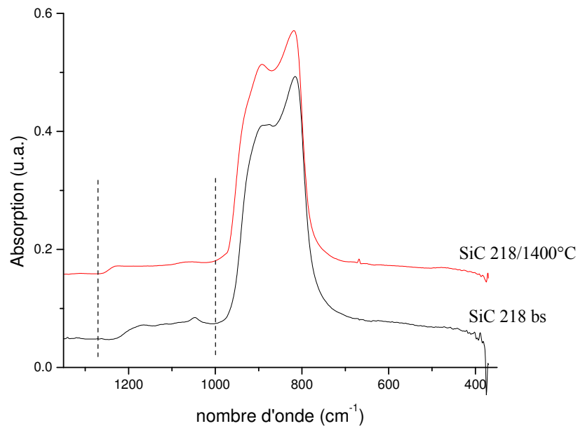
Figure IV-16 : Spectres infrarouges du SiC 218 brut et recuit à 1400^\circ\text{C}
