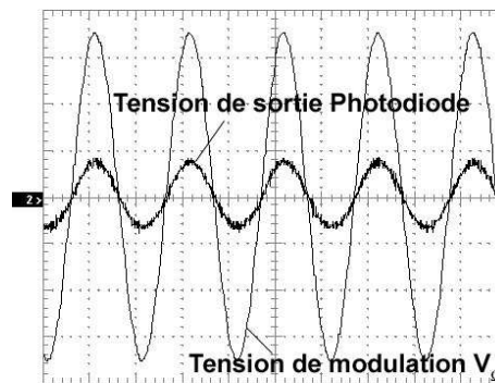
Figure IV-49 : Capture d'écran d'oscilloscope (PMMA/1% SiC 218/1400°C) ( f=1\text{kHz} , V_m=16 \text{ V} – CH1(Photodiode)=2mV/div, CH2( V_\Omega )=5V/div, 500 \mu\text{s} /div)
