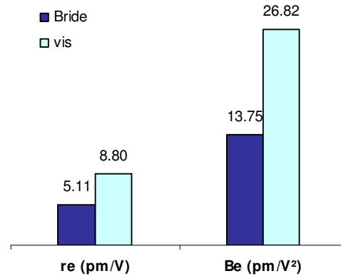
Figure IV-54 : Influence du support sur la modulation électro-optique
