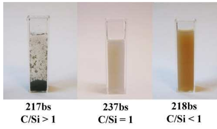
Figure IV-27 : Dispersion dans l'eau – 1 minute de sonification (amplitude de 35%)
