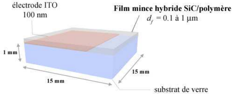
Figure II-4 : Structure des échantillons après dépôt par spin-coating
