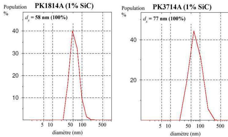
Figure IV-40 : Distributions de taille des solutions SiC/PVK/chloroforme
