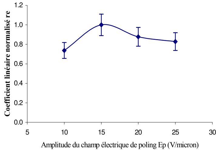
Figure IV-47 : Effet de la tension de poling sur le coefficient r_e des films minces à base de PMMA
