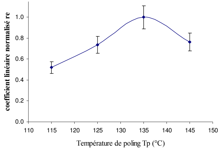
Figure IV-48 : Effet de la température de poling sur le coefficient r_e des films minces à base de PMMA
