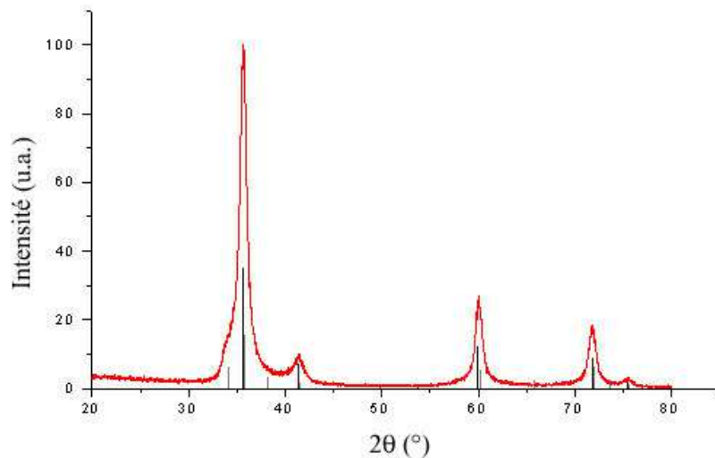
Figure IV-8 : Spectre DRX de l'échantillon SiC 237 bs
