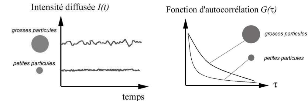
Figure III-7 : Intensité diffusée et fonction d'autocorrélation pour différentes tailles de particules
