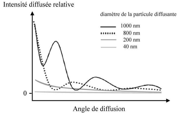
Figure III-6 : Lumière diffusée par des particules de différentes tailles (théorie de Mie)
