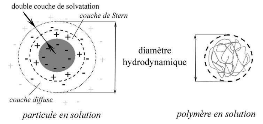
Figure III-8 : Notion de diamètre hydrodynamique
