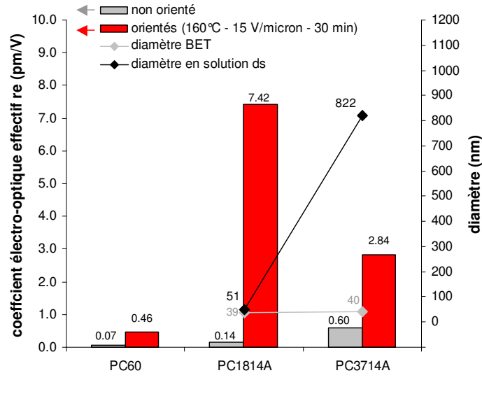
Figure IV-67 : Paramètres r_e et diamètres caractéristiques pour le système SiC-PC (1%)
