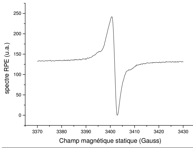
Figure IV-22 : Spectre RPE de l'échantillon SiC 237/1400°C en bande X à 300K
