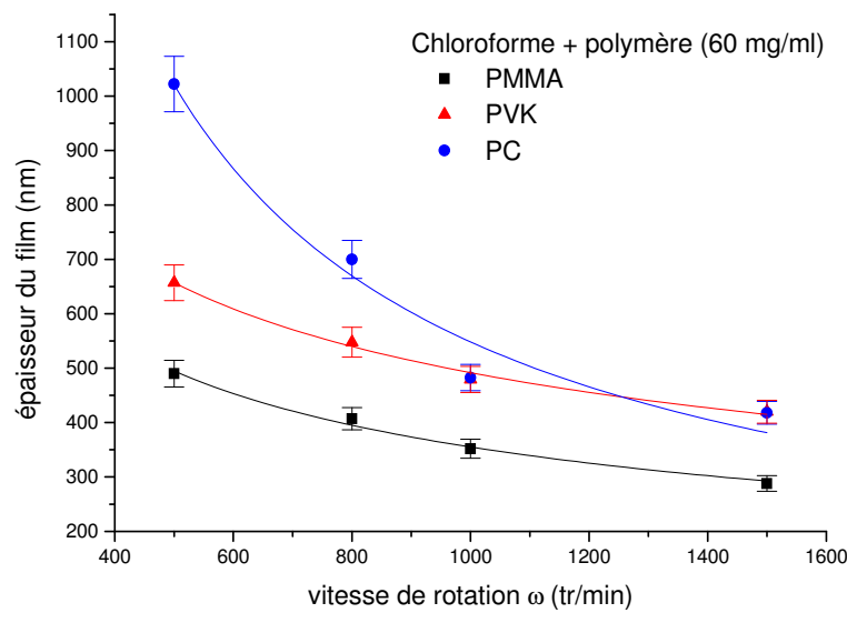
Figure IV-41 : Epaisseurs des films en fonction de la vitesse de dépôt
