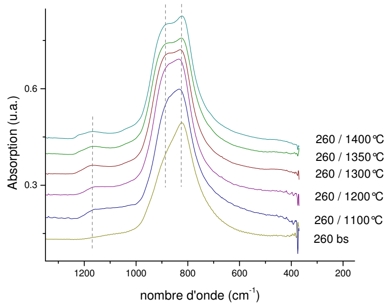
Figure IV-17 : Spectres infrarouges de l'échantillon SiC 260 en fonction du recuit
