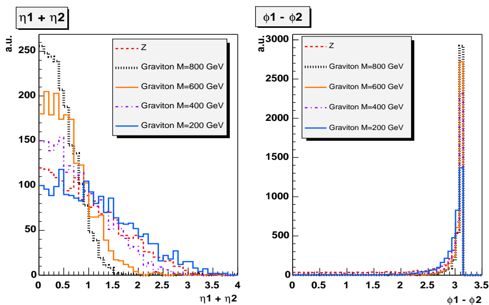
FIG. 4.16 – Distributions angulaires entre les deux muons issus de la désintégration d'un Z et de gravitons de masse 200 GeV, 400 GeV, 600 GeV et 800 GeV. La figure de gauche montre la somme des valeurs de \eta des deux muons, la figure de droite montre la différence en \phi entre les deux muons.
