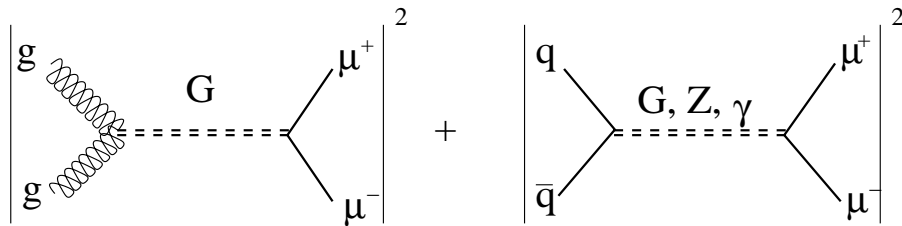
FIG. 2.5 – Diagrammes de Feynman des processus étudiés pour la production résonante de graviton de Kaluza-Klein. Le processus faisant intervenir des quarks dans l'état initial interfère avec la production dimuons via un boson \gamma ou Z , ce qui n'est pas le cas pour le processus dû à la fusion de gluons.
