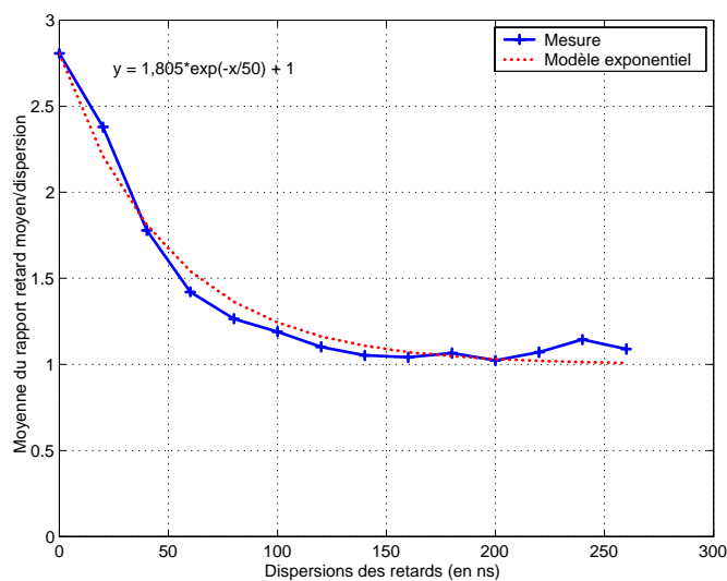
FIG. 7.33 – Moyenne du rapport de forme (retard moyen/dispersion des retards) de la loi gamma
