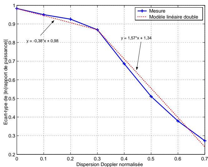
FIG. 7.44 – Ecart-type de la valeur absolue du logarithme du rapport des puissances de chacune des lois de VM associées au modèle VM double - Premiers groupes
