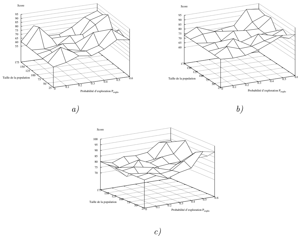
FIG. 5.2 – Influence conjointe de la taille de Pop_G et de P_{expl} pour l'algorithme GeniminerII pour la requête 1 sur les a) 30, b) 60, c) 100 premiers résultats obtenus au bout de 1000 téléchargements.
