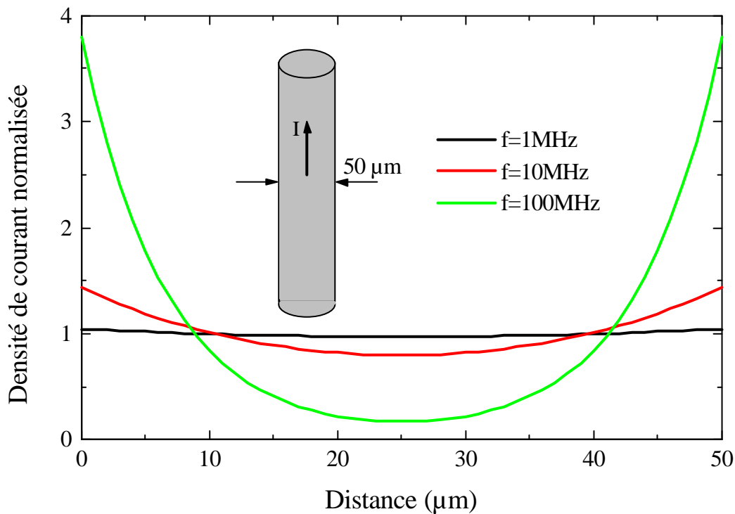
Figure 2.2 : Distribution de courant à l'intérieur d'un fil cylindrique de cuivre de 50 μm d'épaisseur (section transversale) à température ambiante pour 3 différentes fréquences.
