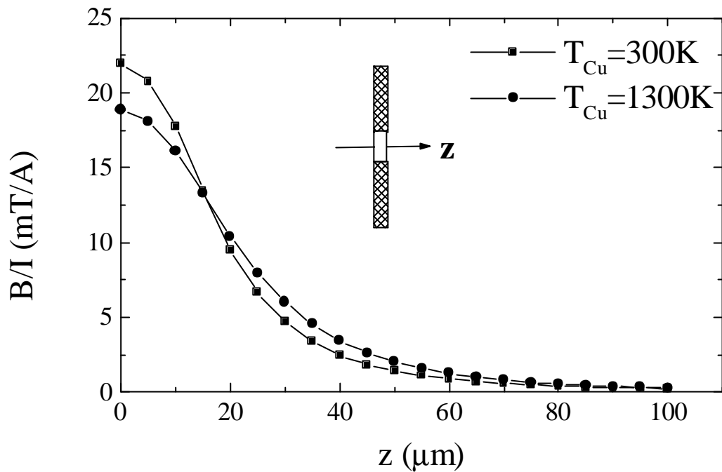
Figure 3.9 : Simulation du champ B au long de l'axe z de la bobine pour deux températures différentes. Les dimensions de la bobine sont, diamètre interne 50\mu\text{m} , diamètre externe 150\mu\text{m} , épaisseur du cuivre 30\mu\text{m} ( z=0 est au centre de la bobine).
