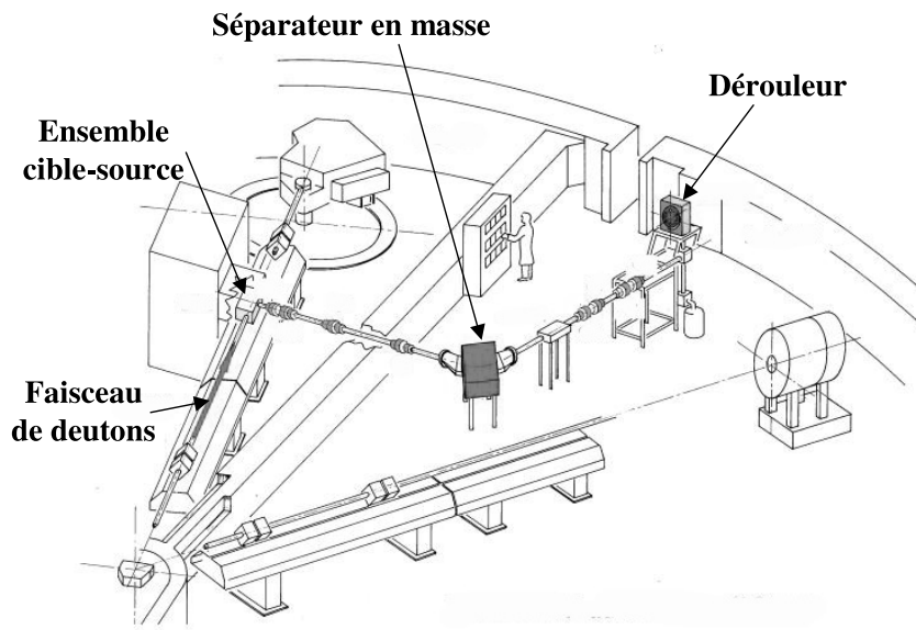
FIG. 3.7 – Schéma de PARRNe au Tandem d'Orsay.
