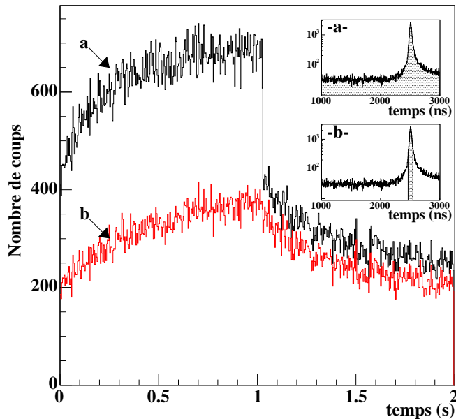
FIG. 3.19 – Projections en temps de la matrice "énergie-énergie" réalisée avec une fenêtre de coincidence \beta - \gamma de 2 \mu\text{s} (insert a), et de 70 ns (insert b).
