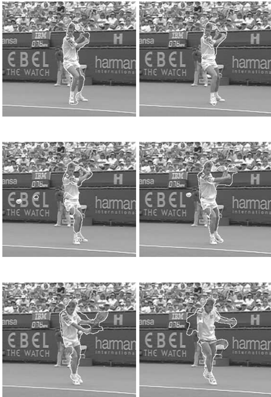
FIG. 4.10: Résultats de notre méthode de segmentation par flot optique pour les paramètres suivants : \alpha = 1 , \lambda = 5 , \nu = 1 . Les mouvements non rigides ne favorisent pas l'utilisation de cette méthode. L'emploi d'un flot optique obtenu avec multirésolution permet toutefois d'obtenir un résultat certes approximatif, mais qui peut se combiner avec d'autres algorithmes.
