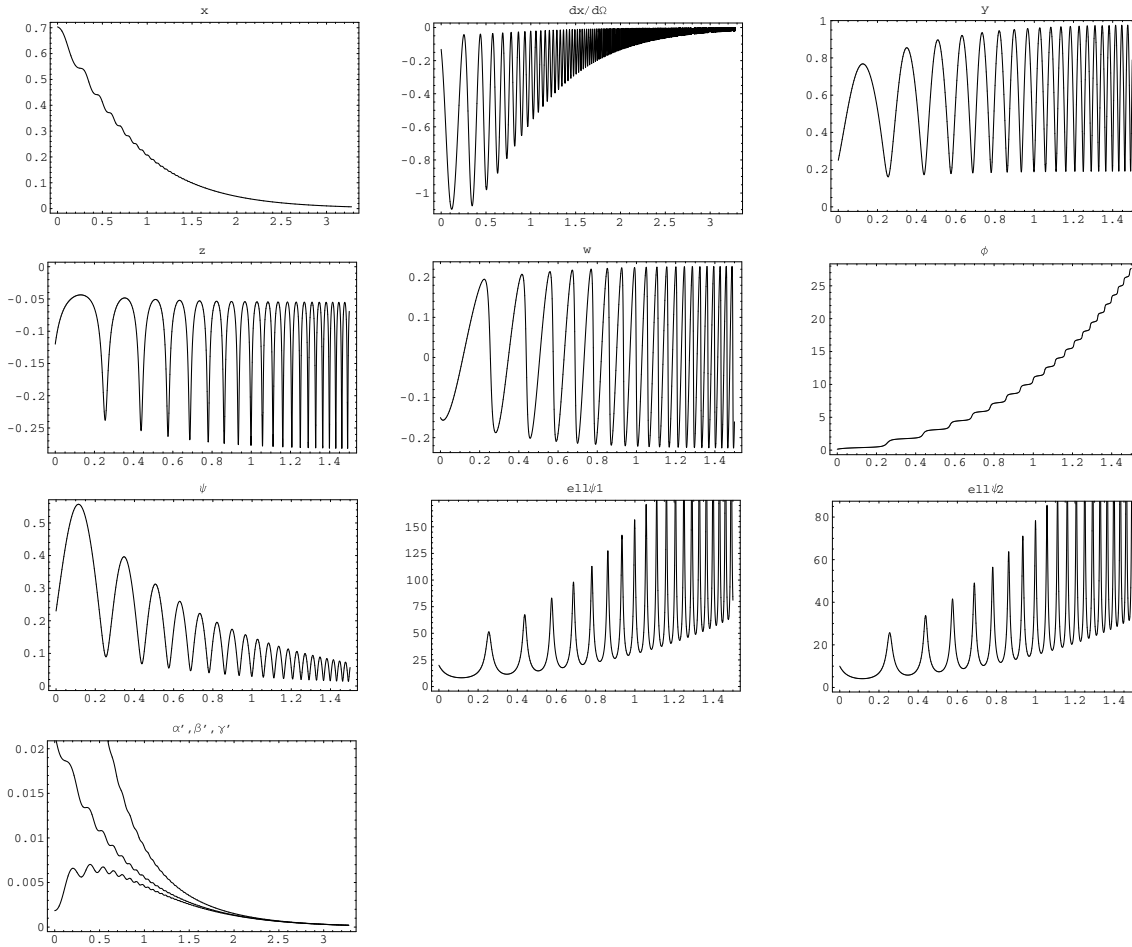
FIG. 1.6 – Ces figures, avec -\Omega en abscisse, représente successivement les comportements de (x, \dot{x}, y, z, w, \phi, \psi, \ell_{\psi_2}) pour les conditions initiales (x, y, z, w, \phi, \psi) = (-0.70, 0.25, -0.12, -0.15, 0.14, 0.23) et le paramètre m = -2.3 . x est la seule variable à atteindre l'équilibre alors que y, z et w oscillent de plus en plus lorsque -\Omega \rightarrow +\infty . Le champ scalaire subit des oscillations amorties alors que les oscillations de \ell_{\phi_2} et \ell_{\psi_2} augmentent. La dernière figure montre la disparition des dérivées de \alpha, \beta et \gamma par rapport au temps propre. Notons qu'elles oscillent.
