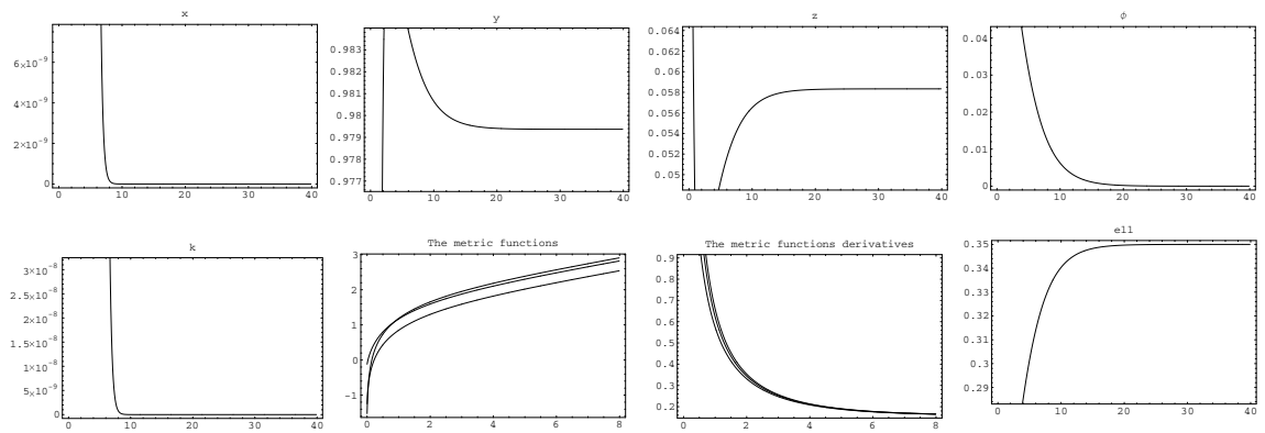
FIG. 1.16 – Ces figures représentent l'approche des variables pour une isotropisation de classe 1 lorsque \omega = 2.3 , \omega_1 = 0.5 , n = -3.1 , m = 1.1 et p = 0.7 . k et \phi tendent vers zéro. \ell tend vers 0.35 ce qui est plus petit que 3/2\gamma = 3/2
