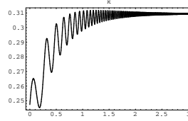
FIG. 1.7 – Si l'on prend en compte un fluide parfait, k peut atteindre une constante durant l'isotropisation.
