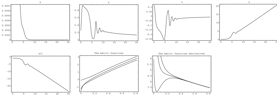
FIG. 1.10 – Ces figures représentent l'approche des variables pour une isotropisation de classe 2 lorsque \omega_0 = 2.3 , n = -3.1 et m = 1.1 . x tend toujours vers zéro mais y aussi. \phi et donc \ell diverge. Notons que \phi , y , z et \ell subissent des oscillations amorties. Dans le référentiel de Brans-Dicke, les dérivées des fonctions métriques \alpha , \beta et \gamma tendent vers une fonction commune, montrant l'isotropisation.
