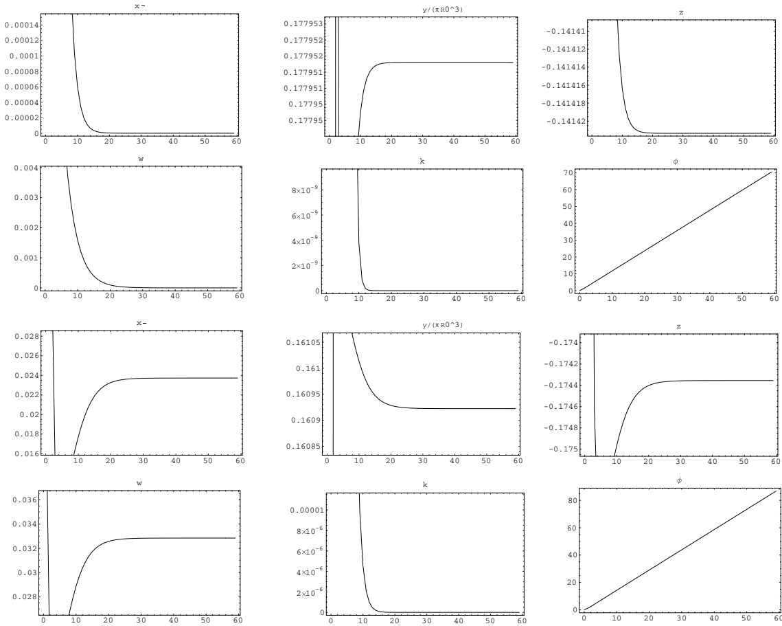
FIG. 2.1 – Evolution des variables x , y et z lorsque \frac{(3+2\omega)^{1/2}}{\phi} = \sqrt{2} , U = e^{m\phi} , R_0^3 = (\sqrt{24}\pi)^{-1} avec les valeurs initiales (x_+, x_-, y, z, w, \phi) = (0.87, 0.06, 0.025, -0.12, 0.065, 0.014) . Les 6 premières figures sont telles que m = -1.2 (l'évolution de x_+ est semblable à celle de x_- ): l'Univers s'isotropise. La deuxième série de 6 figures est telle que m = -1.5 : l'Univers ne s'isotropise plus.
