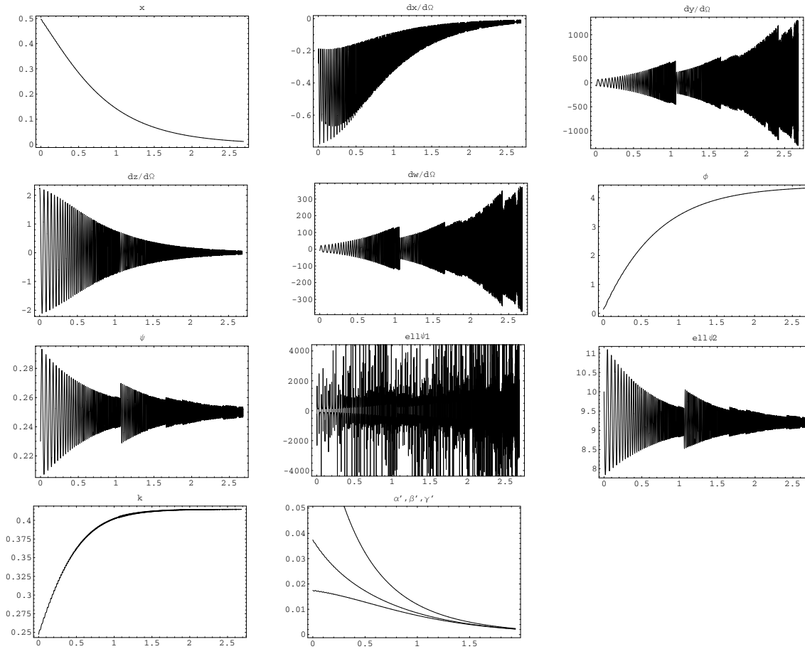
FIG. 1.8 — Ces figures, avec -\Omega en abscisse, représentent successivement les comportements de (x, \dot{x}, \dot{y}, \dot{z}, \dot{w}, \phi, \psi, \ell_{\psi_1}, \ell_{\psi_2}) pour les valeurs initiales (x, y, z, w, \phi, \psi) = (0.49, 0.25, -0.12, -0.15, 0.14, 0.23) et les paramètres (\lambda, \eta) = (0.25, 0.25) . x, z et le champ scalaire atteignent l'équilibre alors que \ell_{\psi_1} subit des oscillations non amorties. La dernière figure montre la disparition des dérivées de \alpha, \beta et \gamma par rapport au temps propre.
