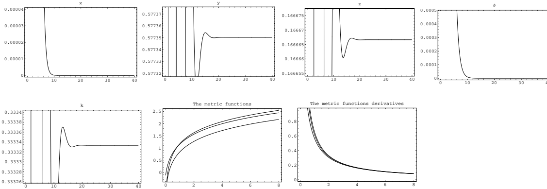
FIG. 1.15 – Ces figures représentent l'approche des variables pour une isotropisation de classe 1 lorsque \omega = 2.3 , \omega_1 = 0.5 , n = -3.1 , m = 1.1 et p = 3 . k oscille vers une constante et \phi tend vers zéro. Notons les fortes oscillations de y , z et k .
