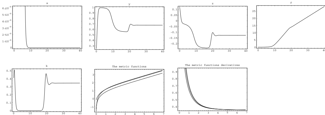
FIG. 1.13 — Ces figures représentent l'approche des variables pour une isotropisation de classe 1 lorsque \omega_0 = 2.3 , n = -3.1 et m = 1.1 . k tend vers une constante mais nous remarquons également l'existence, avant l'équilibre, d'une période durant laquelle le paramètre de densité du fluide parfait est quasiment nul.
