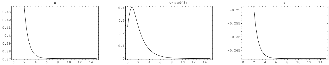
FIG. 1.2 – Evolution des variables x , y et z lorsque \frac{(3+2\omega)^{1/2}}{\phi} = \sqrt{2} , U = e^{m\phi} , R_0^3 = (\sqrt{24}\pi)^{-1} et m = -3.2 avec les valeurs initiales (x, y, z, \phi) = (0.87, 0.25, -0.12, 0.14) . L'Univers ne s'isotropise pas: le système tend vers un point d'équilibre anisotrope tel que les fonctions \underline{g} décrivant l'anisotropie divergent.
