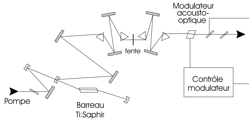
FIG. 2.7 – Schéma de l'oscillateur titane:saphir ( Tsunami Spectra Physics ).
