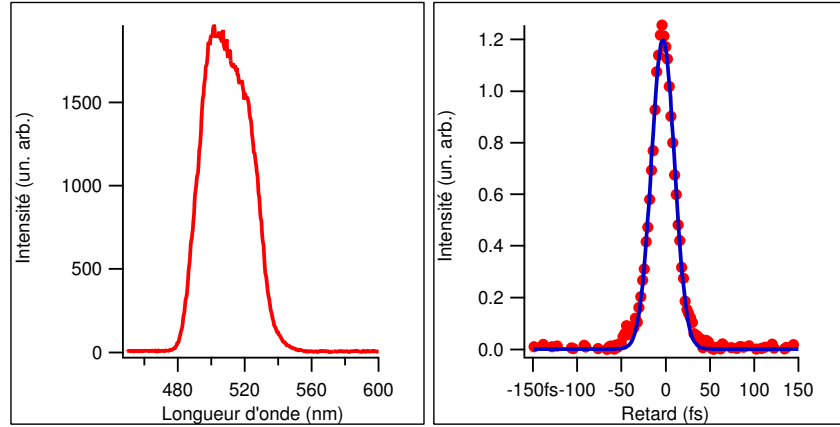
FIG. 2.24 – Autocorrélation en intensité (point à droite) obtenue pour une impulsion centrée autour de 505 nm (à gauche) (BBO type I, \theta=45.3^\circ , L=100 \mu\text{m} ). La courbe en trait plein est un fit gaussien avec un durée d'impulsion de 20 fs.
