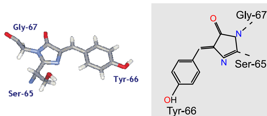
FIG. 1.2 – Structure chimique du chromophore GFP ( p -hydroxybenzylimidazolinone) mise en évidence par Shimomura en 1979 [Shi79].
