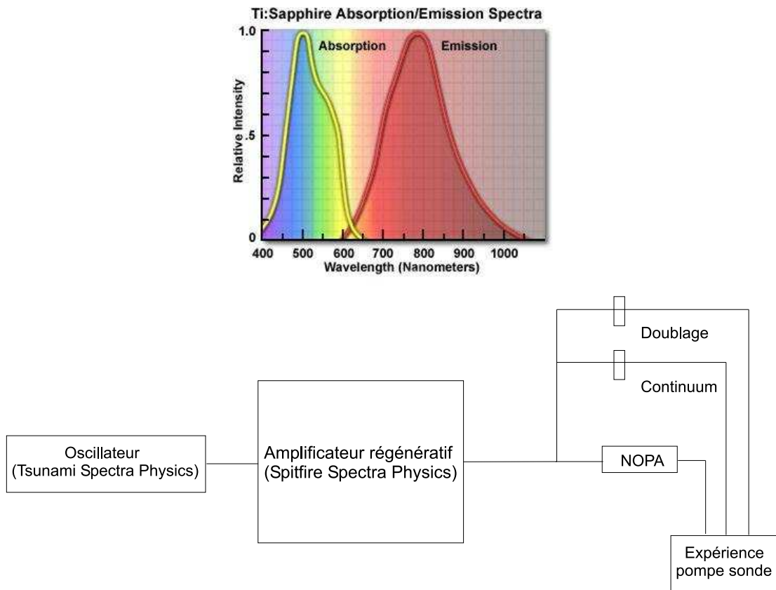
FIG. 2.6 – En haut, spectre d'absorption et d'émission d'un barreau de saphir dopé aux ions Ti^{3+} (site web d'Olympus © ). En bas, schéma général du montage expérimental.
