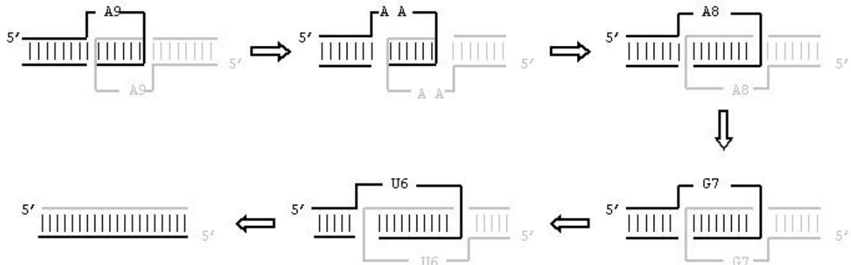
Figure 18 : Modèle de transition entre le dimère instable et le dimère stable suggéré par Beaurain et al. (2003) et consistant en une élévation de l'hélice boucle-boucle du dimère instable.
