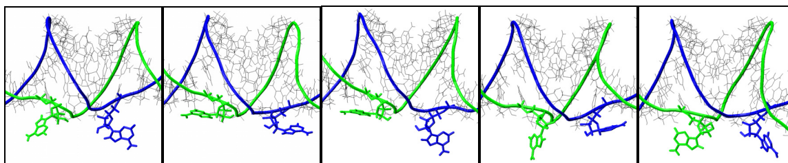
Figure 80 : Images instantanées des configurations prises par les résidus A8 (en bleu) et A8' (en vert) au cours de la simulation du dimère de Ennifar et al. (1999).
