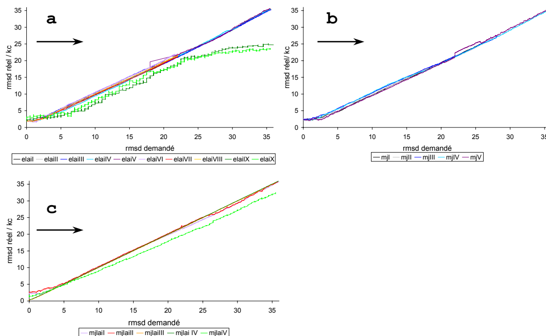
Figure 97 : Evolution des valeurs de \rho(\text{KC}) en fonction \rho_0(\text{KC}) pour les TMD -1 à partir des structures initiales X-ray_KC Lai (a), NMR_KC LaiΔ (b) et NMR_KC Lai (c). La flèche noire donne le sens de la simulation.
