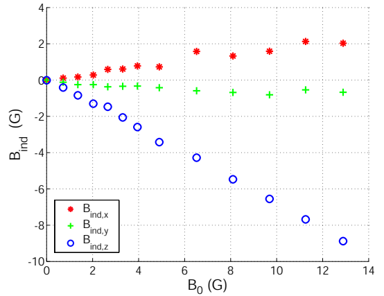
(d) \vec{B}_0 transverse, \Omega = 17 Hz
