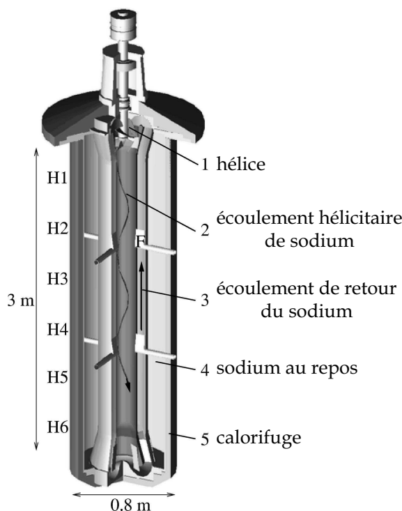
Fig. I.10: L'expérience dynamo de Riga.
