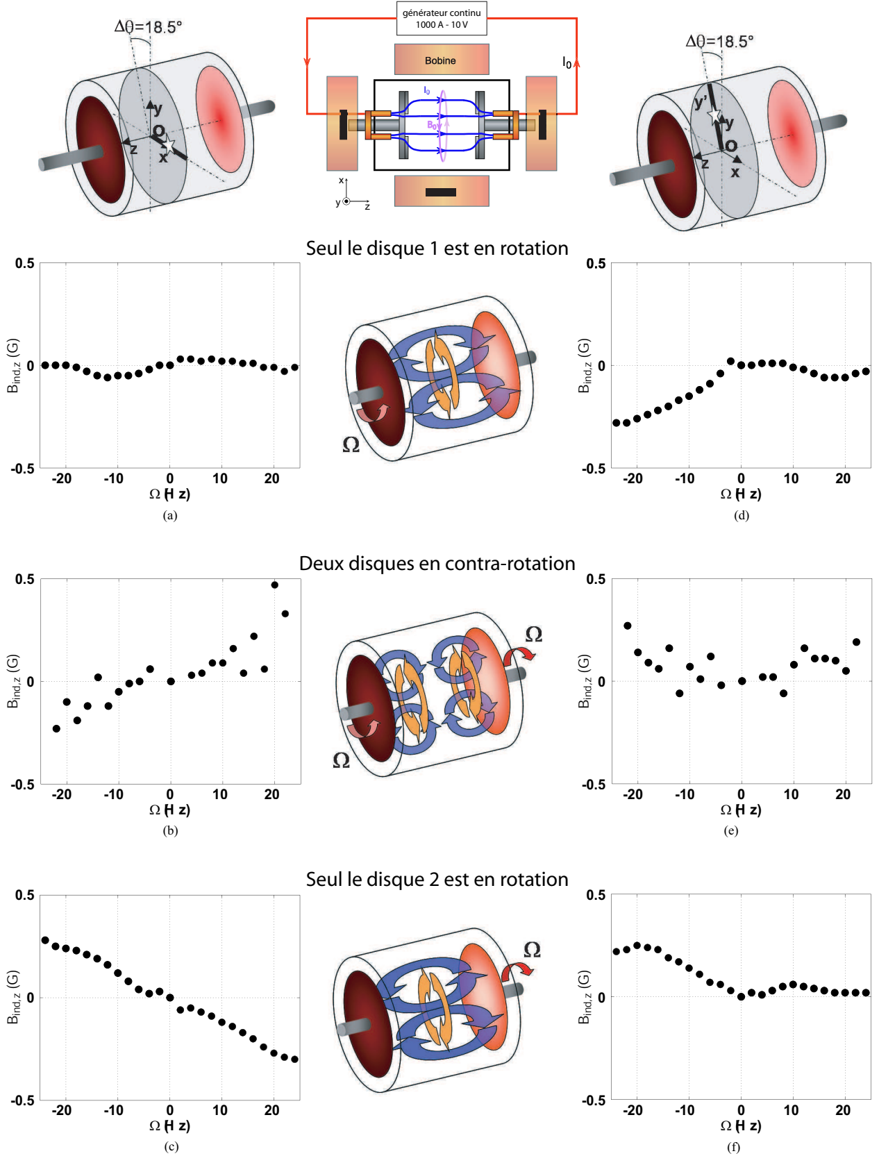
Fig. IV.37: Mesures d'induction magnétique axiale en présence d'un champ appliqué azimuthal. Les figures a,b et c correspondent à des mesures faites au point (r = 0.5R, \theta = 0, z = 0) de l'axe Ox et les figures d,e et f à des mesures faites au point (r = 0.5R, \theta = 108.5^\circ, z = 0) de l'axe Oy' proche de Oy .
