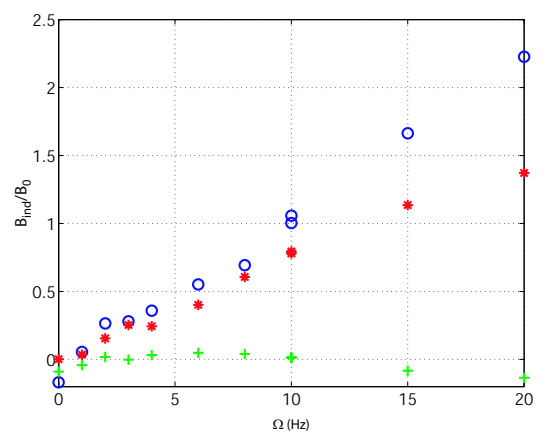
(b) mesure au point (x = 0, y = 4 \text{ cm}, z = 0)
