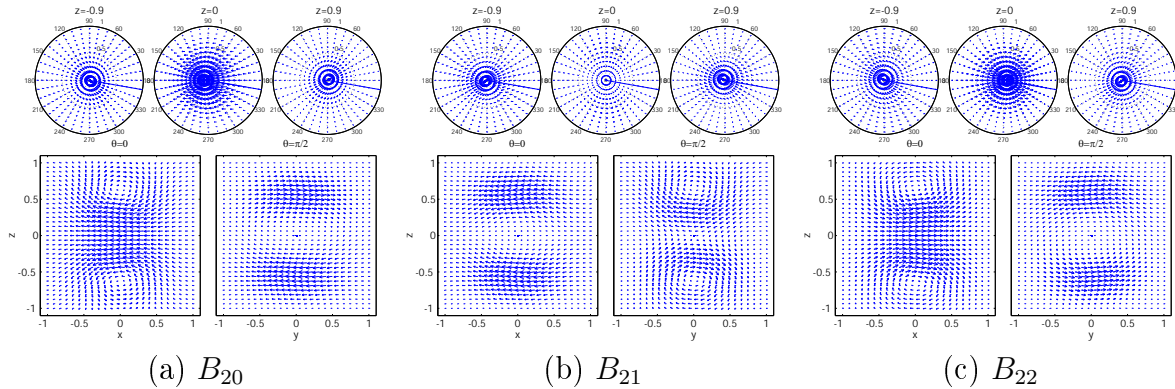
Fig. III.57: Schéma de bouclage en deux étapes : \vec{B}_{20} \propto -\vec{B}_{22} .
