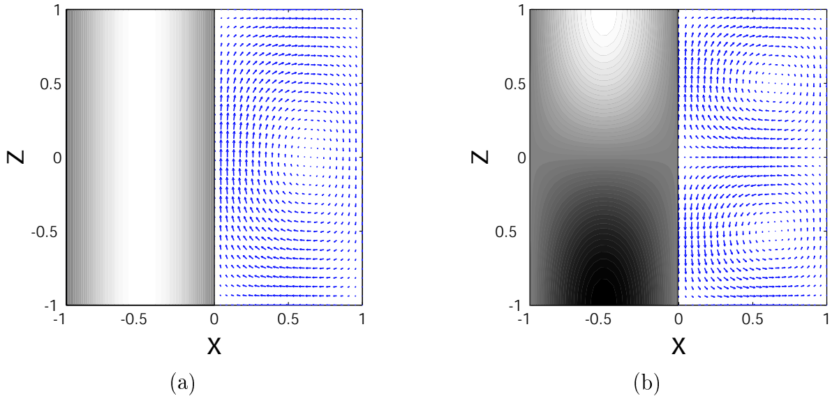
Fig. II.8: Champ de vitesse modèle pour les écoulements de von Kármán à un disque en rotation et deux disques contra-rotatifs. Les contours représentent la composante azimutale de la vitesse (négative en sombre et positive en clair.)
