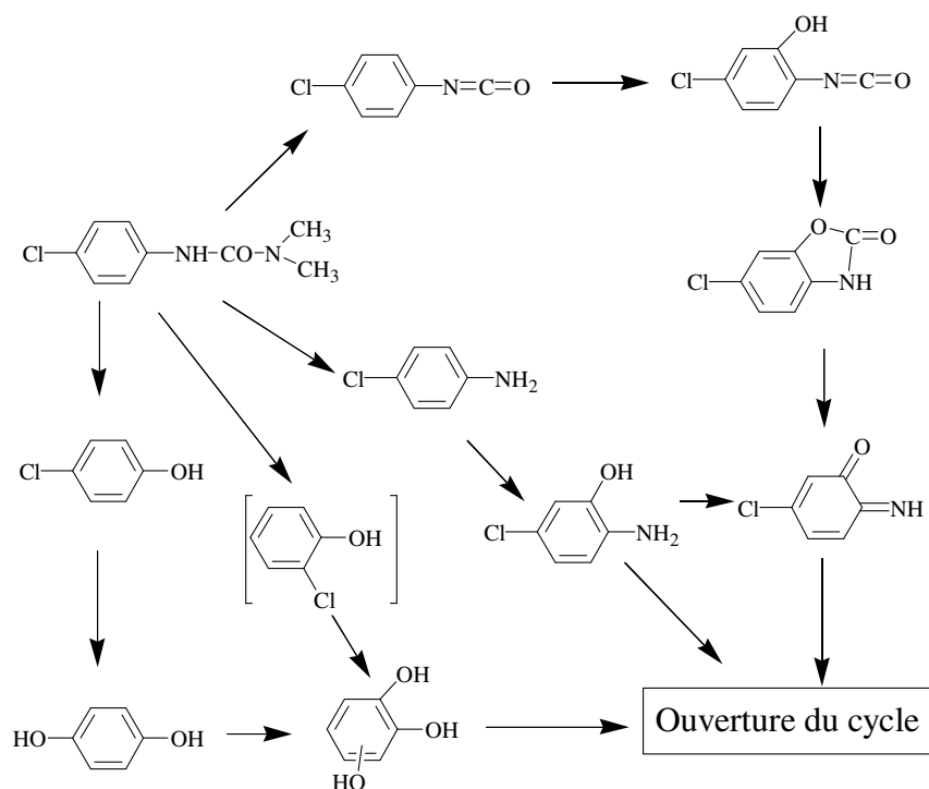
Figure 1.10 : Schéma du mécanisme réactionnel de la dégradation photocatalytique de monuron [134].
